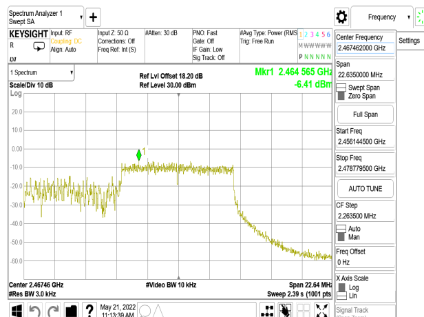
802.11ax_20MHz_Chain1_2462MHz_RU26_8
