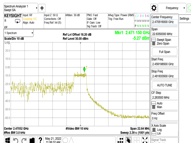
802.11ax_20MHz_Chain1_2462MHz_RU52_40
