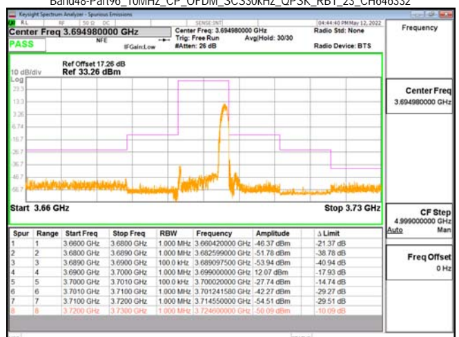
Band48-Part96_10MHz_CP_OFDM_SCS30kHz_QPSK_RB1_23_CH646332
