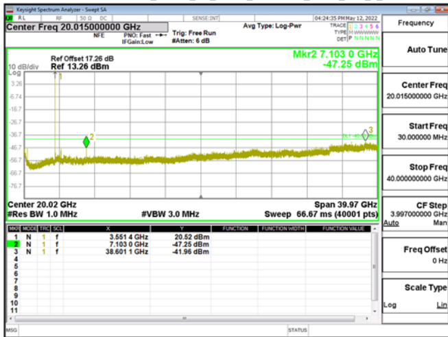
Band48-Part96_10MHz_CP_OFDM_SCS30kHz_QPSK_RB1_1_CH641666
