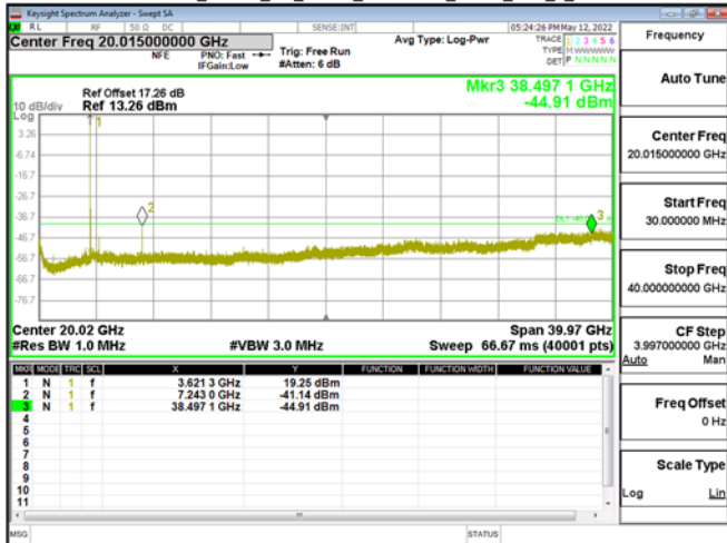
Band48-Part96_10MHz_CP_OFDM_SCS30kHz_QPSK_RB1_1_CH646332
