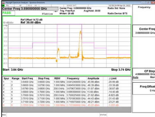
Band48-Part96_20MHz_CP_OFDM_SCS30kHz_QPSK_RB1_50_CH646000
