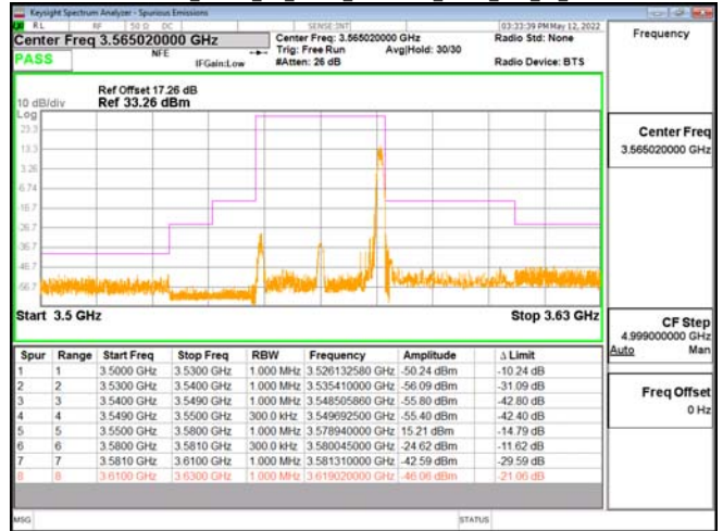
Band48-Part96_30MHz_CP_OFDM_SCS30kHz_QPSK_RB1_77_CH641666
