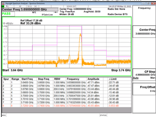
Band48-Part96_20MHz_CP_OFDM_SCS30kHz_QPSK_RB1_50_CH646000
