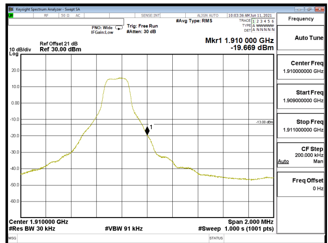
EDGE B2 3M CH19185 QPSK(1,14)
