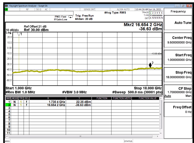
CSE B4 5M CH20175 QPSK(1,0) 1G-18G
