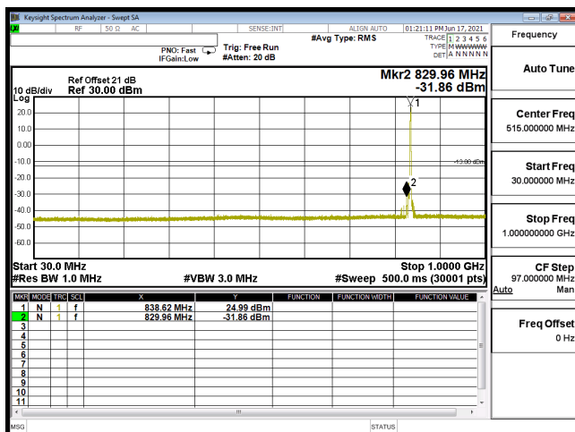
CSE B5 5M CH20525 QPSK(1,24) 30M-1G
