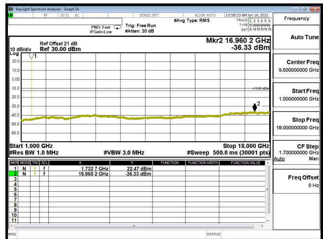
CSE B4 10M CH20350 QPSK(1,25) 1G-18G
