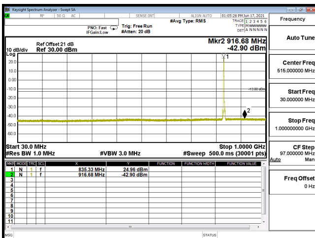
CSE B5 3M CH20525 QPSK(1,0) 30M-1G
