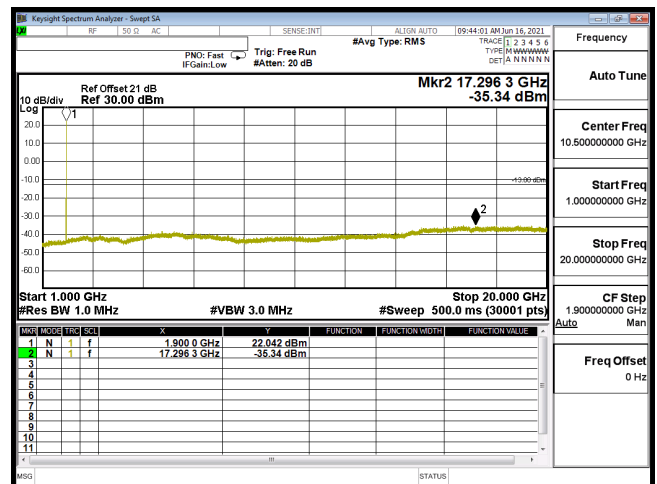
CSE B2 20M CH19100 QPSK(1,50) 1G-20G
