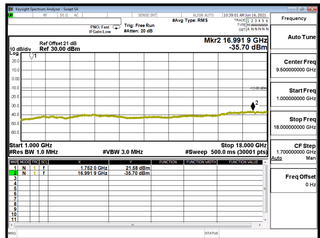
CSE B4 3M CH20385 QPSK(1,0) 1G-18G
