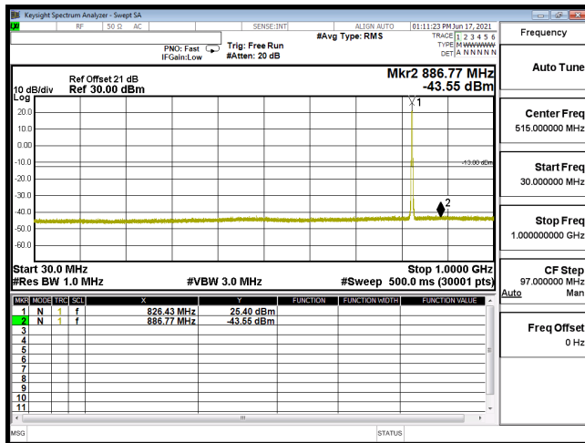
CSE B5 5M CH20425 QPSK(1,12) 30M-1G
