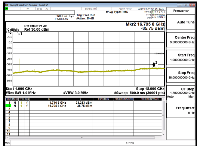
CSE B4 10M CH20000 QPSK(1,0) 1G-18G
