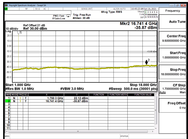
CSE B4 5M CH20375 QPSK(1,0) 1G-18G
