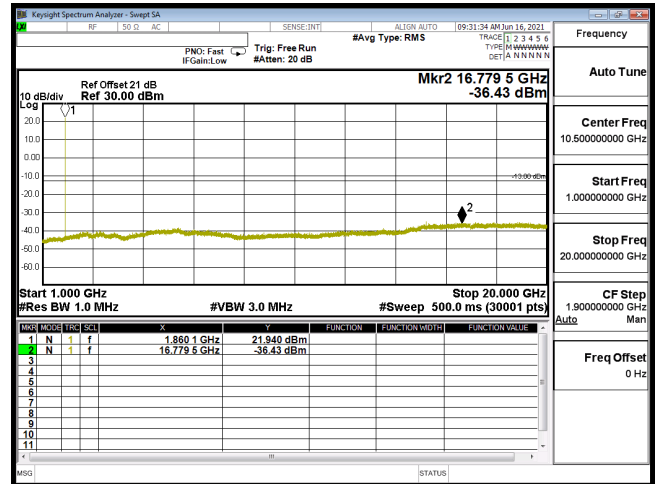
CSE B2 20M CH18700 QPSK(1,50) 1G-20G
