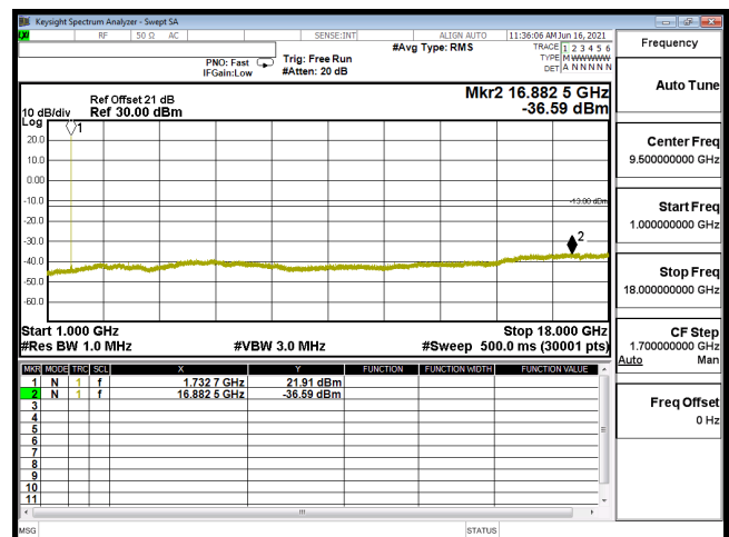
CSE B4 20M CH20175 QPSK(1,50) 1G-18G
