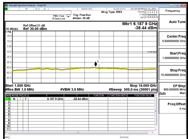
CSE B5 1.4M CH20525 QPSK(3,0) 1G-10G
