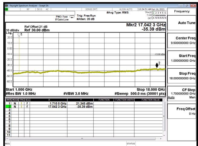
CSE B4 3M CH19965 QPSK(1,0) 1G-18G
