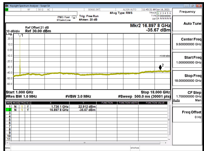
CSE B4 20M CH20300 QPSK(1,0) 1G-18G
