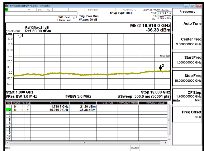
CSE B4 20M CH20050 16QAM(1,50) 1G-18G
