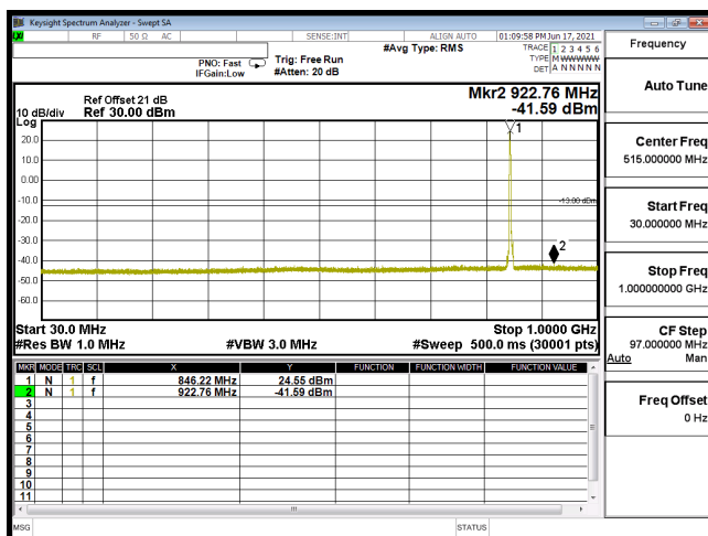
CSE B5 3M CH20635 QPSK(1,0) 30M-1G
