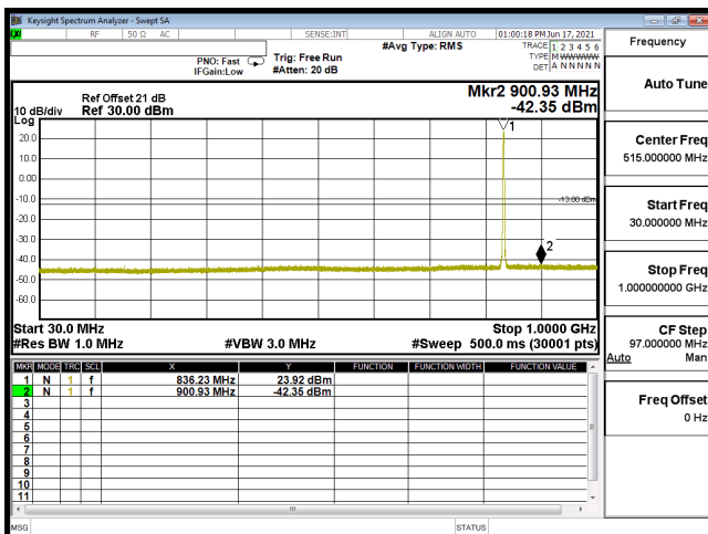
CSE B5 1.4M CH20525 QPSK(3,0) 30M-1G
