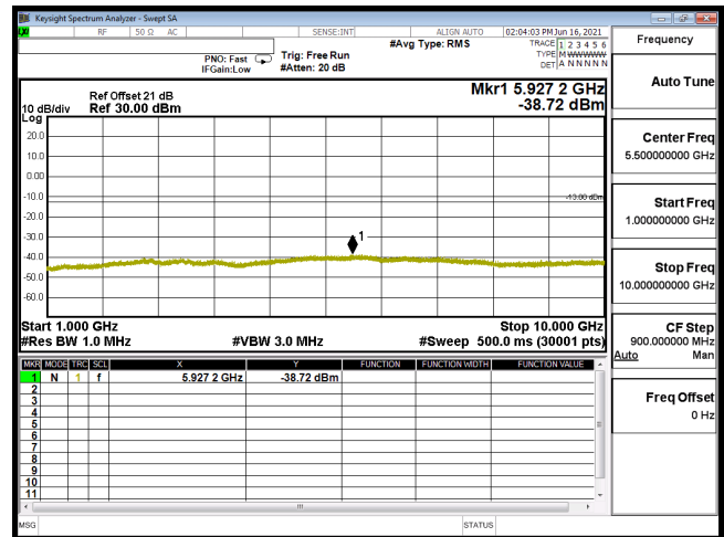
CSE B5 5M CH20425 QPSK(1,12) 1G-10G
