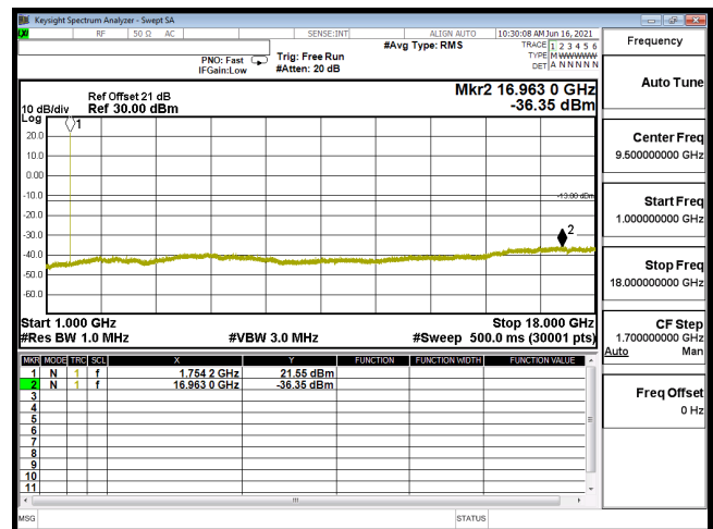
CSE B4 1.4M CH20393 QPSK(1,2) 1G-18G
