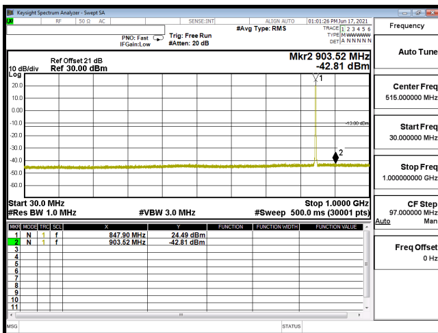
CSE B5 1.4M CH20643 QPSK(1,0) 30M-1G
