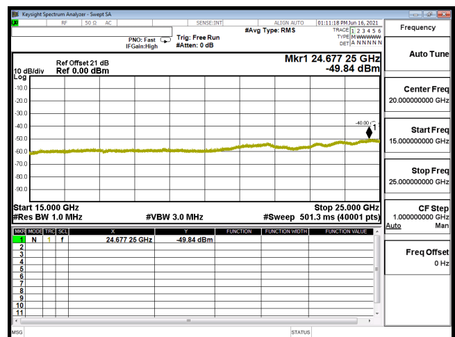
CSE B30 5M CH27685 16QAM(1,0) 15G-25G
