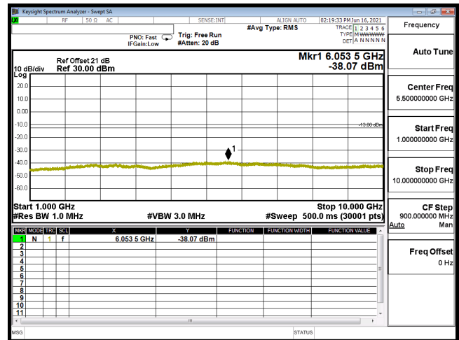
CSE B5 10M CH20450 QPSK(1,49) 1G-10G
