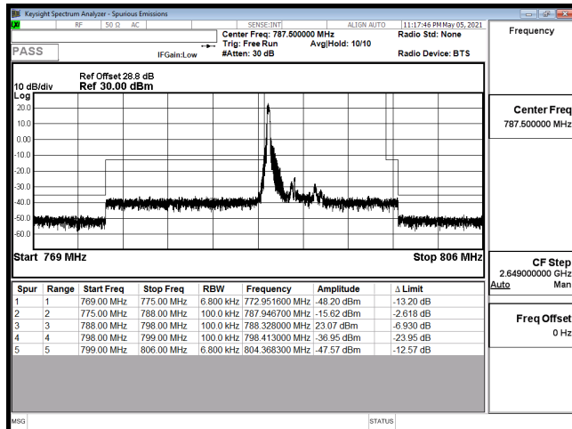
EDGE-B14 5M-CH23305-QPSK(1,0)
