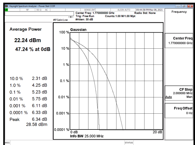
PTAR-B66_20M-CH132572-QPSK
