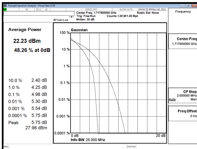
PTAR-B66_15M-CH132047-QPSK
