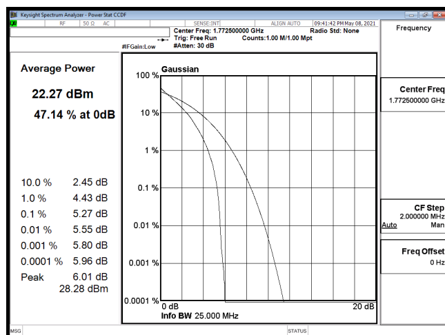
PTAR-B66_15M-CH132597-QPSK
