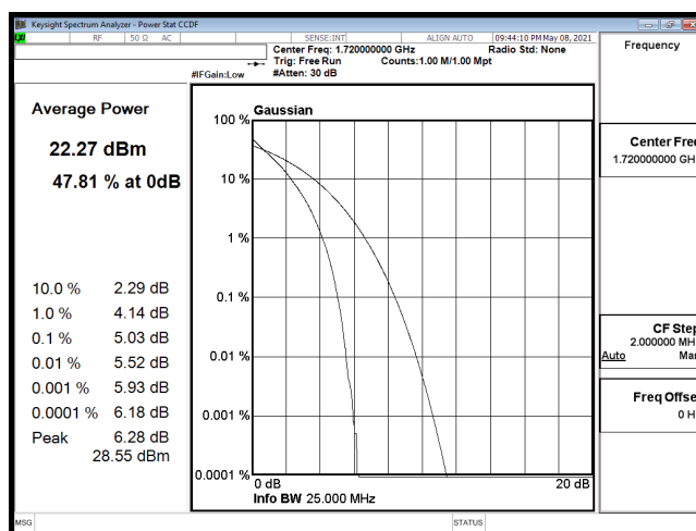
PTAR-B66_20M-CH132072-QPSK
