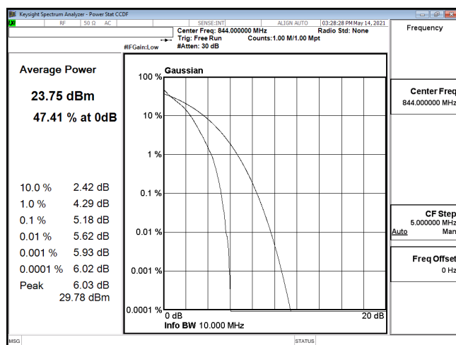
PTAR-ENDC_30A_n5-QPSK_10M_CH168800_844(50,0)
