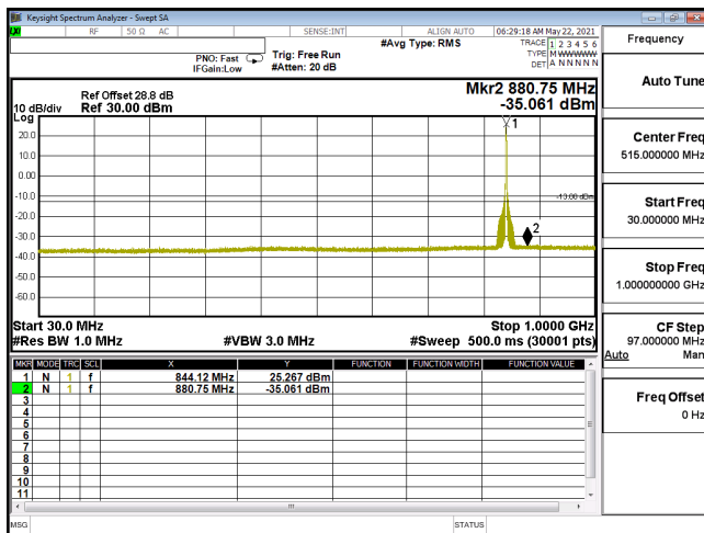
CSE-ENDC_30A_n5-PI2-BPSK_10M_CH168800_844(1,26)-30M-1G
