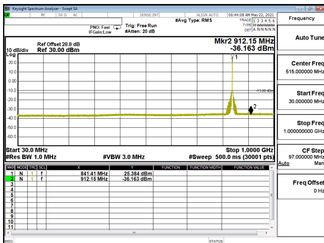
CSE-ENDC_30A_n5-QPSK_15M_CH168300_841.5(1,39)-30M-1G
