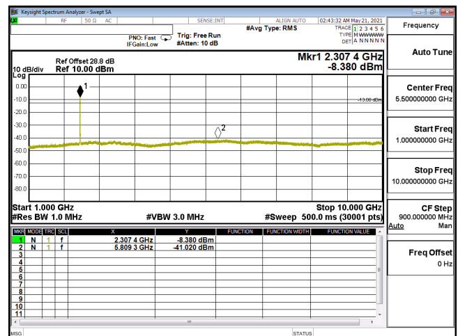
CSE-ENDC_30A_n5-QPSK_10M_CH168800_844(1,26)-1G-10G
