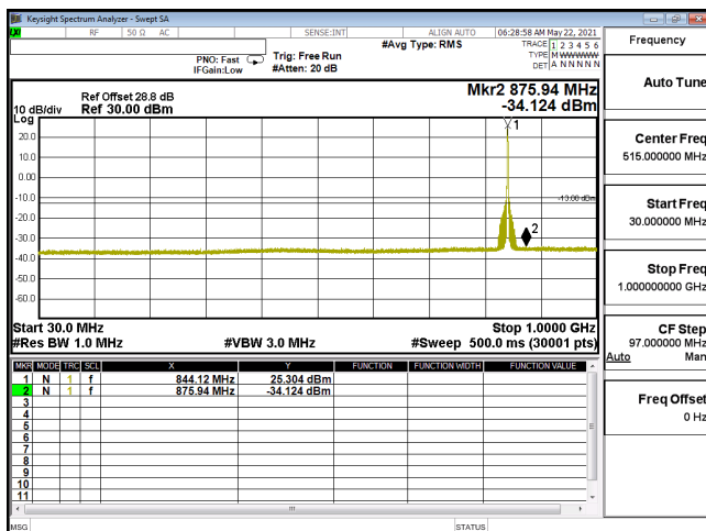
CSE-ENDC_30A_n5-QPSK_10M_CH168800_844(1,26)-30M-1G
