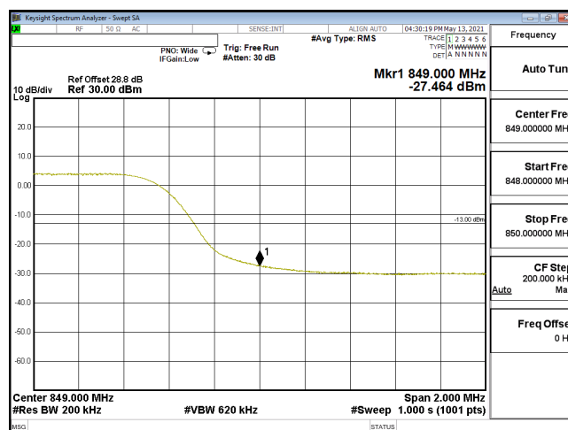
EDGE-ENDC 30A n5-QPSK 20M CH167800 839(100,6) SCS15KHz
