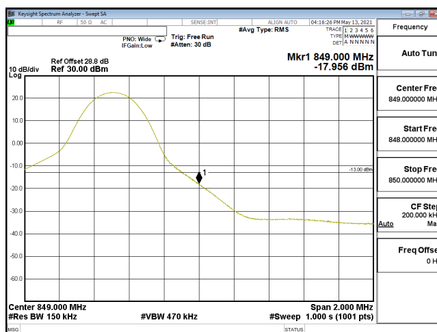
EDGE-ENDC_30A_n5-QPSK_15M_CH168300_841.5(1,78)_SCS15KHz
