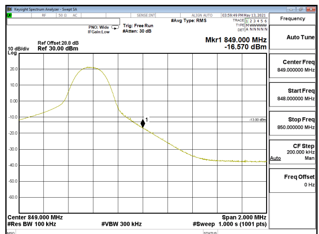
EDGE-ENDC 30A n5-QPSK 10M CH168800 844(1,51) SCS15KHz
