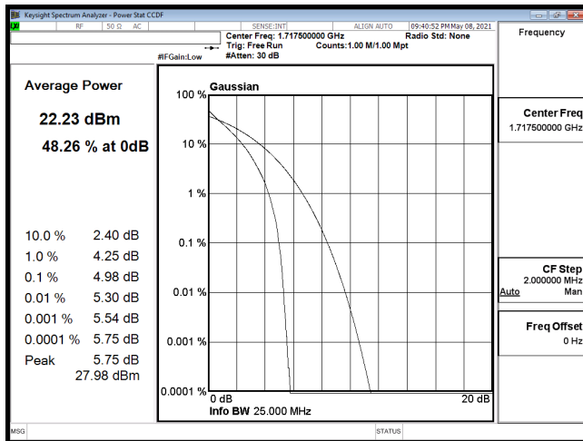
PTAR-B66_15M-CH132047-QPSK
