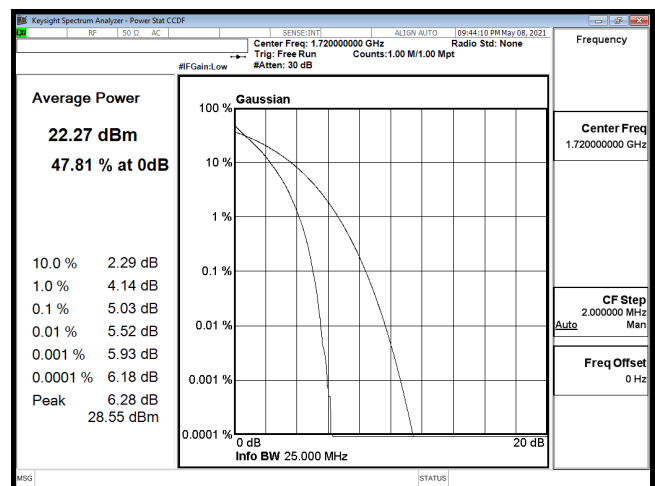
PTAR-B66_20M-CH132072-QPSK
