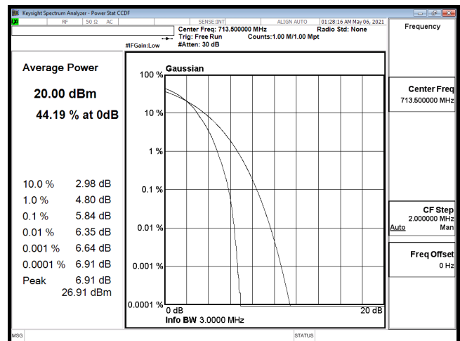
PTAR-B12_5M-CH23155-16QAM
