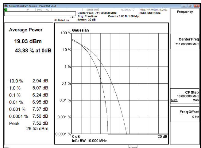
PTAR-B12_10M-CH23130-64QAM
