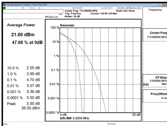
PTAR-B12_5M-CH23155-QPSK
