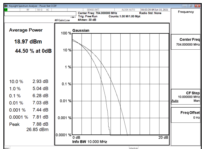
PTAR-B12_10M-CH23060-64QAM
