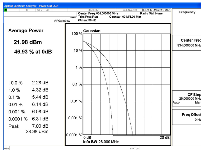
PTAR(10M+10M)-2ULCA_5B-QPSK_829(50,0)+838.9(50,0)
