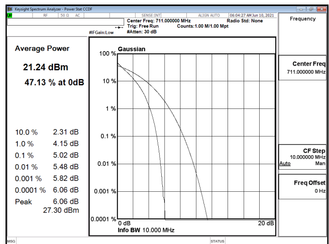
PTAR-B12_10M-CH23130-QPSK
