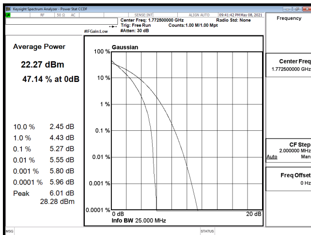
PTAR-B66_15M-CH132597-QPSK
