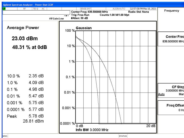
PTAR-B5_3M-CH20525-QPSK
