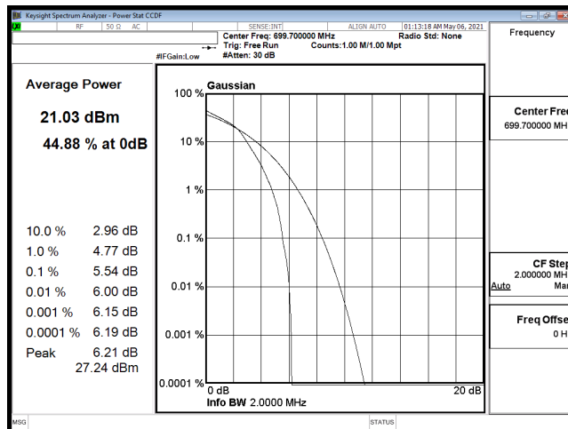
PTAR-B12_1.4M-CH23017-16QAM
