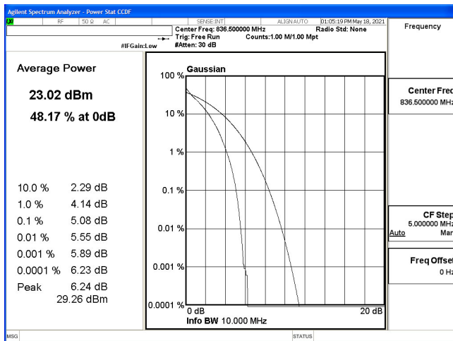
PTAR-B5_10M-CH20525-QPSK
