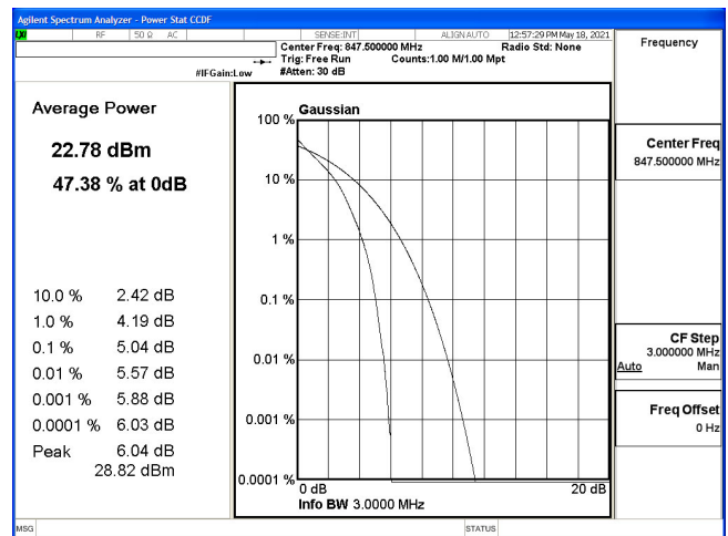
PTAR-B5_3M-CH20635-QPSK
