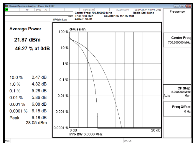
PTAR-B12_3M-CH23025-QPSK
