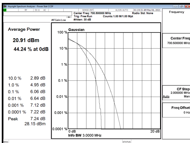
PTAR-B12_3M-CH23025-16QAM
