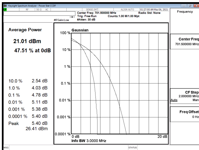
PTAR-B12_5M-CH23035-QPSK
