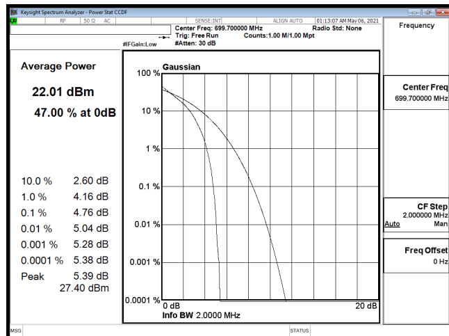
PTAR-B12_1.4M-CH23017-QPSK
