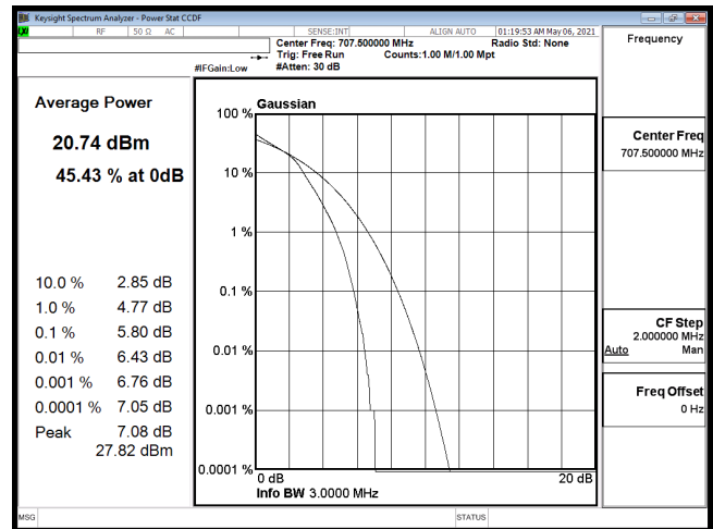
PTAR-B12_3M-CH23095-16QAM
