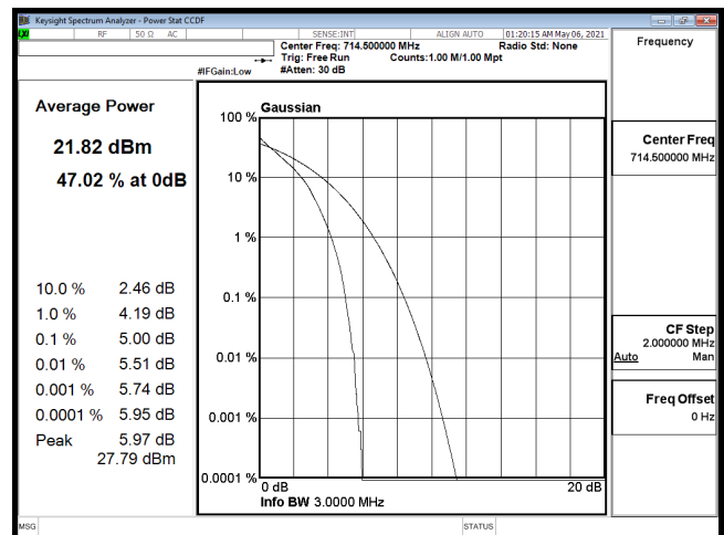
PTAR-B12_3M-CH23165-16QAM
