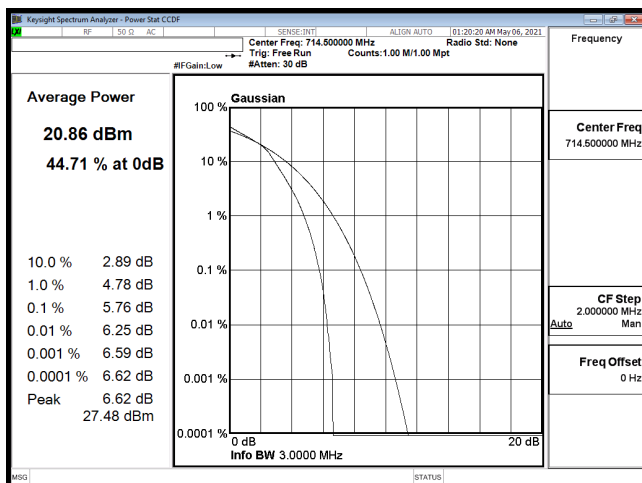
PTAR-B12_3M-CH23165-64QAM
