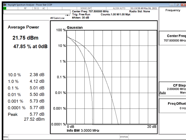
PTAR-B12_3M-CH23095-QPSK
