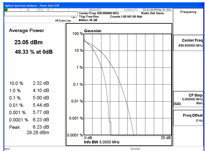
PTAR-B5_5M-CH20525-QPSK
