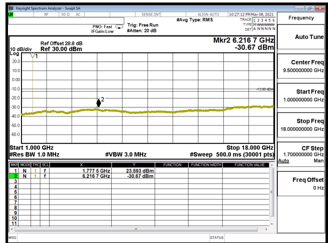
CSE-B66_5M-CH132647-QPSK(1,12)-1G-18G
