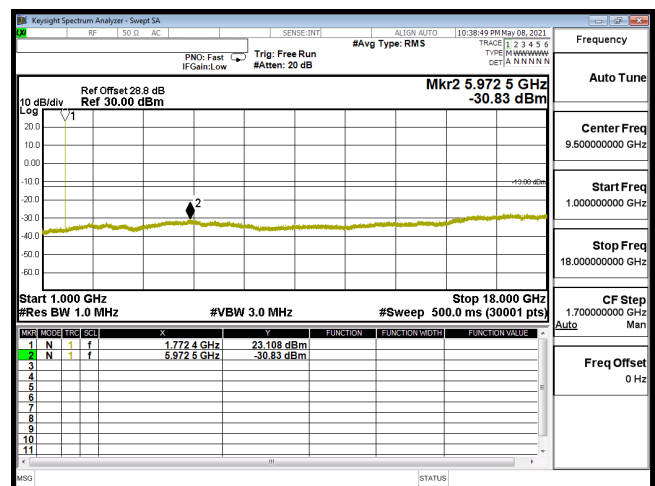
CSE-B66_15M-CH132597-16QAM(1,37)-1G-18G
