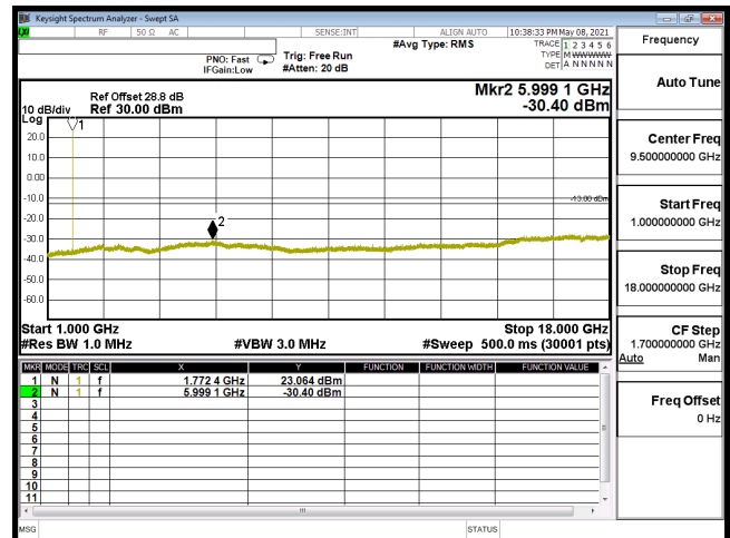
CSE-B66_15M-CH132597-QPSK(1,37)-1G-18G
