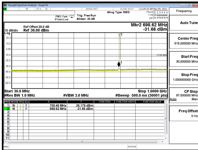
CSE-B12_3M-CH23025-QPSK(1,7)-30M-1G
