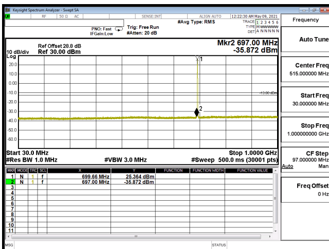
CSE-B12_1.4M-CH23017-16QAM(1,2)-30M-1G
