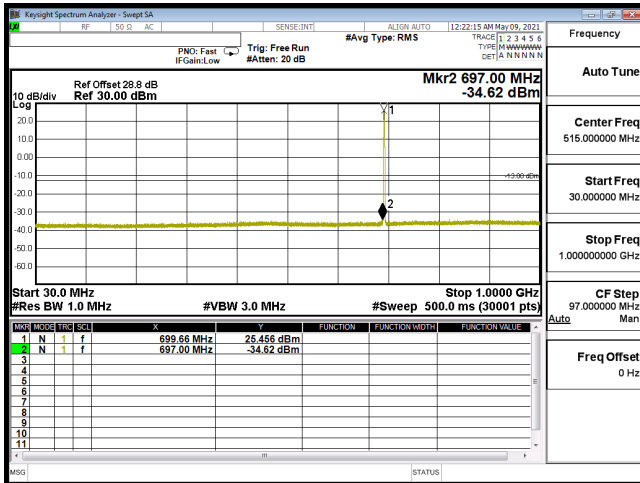
CSE-B12_1.4M-CH23017-QPSK(1,2)-30M-1G
