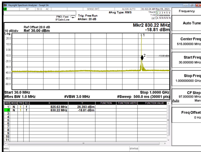
CSE-B5_3M-CH20415-QPSK(1,7)-30M-1G
