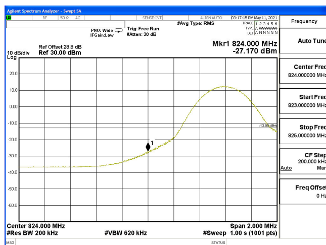
EDGE(10M+10M)-2ULCA_5B-16QAM_829(1,0)+838.9(1,49)
