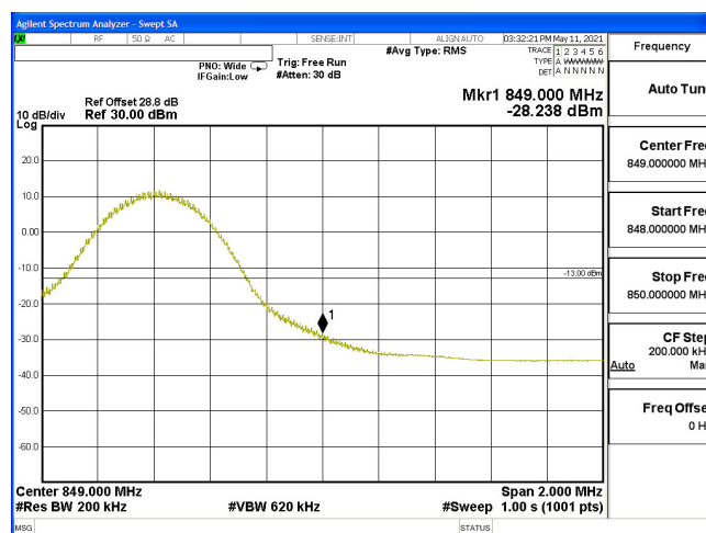
EDGE(10M+10M)-2ULCA_5B-QPSK_834.1(1,0)+844(1,49)
