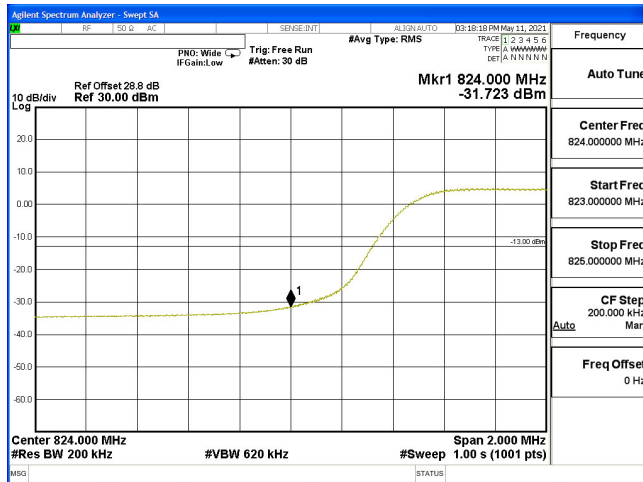
EDGE(10M+10M)-2ULCA_5B-QPSK_829(50,0)+838.9(50,0)
