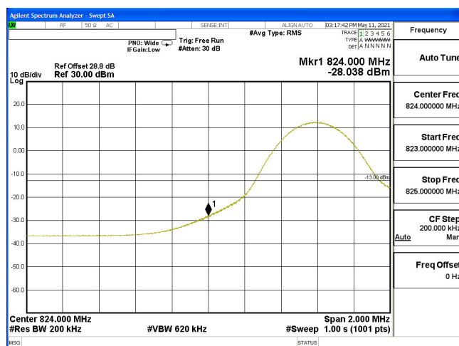
EDGE(10M+10M)-2ULCA_5B-QPSK_829(1,0)+838.9(1,49)
