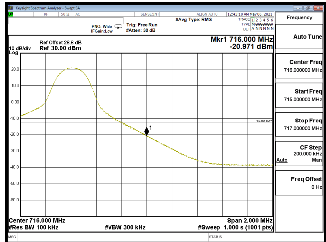
EDGE-B12_10M-CH23130-QPSK(1,49)
