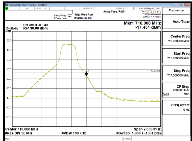
EDGE-B12_3M-CH23165-QPSK(1,14)
