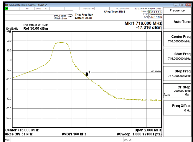
EDGE-B12_5M-CH23155-QPSK(1,24)
