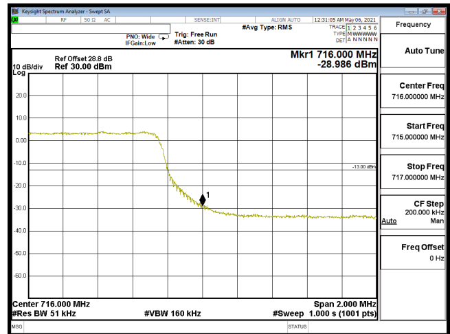
EDGE-B12_5M-CH23155-QPSK(25,0)
