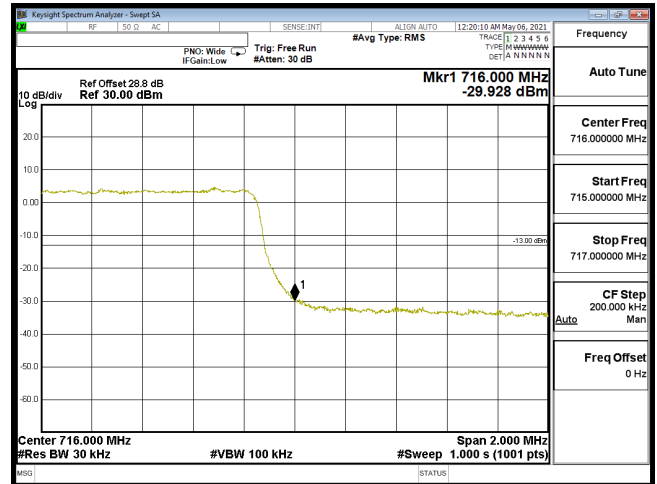
EDGE-B12_3M-CH23165-QPSK(15,0)
