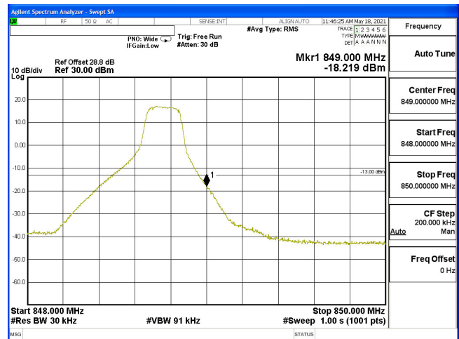
EDGE-B5_3M-CH20635-QPSK(1,14)
