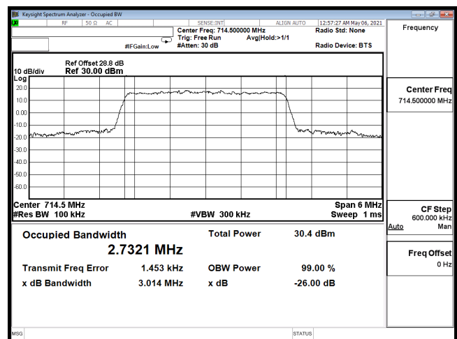
OCC-B12_3M-CH23165-QPSK
