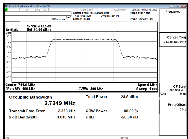
OCC-B12_3M-CH23165-64QAM
