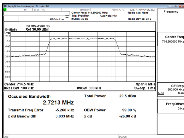
OCC-B12_3M-CH23165-16QAM
