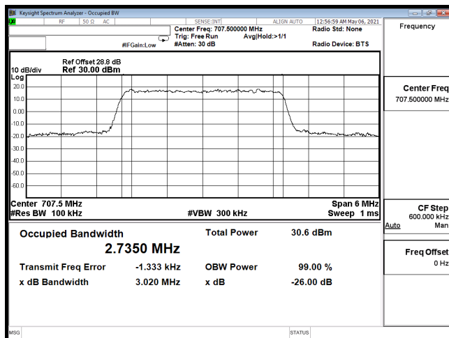
OCC-B12_3M-CH23095-QPSK
