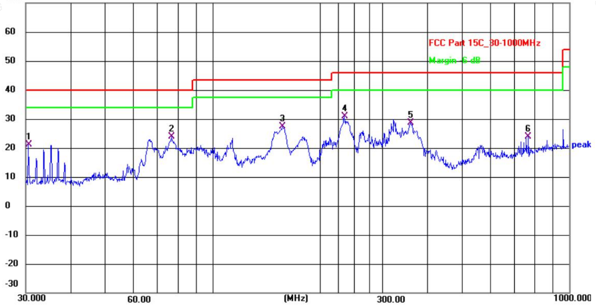
Horizontal 70.0 dBuV/m
