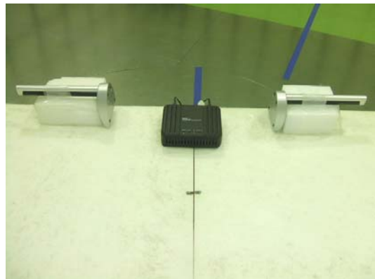
Ant - Z-axis
