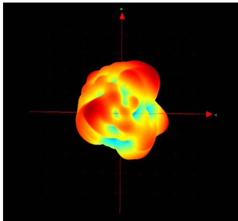
ANT5_2.4G(Frequency=2450MHz)
