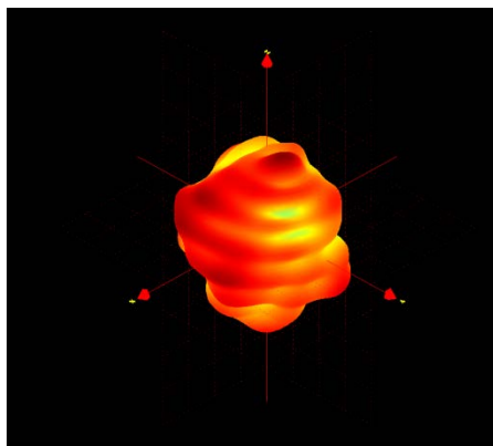
ANT5_6E(Frequency=6000MHz)
