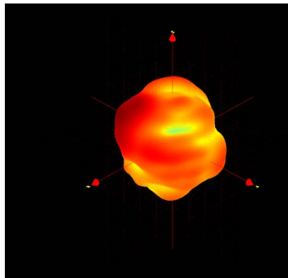
ANT5_5G(Frequency=5800MHz)
