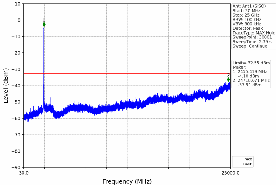
802.11n(HT40)_HCH_2452MHz_Ant1 (SISO)_NTNV
