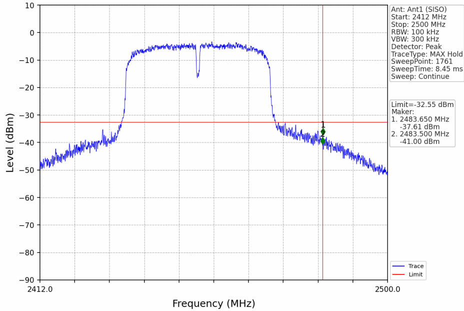
802.11n(HT40)_HCH_2452MHz_Ant1 (SISO)_NTNV
