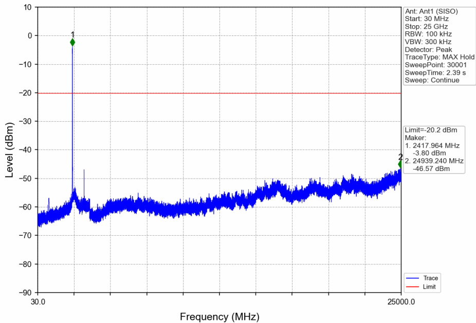
802.11n(HT20)_LCH_2412MHz_Ant1 (SISO)_NTNV
