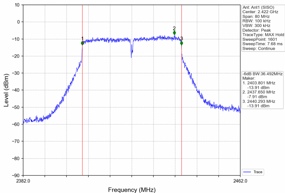
802.11n(HT40)_LCH_2422MHz_Ant1 (SISO)_NTNV
