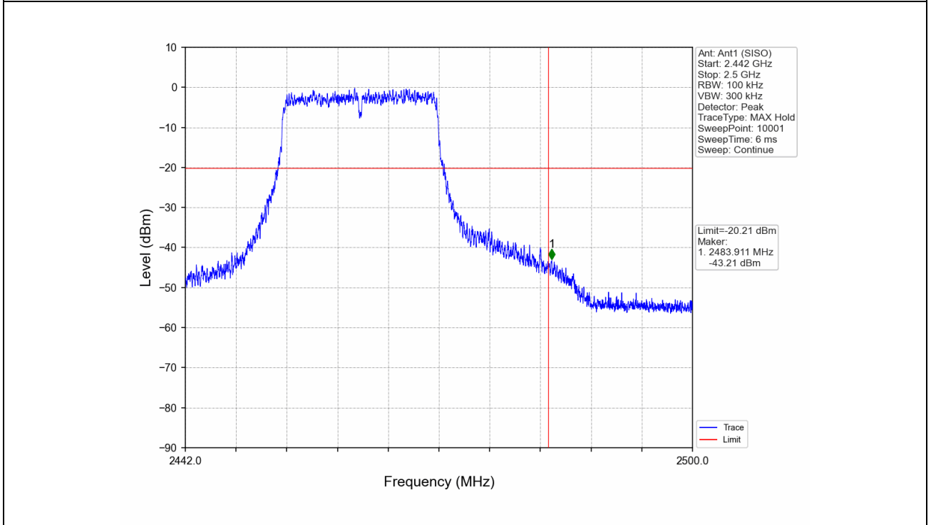
802.11n(HT20)_HCH_2462MHz_Ant1 (SISO)_NTNV
