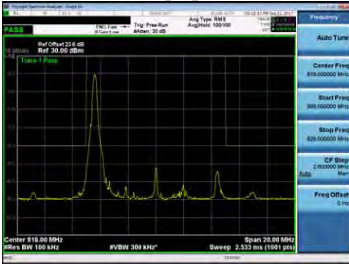
Band 26_10M_RB1,49
