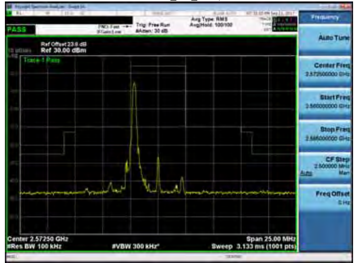
Band 38_5M_RB1,24
