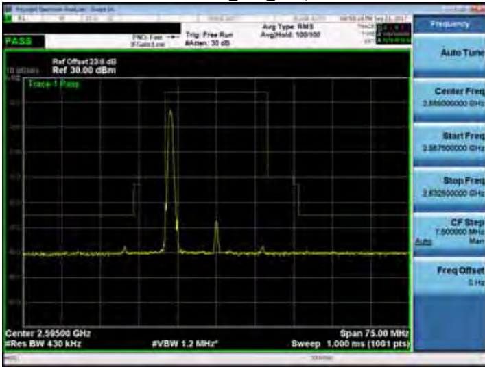
Band 38_20M_RB1,99
