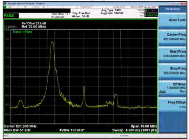
Band 26_5M_RB1,24
