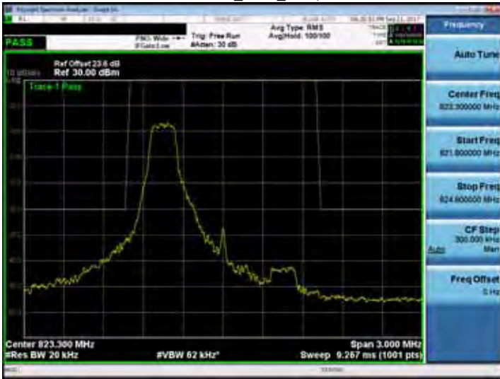
Band 26_1.4M_RB1,5
