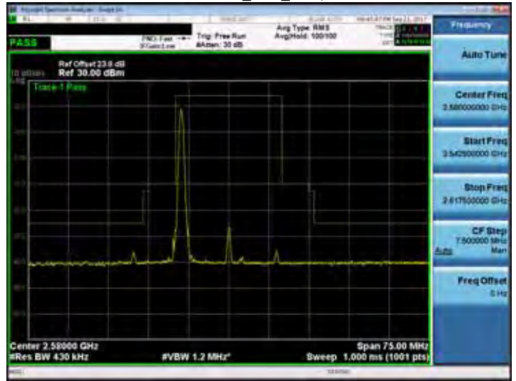
Band 38_20M_RB1,99
