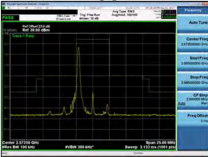
Band 38_5M_RB1,24
