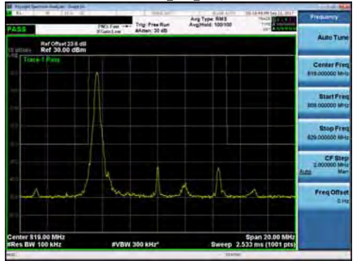
Band 26_10M_RB1,49
