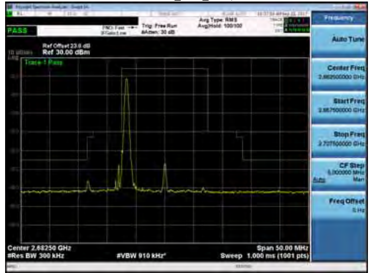
Band 41_15M_RB1,74
