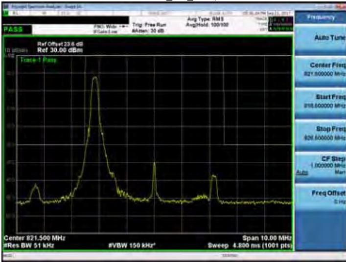
Band 26_5M_RB1,24
