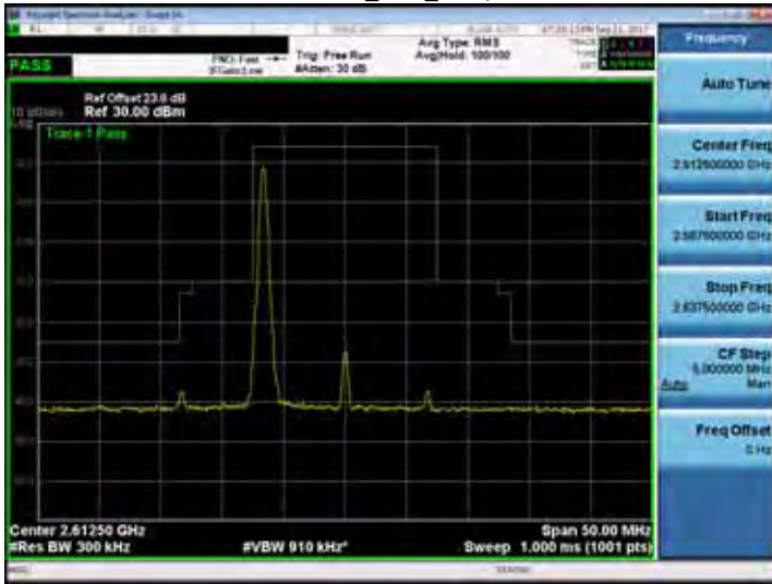
Band 38_15M_RB1,74
