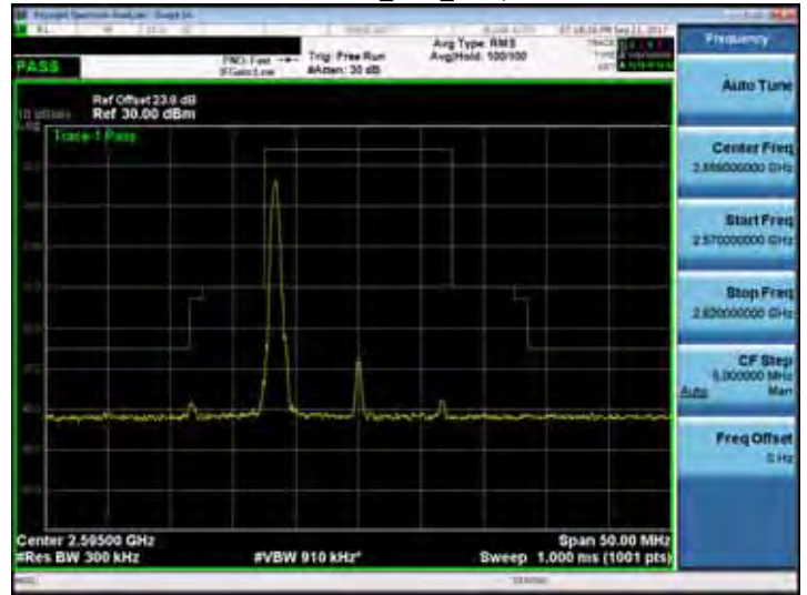
Band 38_15M_RB1,74
