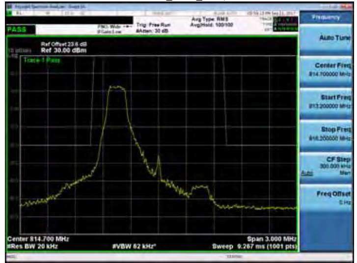
Band 26_1.4M_RB1,5
