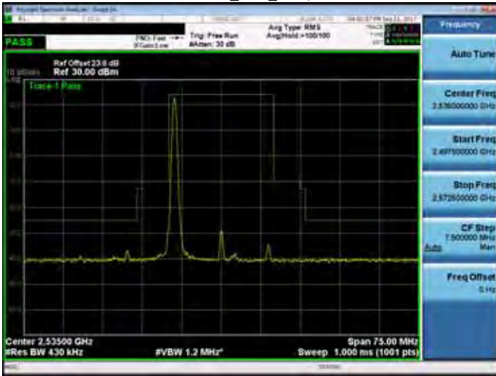
Band 7_20M_RB1,99
