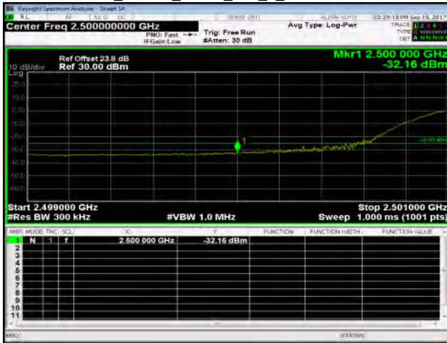
Band7_20MHz_QPSK_100_0_LowCH20850-2510
