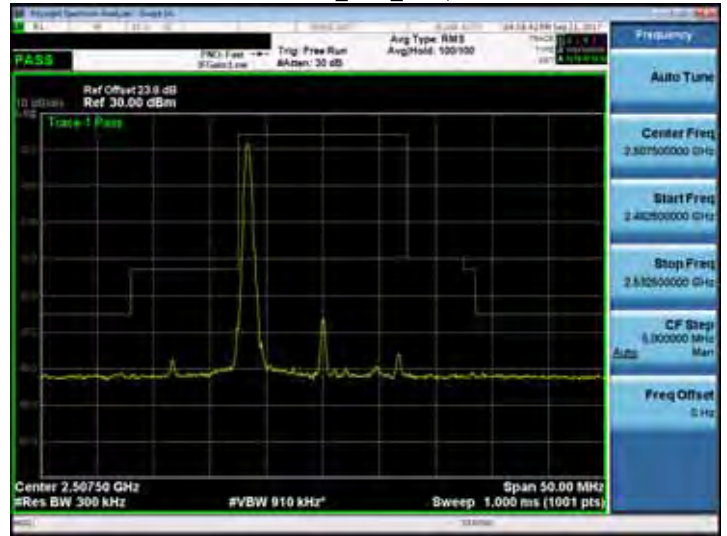
Band 7_15M_RB1,74
