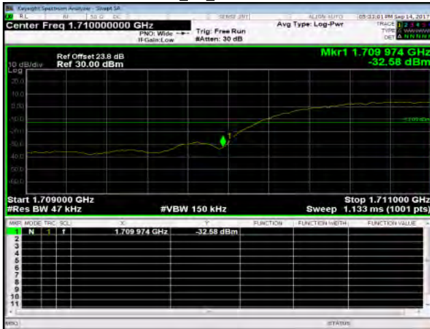
WCDMA_B4_LowCH1312-1712.4
