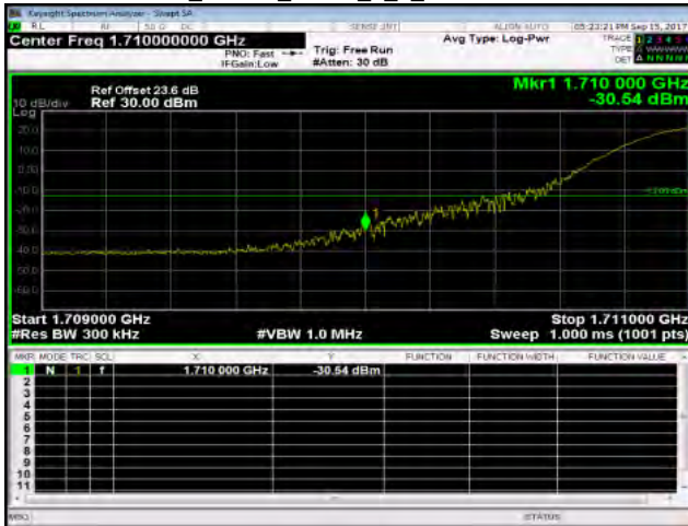
Band4_20MHz_QPSK_1_0_LowCH20050-1720
