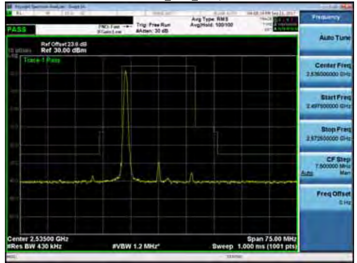
Band 7_20M_RB1,99
