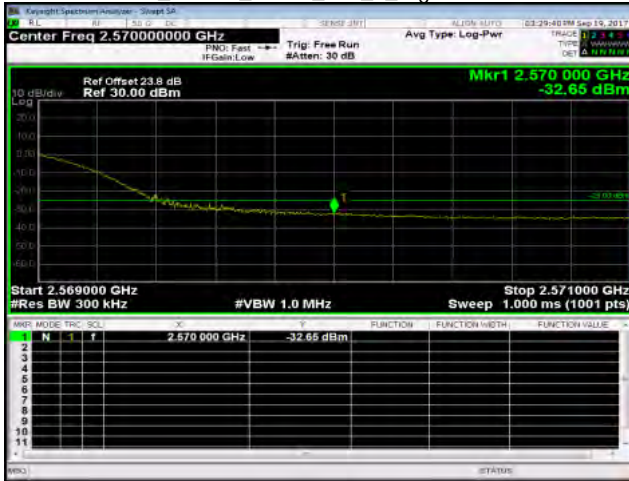
Band7_20MHz_QPSK_100_0_HighCH21350-2560
