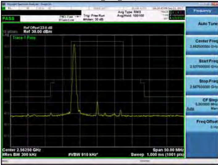
Band 7_15M_RB1,74
