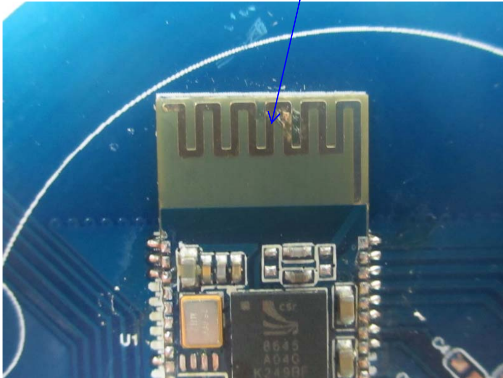
The BT module antenna
