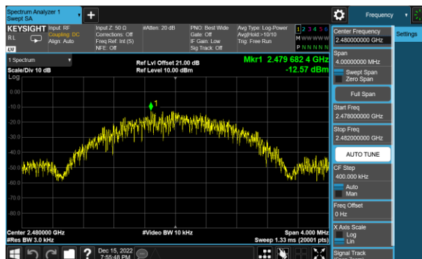
CH78 (2480MHz)
