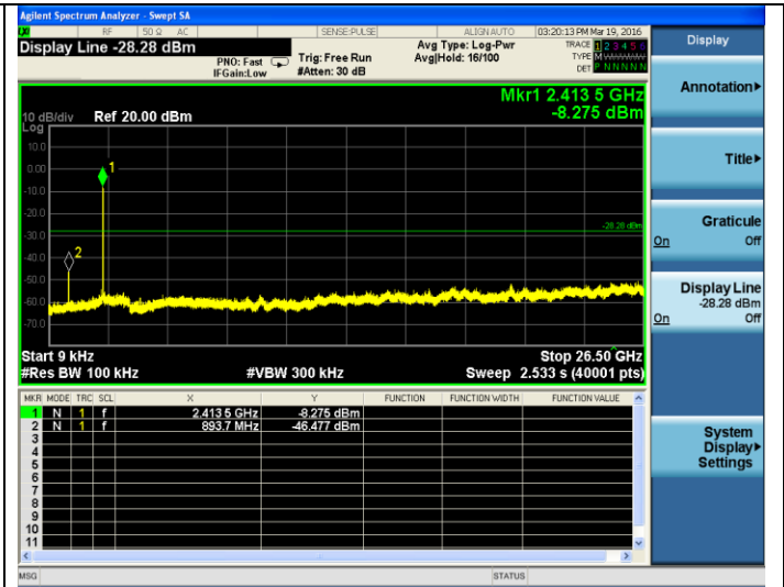
802.11g-2412MHz
