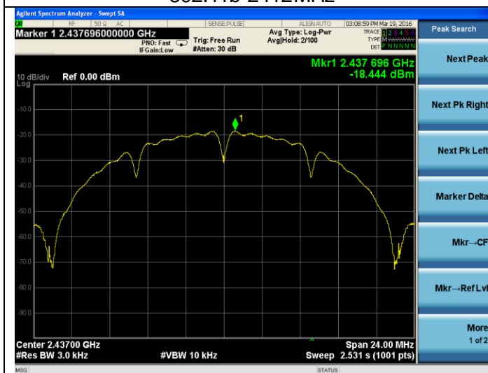
802.11b-2437MHz
