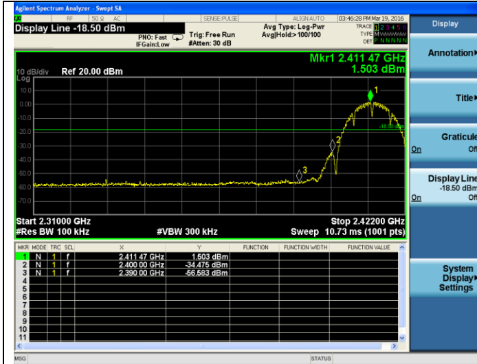
802.11b-2412MHz
