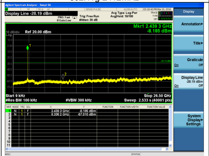
802.11g-2437MHz
