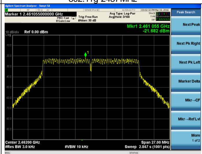
802.11g-2462MHz
