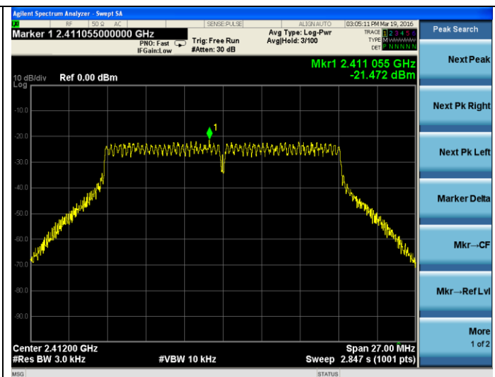
802.11g-2412MHz
