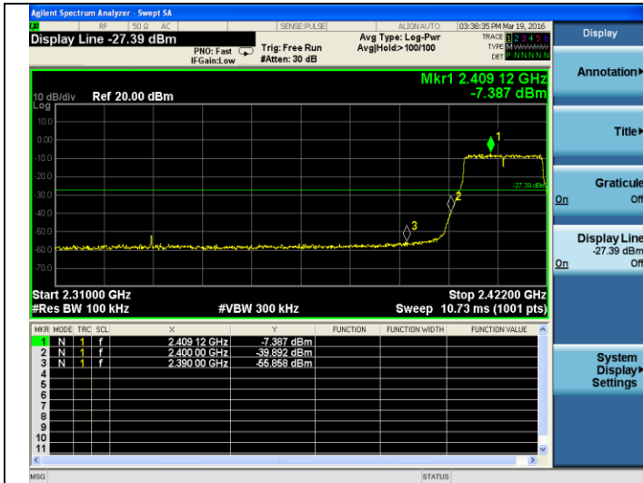
802.11n(HT20)-2412MHz
