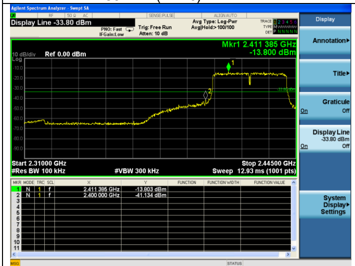
802.11n(HT40)-2422MHz
