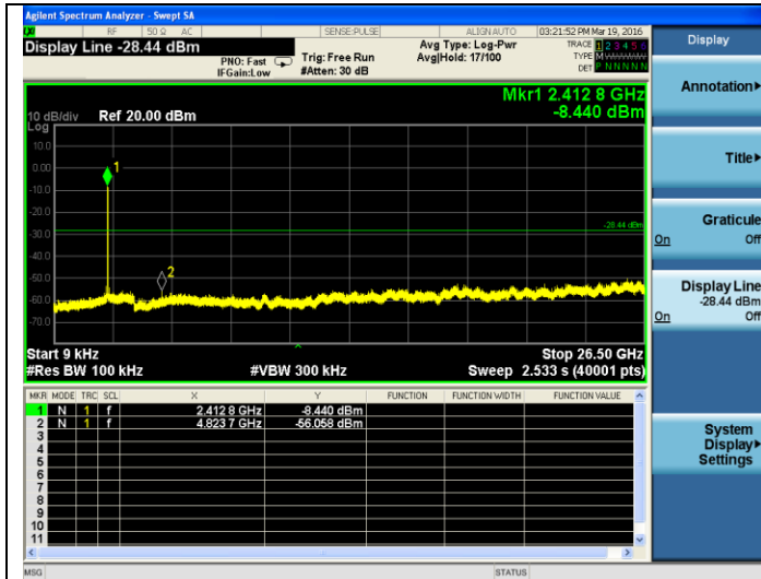
802.11n(HT20)-2412MHz
