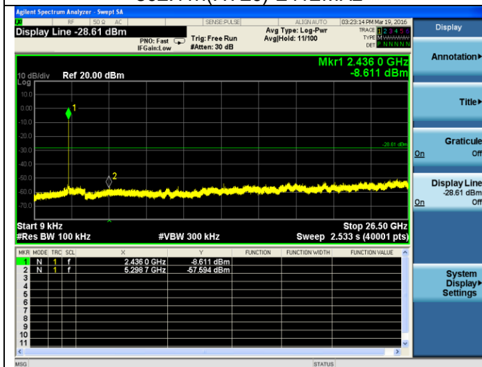
802.11n(HT20)-2437MHz
