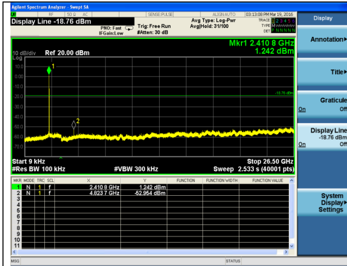
802.11b-2412MHz
