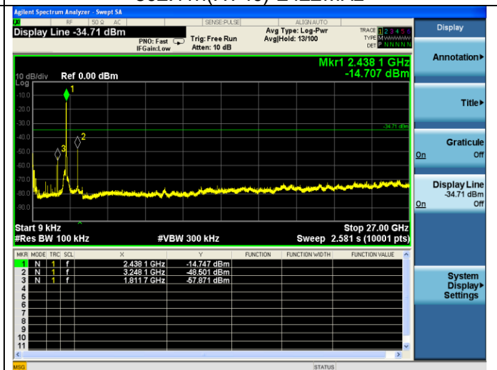
802.11n(HT40)-2437MHz
