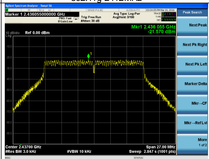
802.11g-2437MHz
