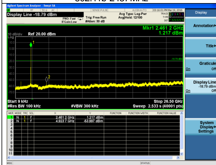
802.11b-2462MHz
