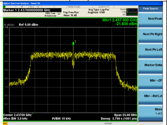
802.11n(HT40)-2437MHz
