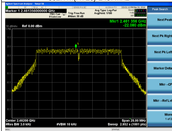
802.11n(HT20)-2462MHz
