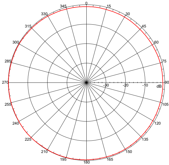
5.15 GHz H-Plane
