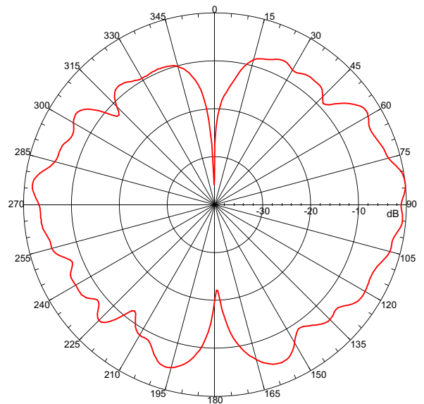
5.875 GHz E-Plane
