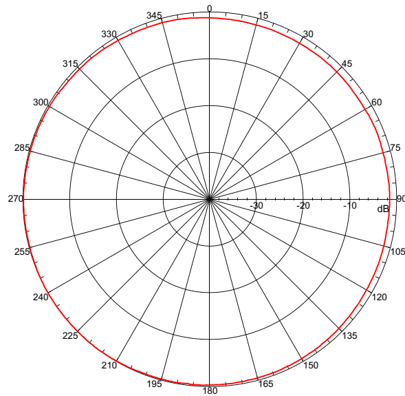
5.50 GHz H-Plane
