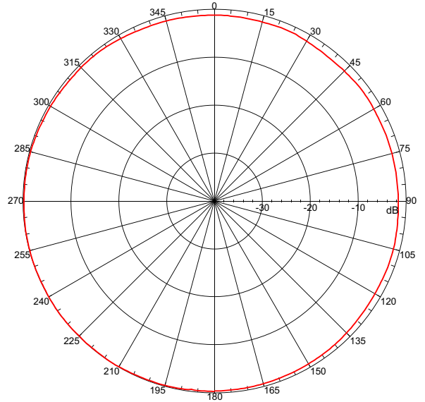
5.35 GHz H-Plane
