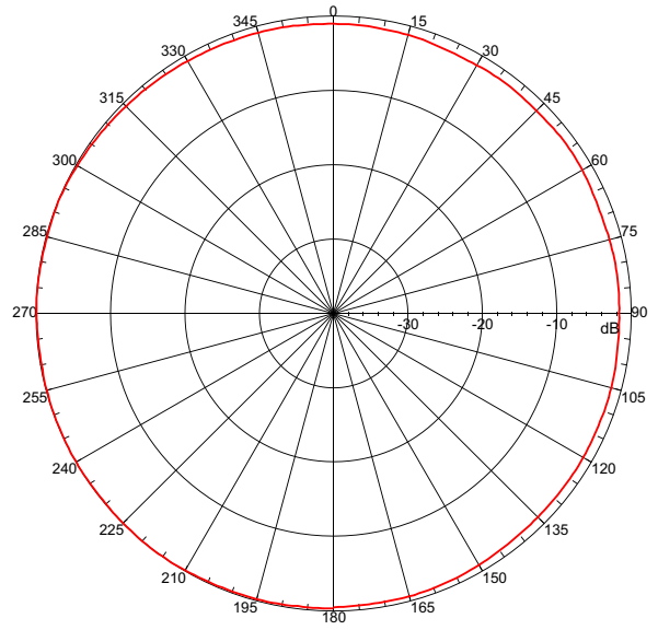
5.875 GHz H-Plane
