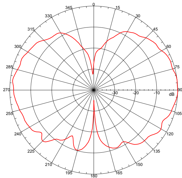
5.50 GHz E-Plane
