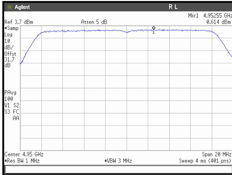
PPSD Low Ch 4950MHz
