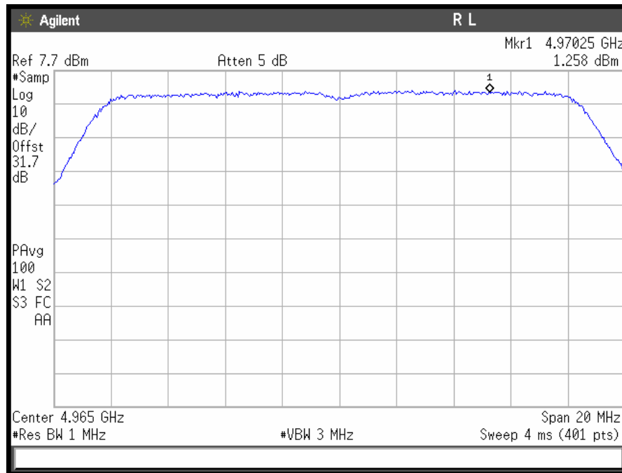
PPSD Mid Ch 4965MHz
