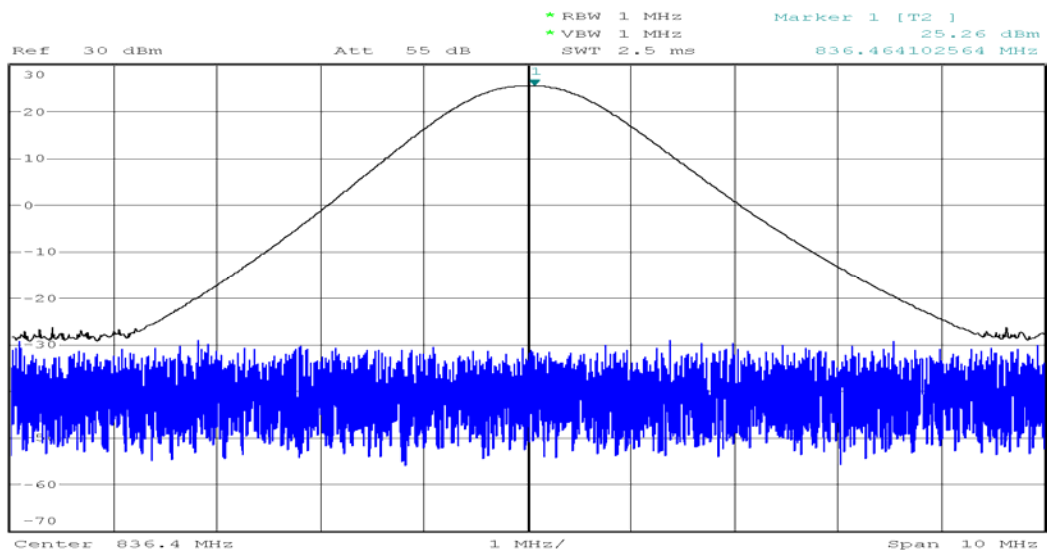
GSM 850 CH 189
