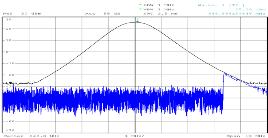
GSM 850 CH 251
