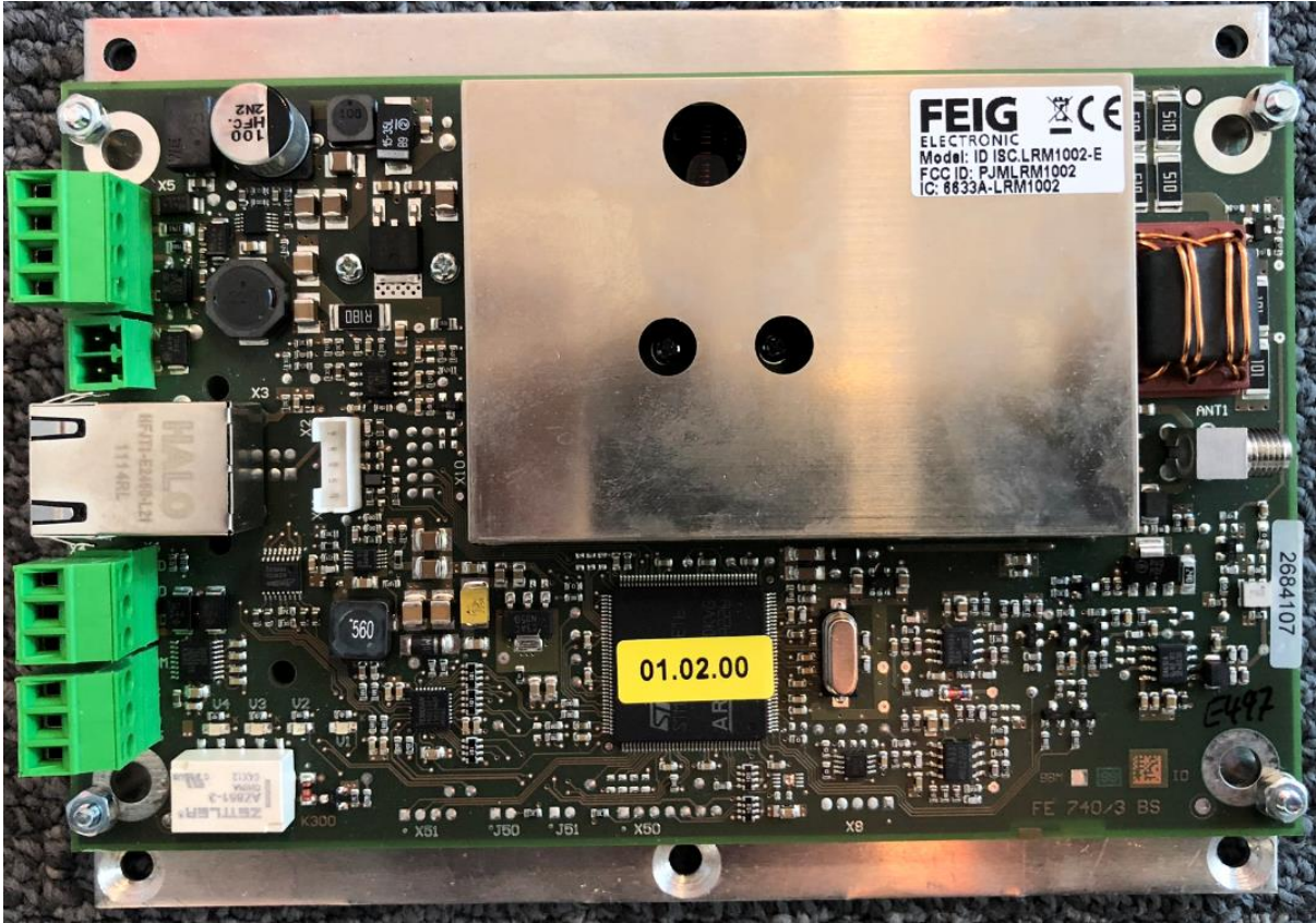
FEIG Model ID ISC.LRM1002-E – Front
