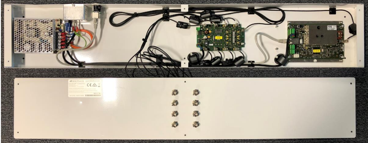
FEIG Model ID ISC.LRM1002-E – Front
