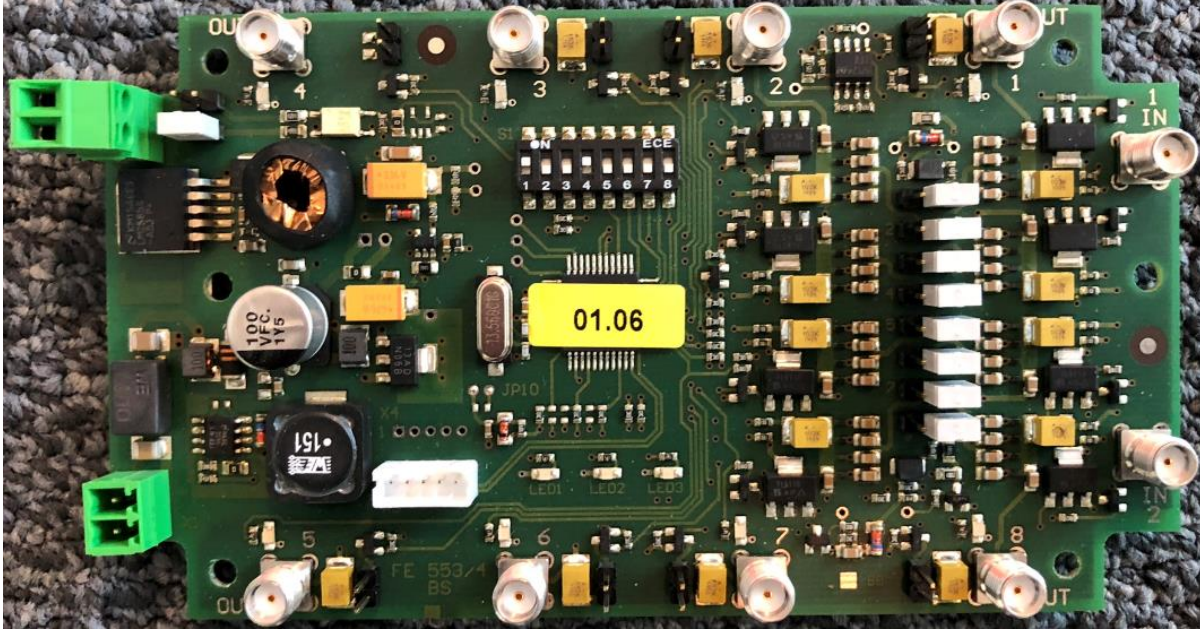
FEIG Model ID ISC.ANT.MUX.M8 - Front
