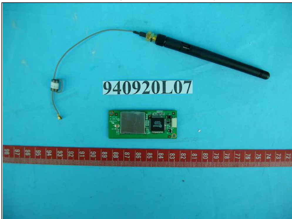
Antenna 4 (Model no: C678-510005-A)
