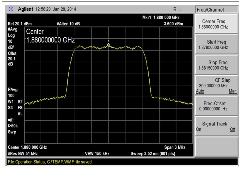
CDMA_UL 1850-1910_Output
