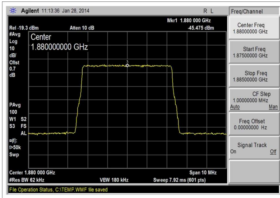
LTE_UL 1850-1910_Input
