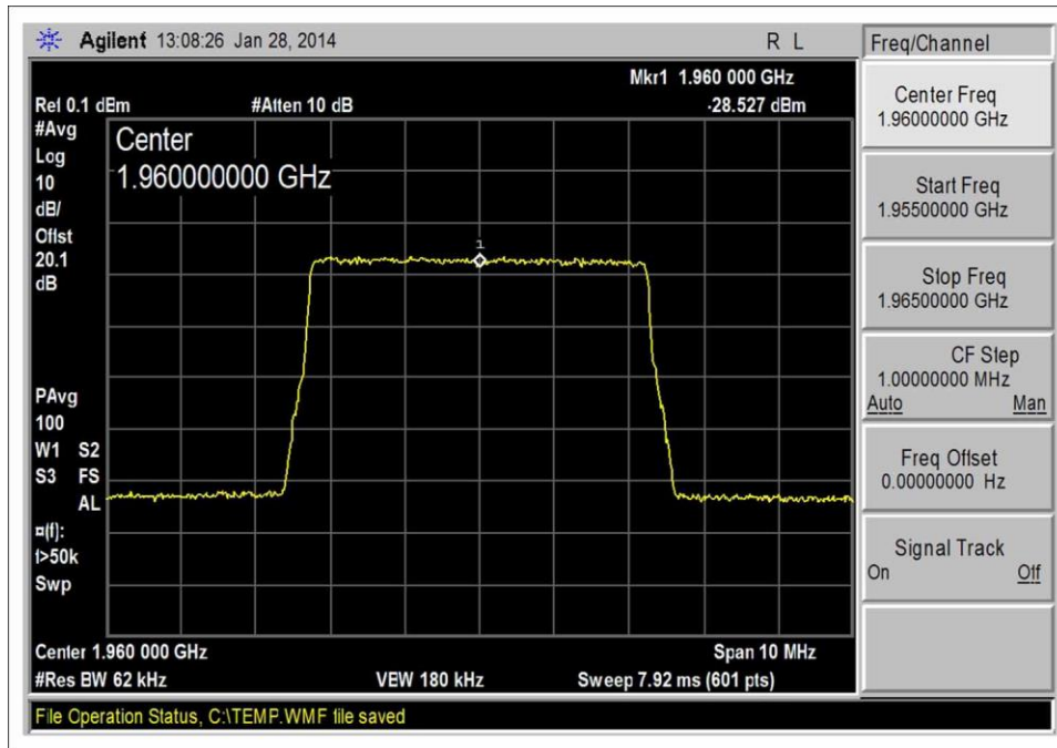
LTE_DL 1930-1990_Output
