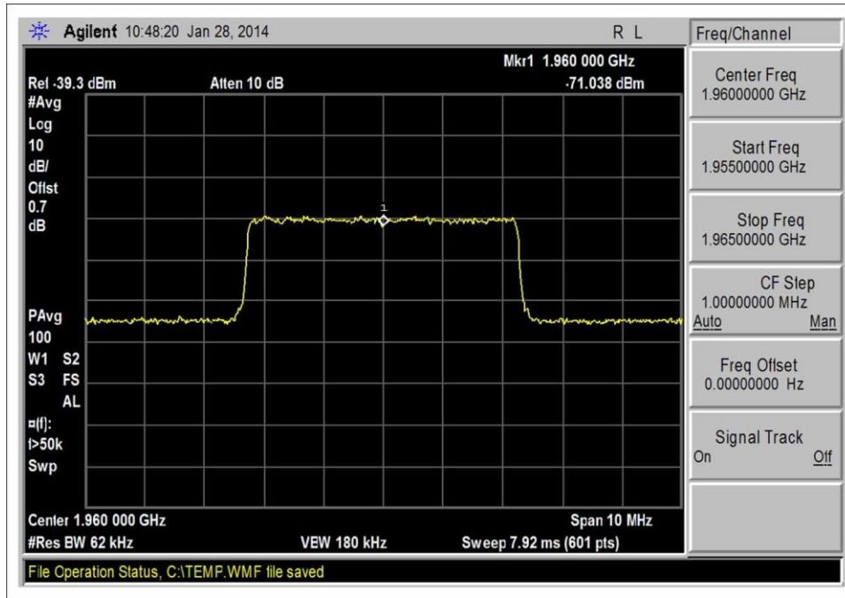
LTE_DL 1930-1990_Input
