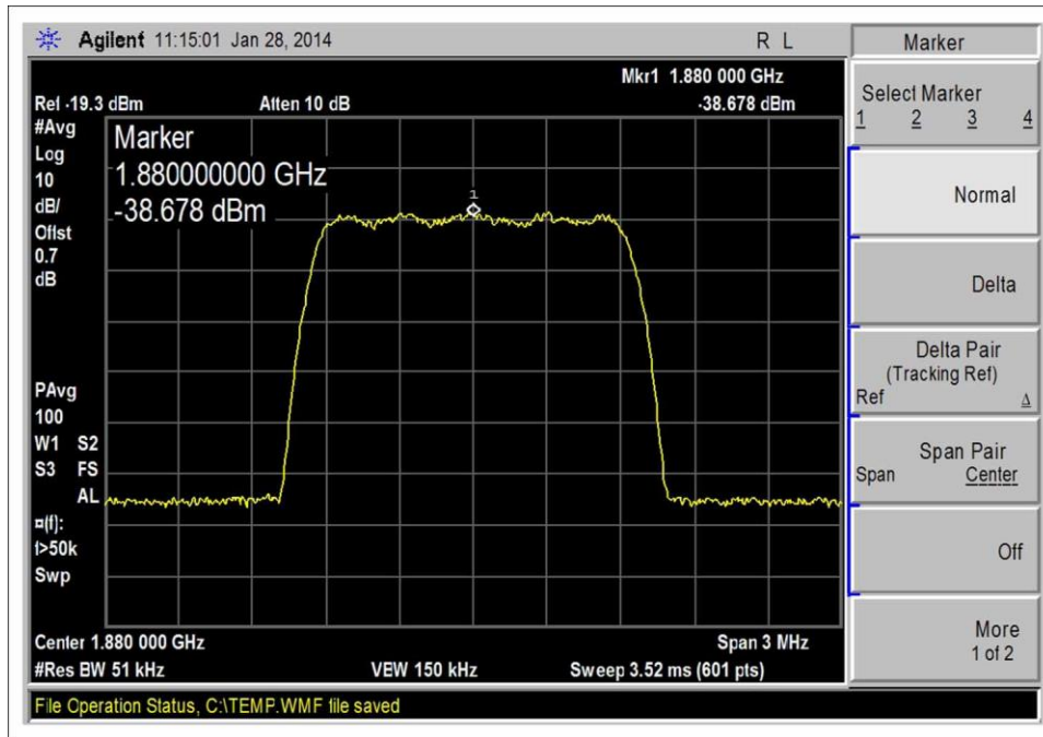
CDMA_UL 1850-1910_Input
