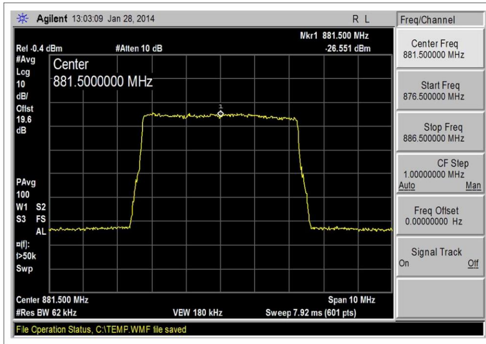
LTE_DL 869-894_Output
