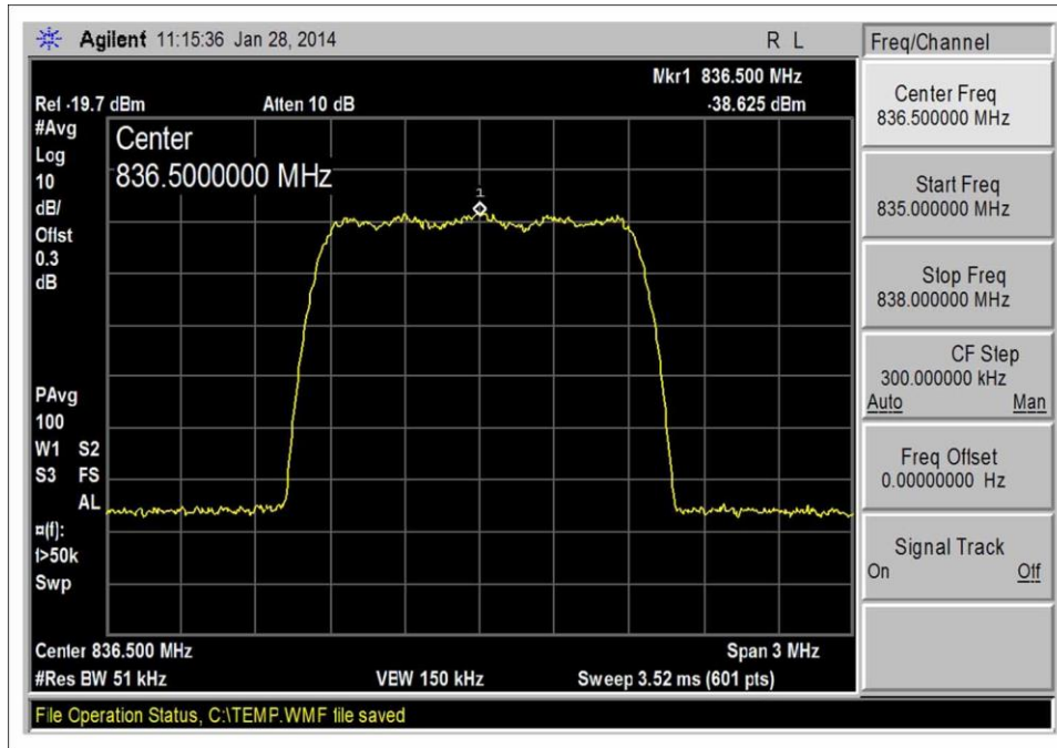
CDMA_UL 824-849_Input
