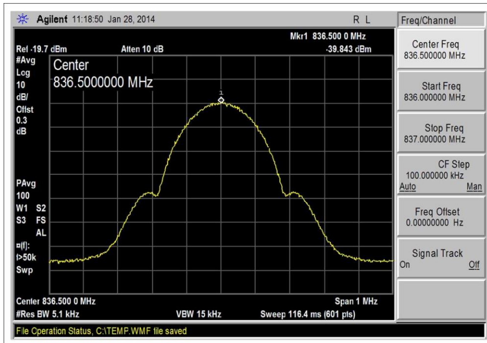
GSM_UL 824-849_Input
