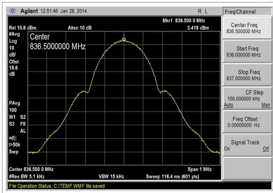
GSM_UL 824-849_Output
