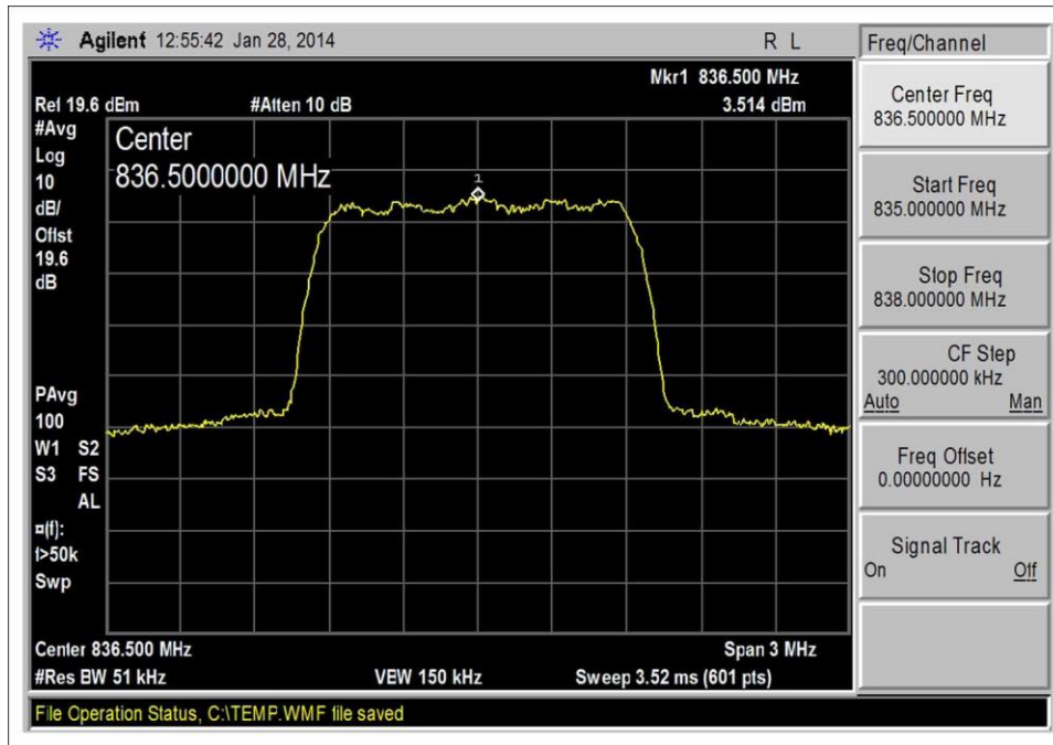
CDMA_UL 824-849_Output
