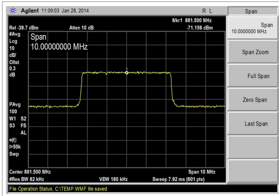
LTE_DL 869-894_Input
