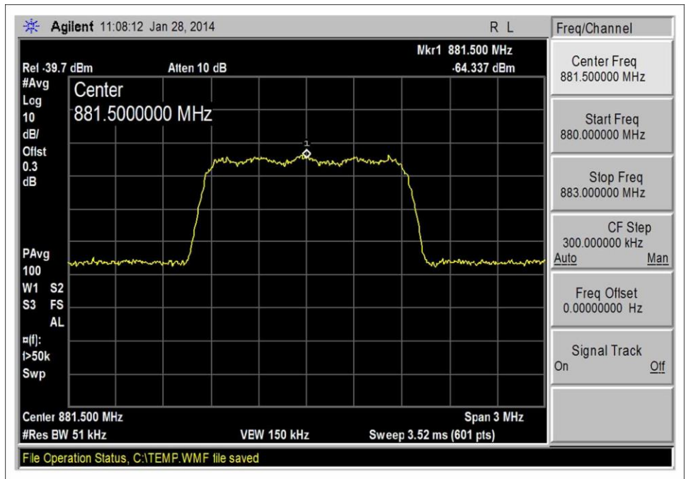
CDMA_DL 869-894_Input
