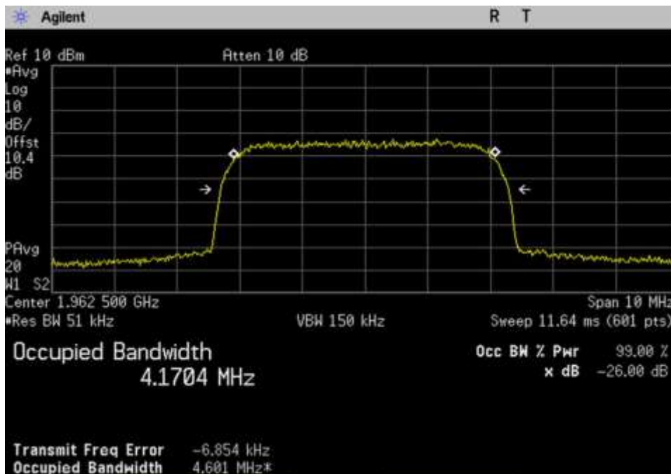
7.10 OBW-Out_DL_1930-1995_WCDMA_1962.5MHz
