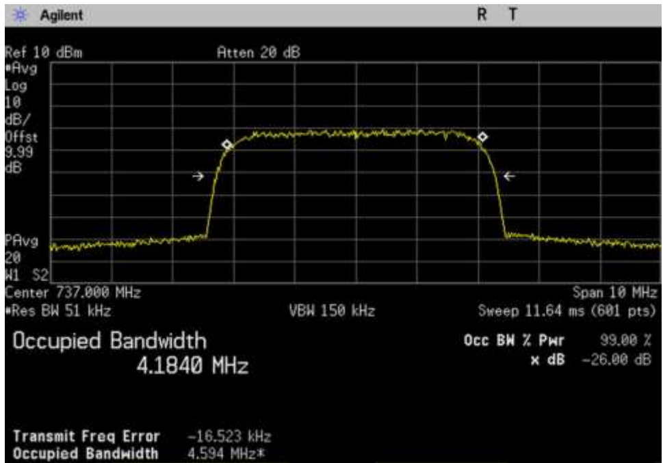
7.10 OBW-Out_DL_728-746_WCDMA_737MHz
