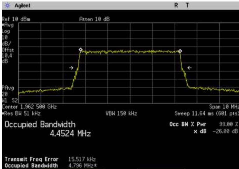
7.10 OBW-Out_DL_1930-1995_LTE_1962.5MHz
