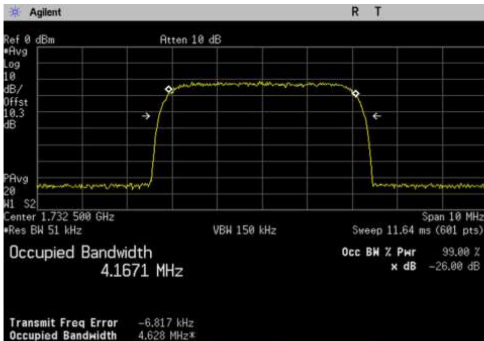
7.10 OBW-In_UL_1710-1755_WCDMA_1732.5MHz
