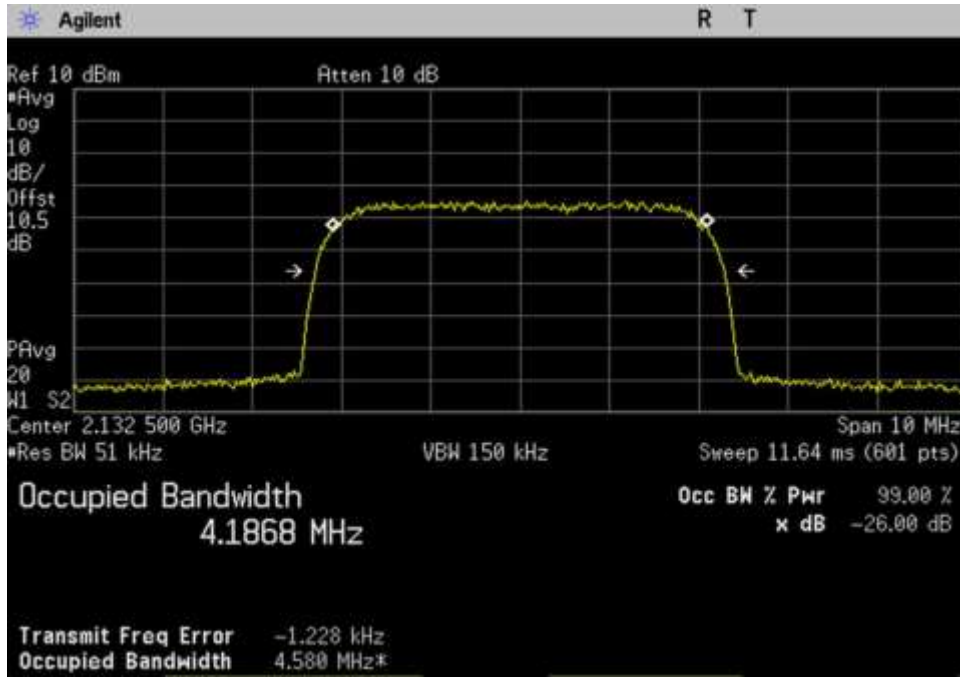
7.10 OBW-Out_DL_2110-2155_WCDMA_ 2132.5MHz
