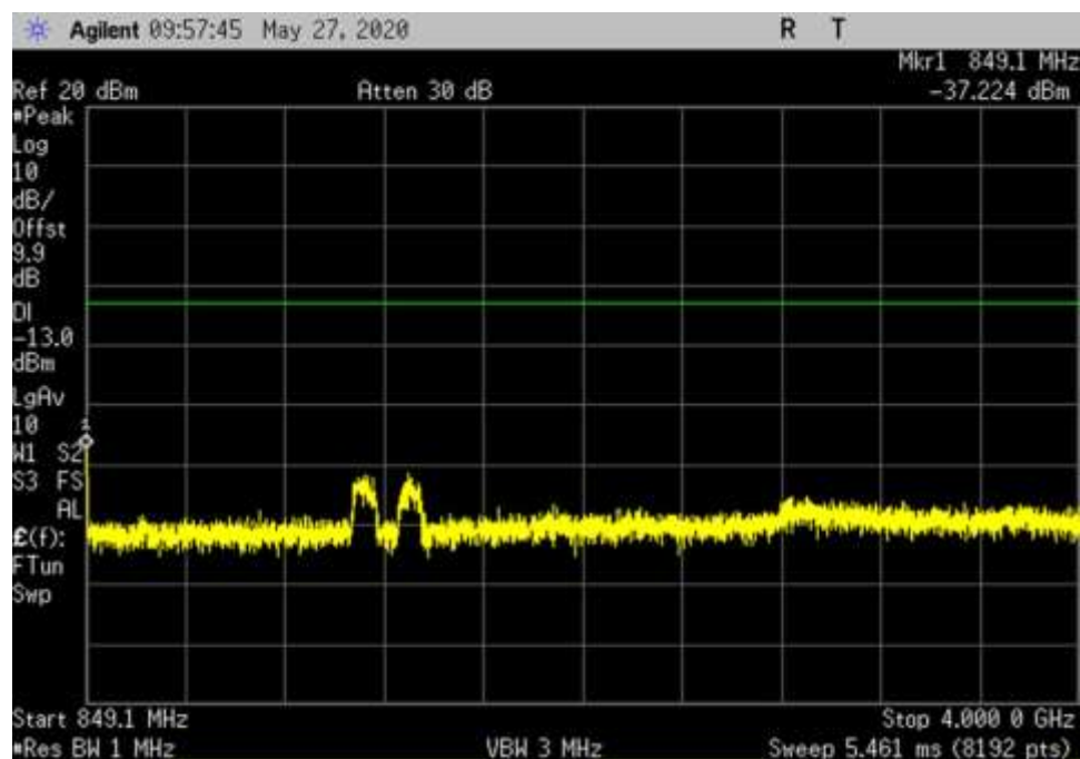
UL_824-849_ 849.1- 4000MHz
