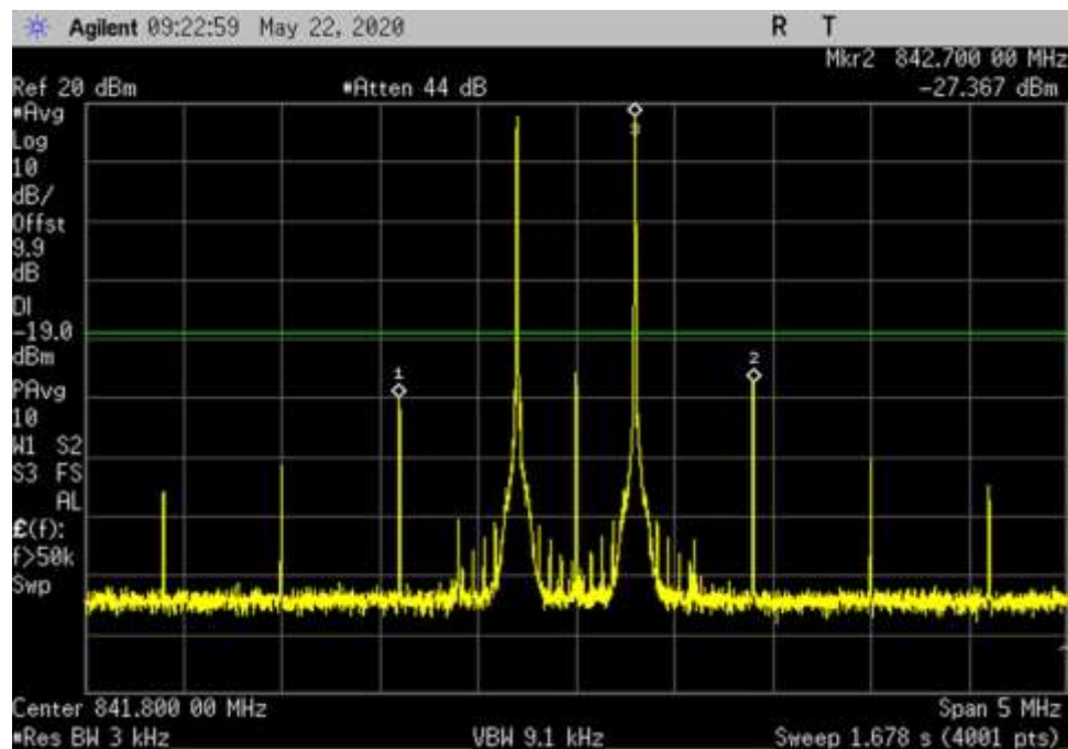
UL_824-849_+10dB_841.8MHz
