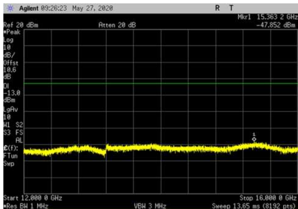
DL_2110-2155_ 12000- 16000MHz
