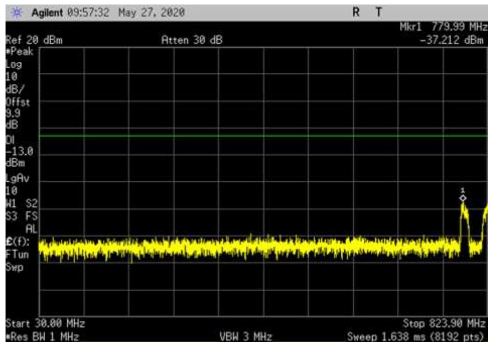
UL_824-849_ 30- 823.9MHz
