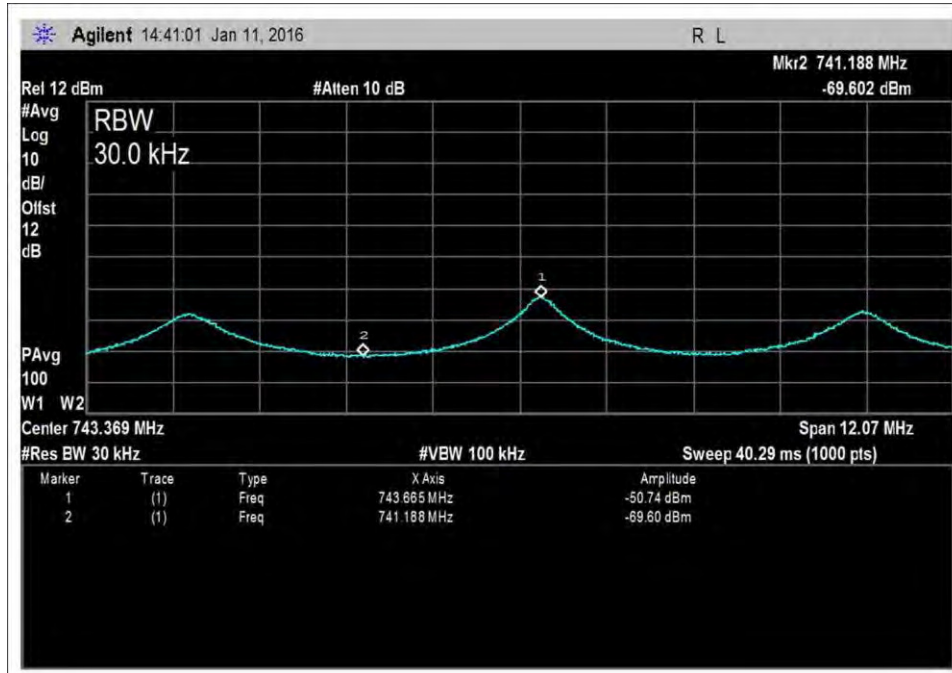
DL-728-746-AWGNL+0
