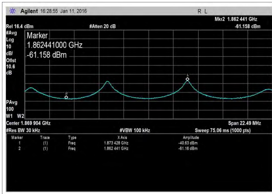
UL-1850-1915-AWGNL+1
