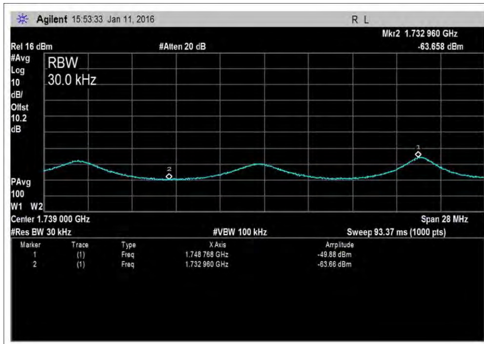
UL-1710-1755-AWGNL+2
