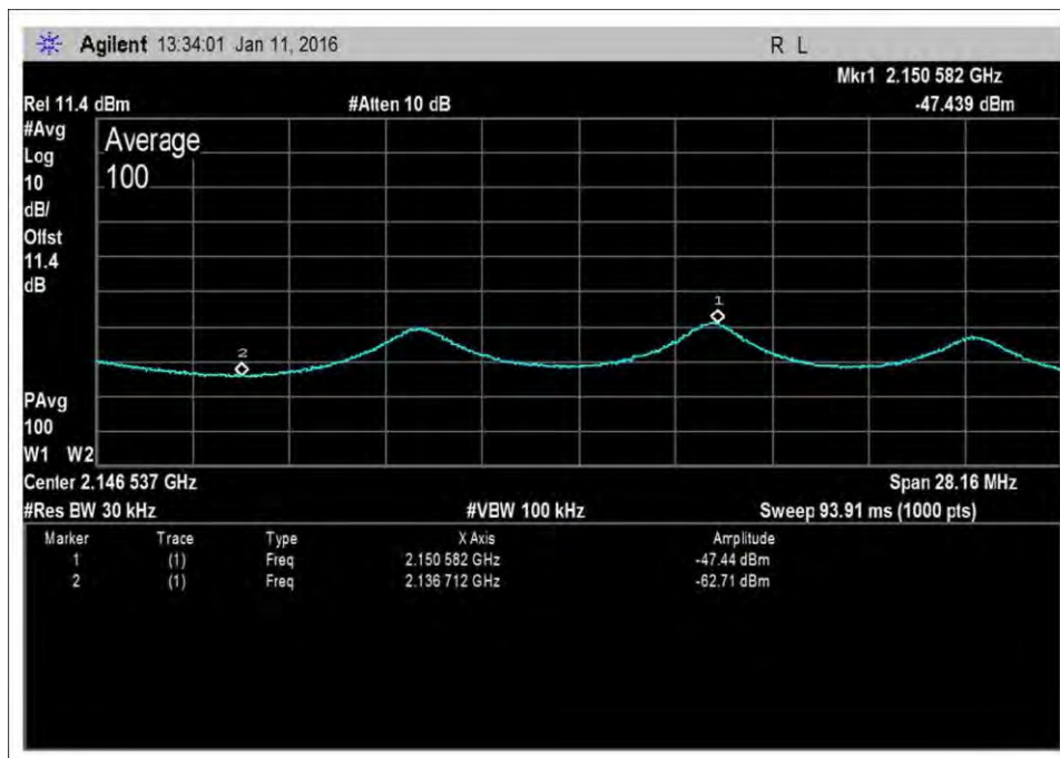
DL-2110-2155-AWGNL+1
