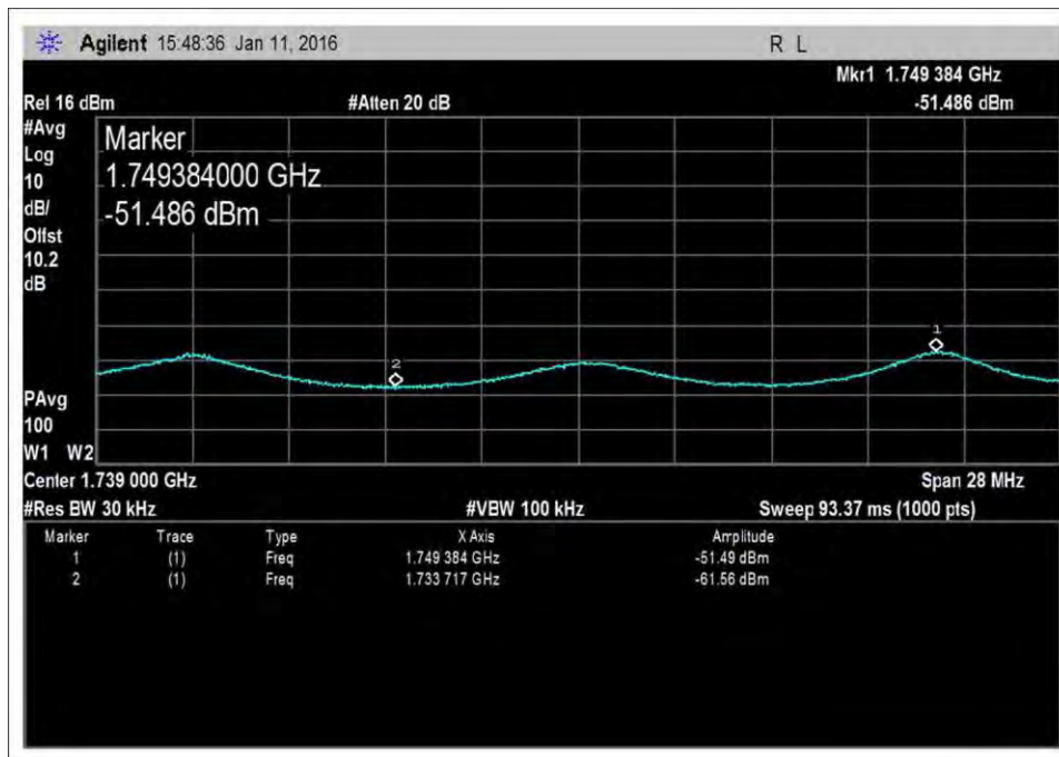
UL-1710-1755-AWGNL+5
