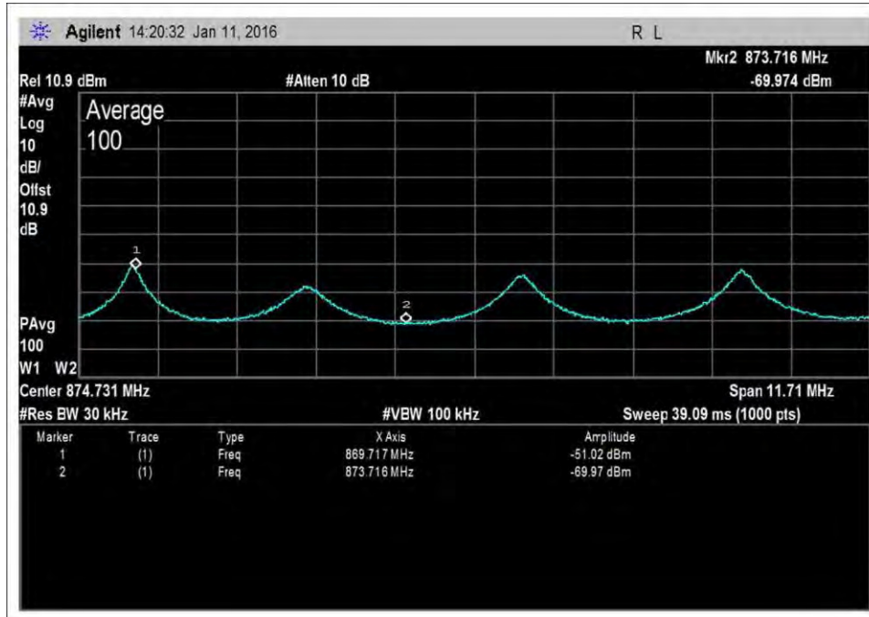
DL-869-894-AWGNR+0
