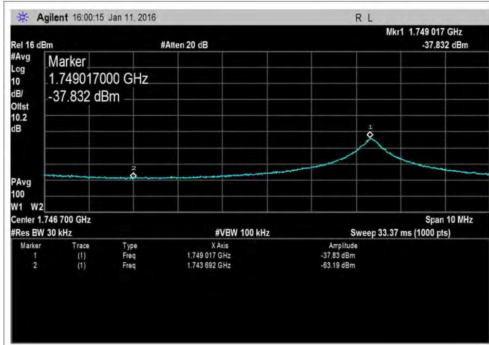
UL-1710-1755-AWGNL-1
