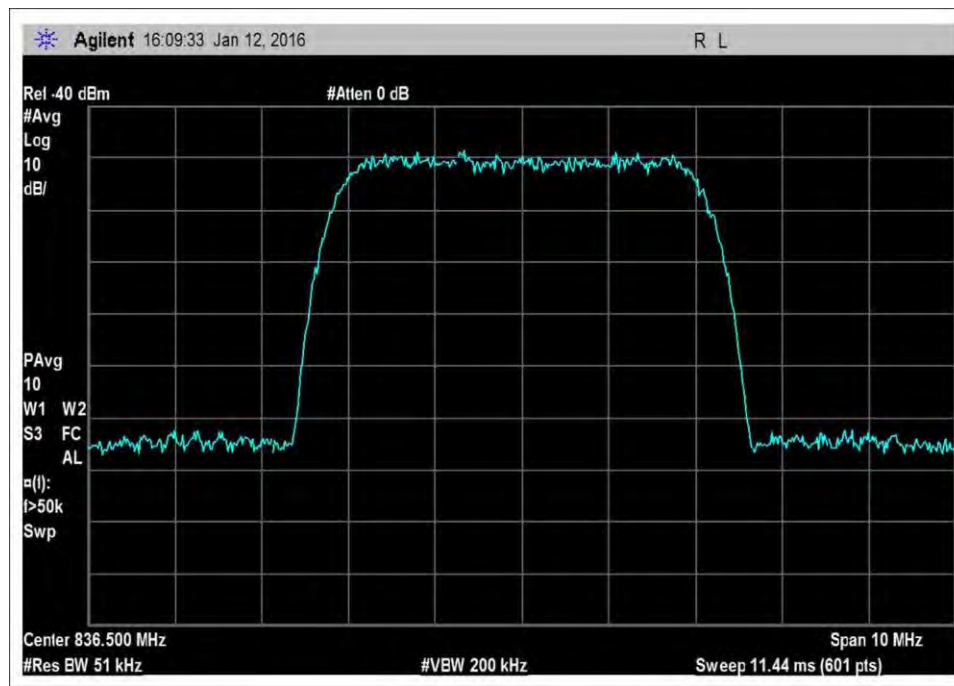
7.10_OBW_UL_824-849MHz_WCDMA
