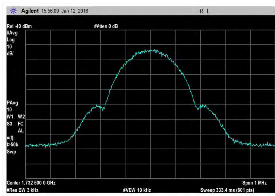
7.10_OBW_UL_1710-1755MHz_GSM
