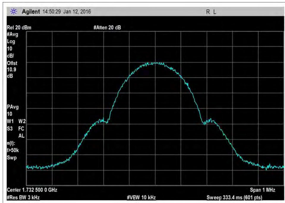
7.10_OBW_UL_1710-1755MHz_GSM
