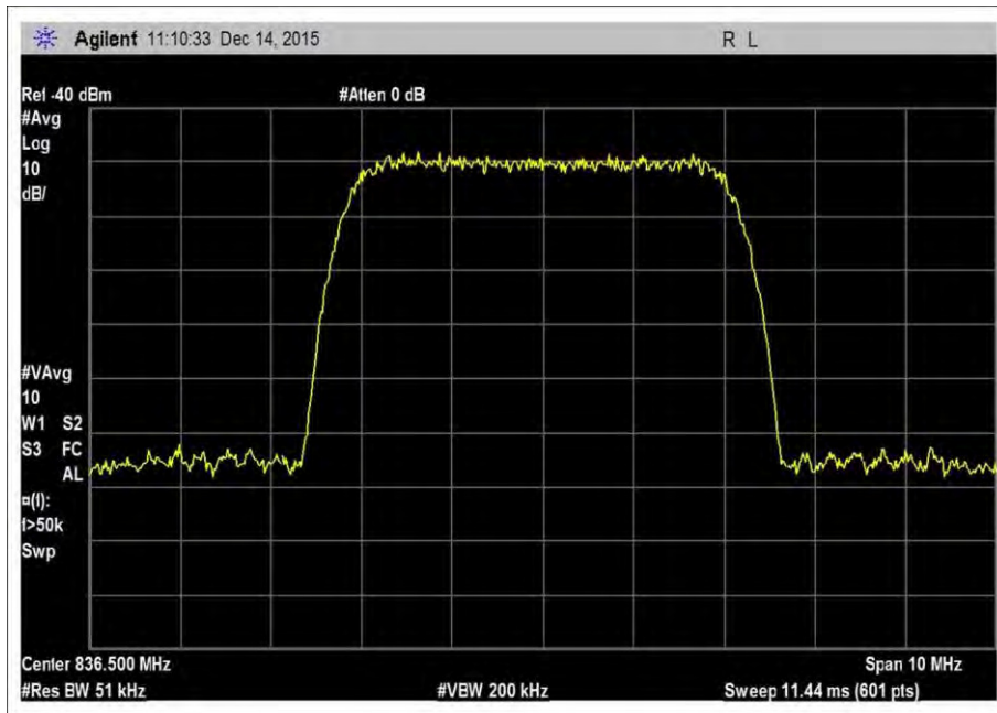
7.10_OBW_UL_824-849MHz_WCDMA
