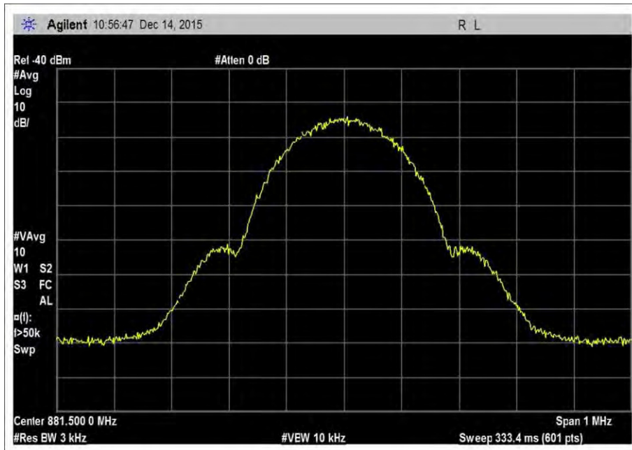
7.10_OBW_DL_869-894MHz_GSM
