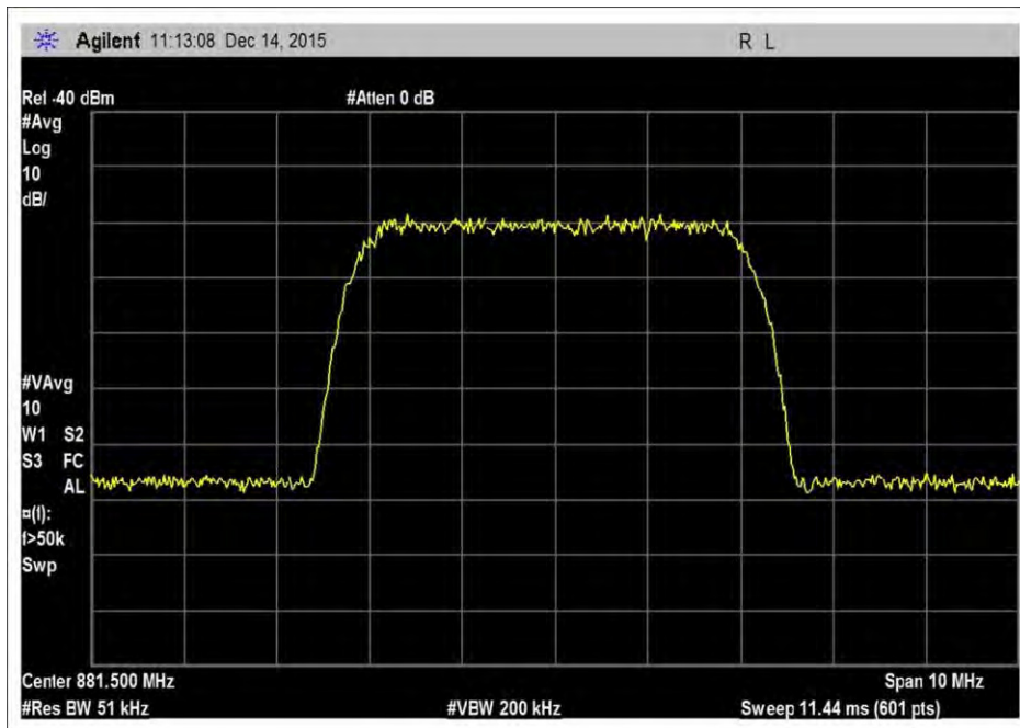
7.10_OBW_DL_869-894MHz_WCDMA
