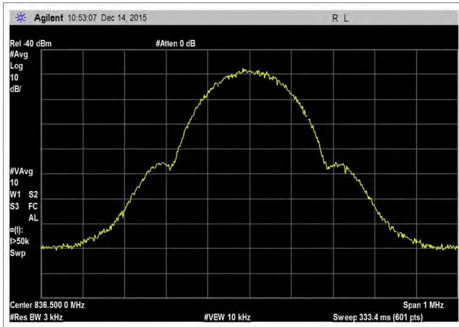
7.10_OBW_UL_824-849MHz_GSM
