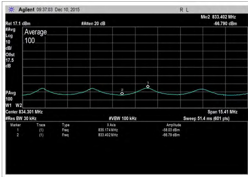
UL-824-849-AWGNR+4
