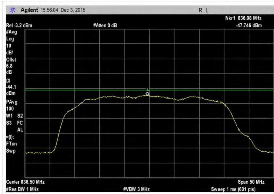
7.7_Noise_UL_824-849MHz
