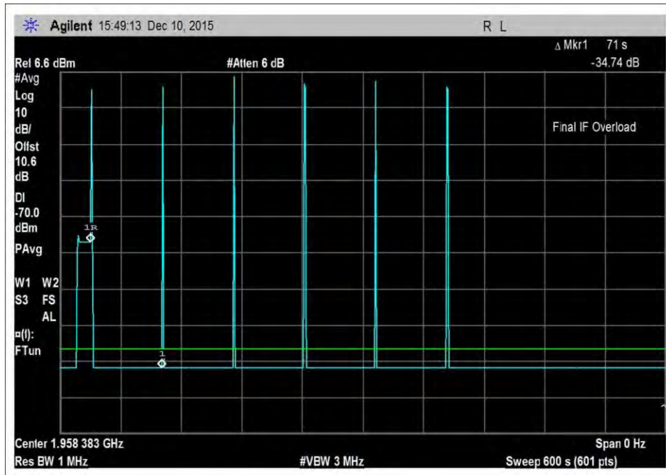
7.11_osc_DL-1930-1995MHz-600sec
