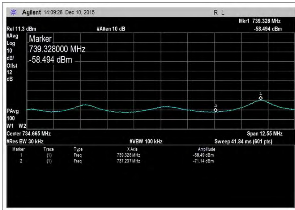
DL-728-746-AWGNR+3
