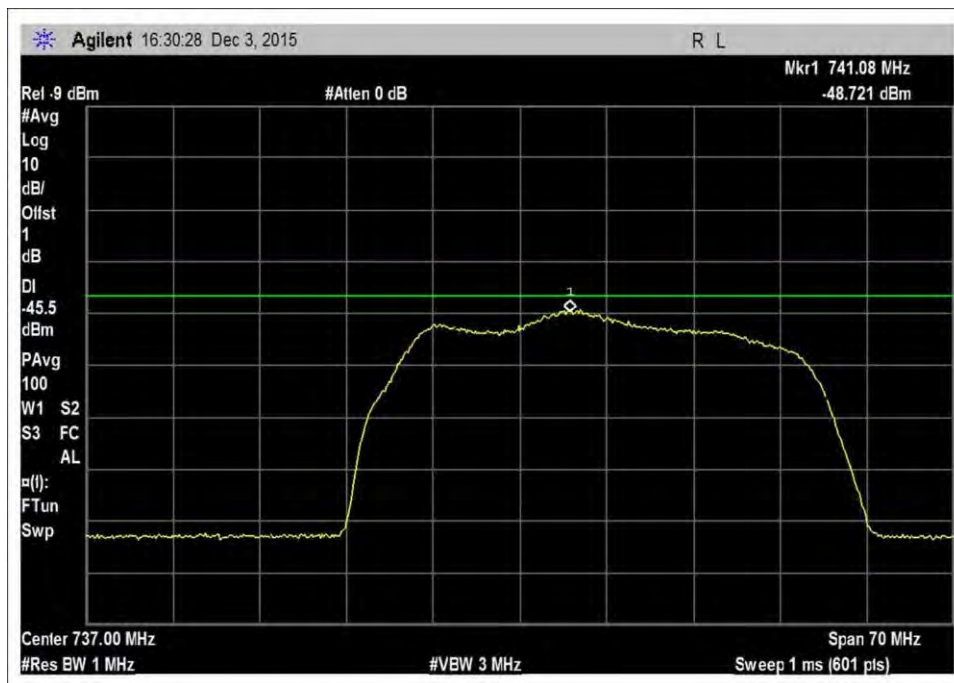
7.7_Noise_DL_728-746MHz-Zoom
