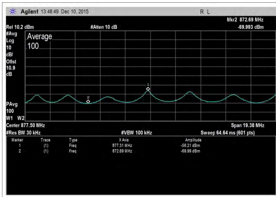
DL-869-894-AWGNR+4
