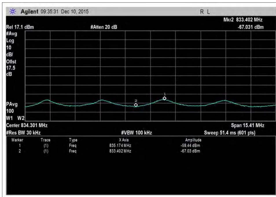
UL-824-849-AWGNR+5
