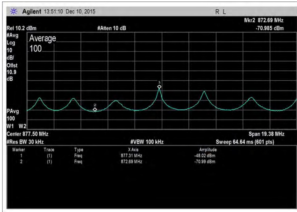
DL-869-894-AWGNR+1
