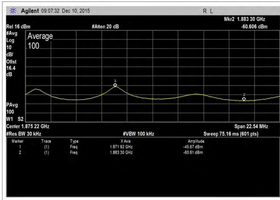
UL-1850-1915-AWGNR+0
