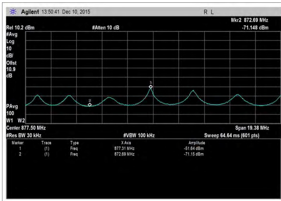
DL-869-894-AWGNR+2
