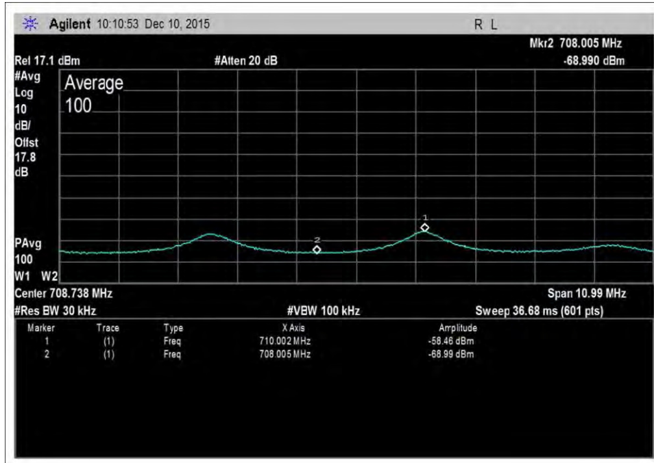
UL-698-716-AWGNL+3
