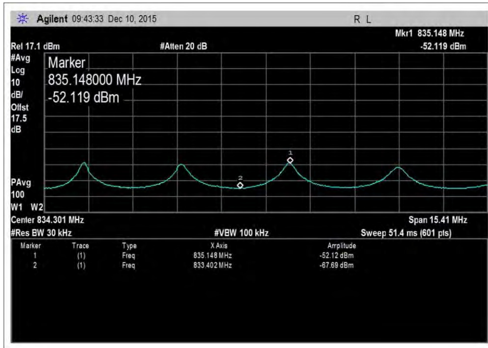
UL-824-849-AWGNR+0
