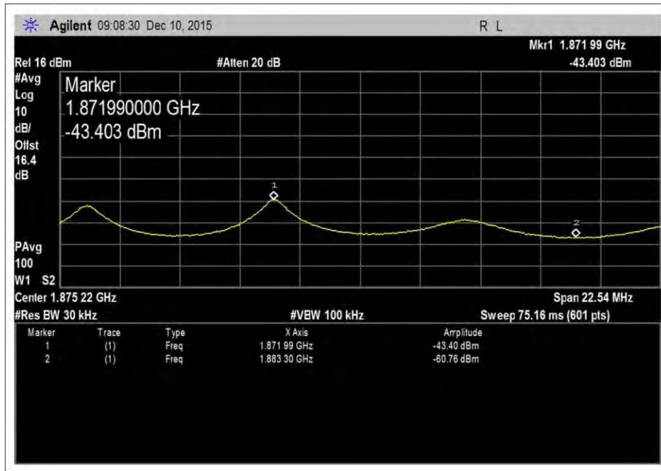
UL-1850-1915-AWGNR-1
