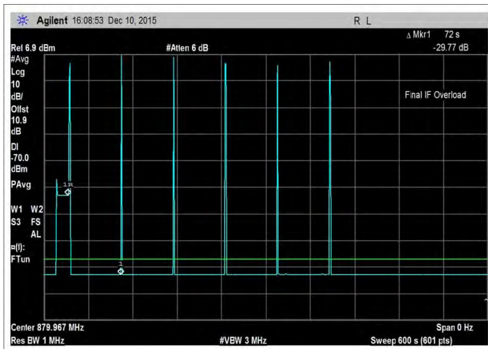
7.11_osc_DL-869-894MHz-600
