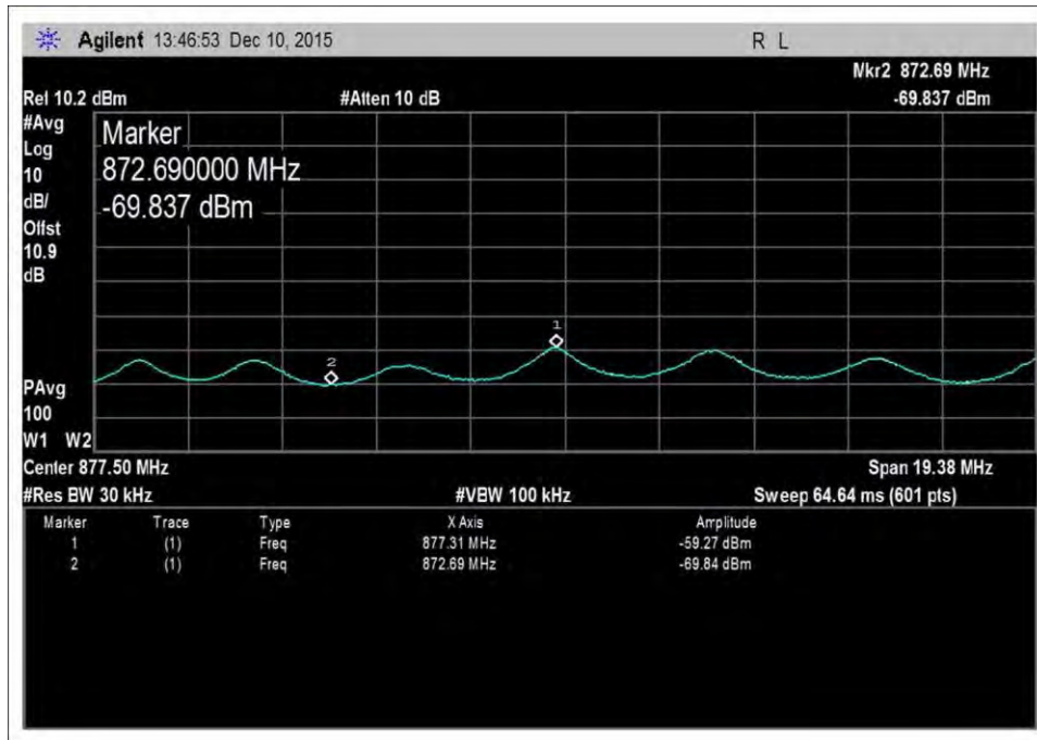
DL-869-894-AWGNR+5
