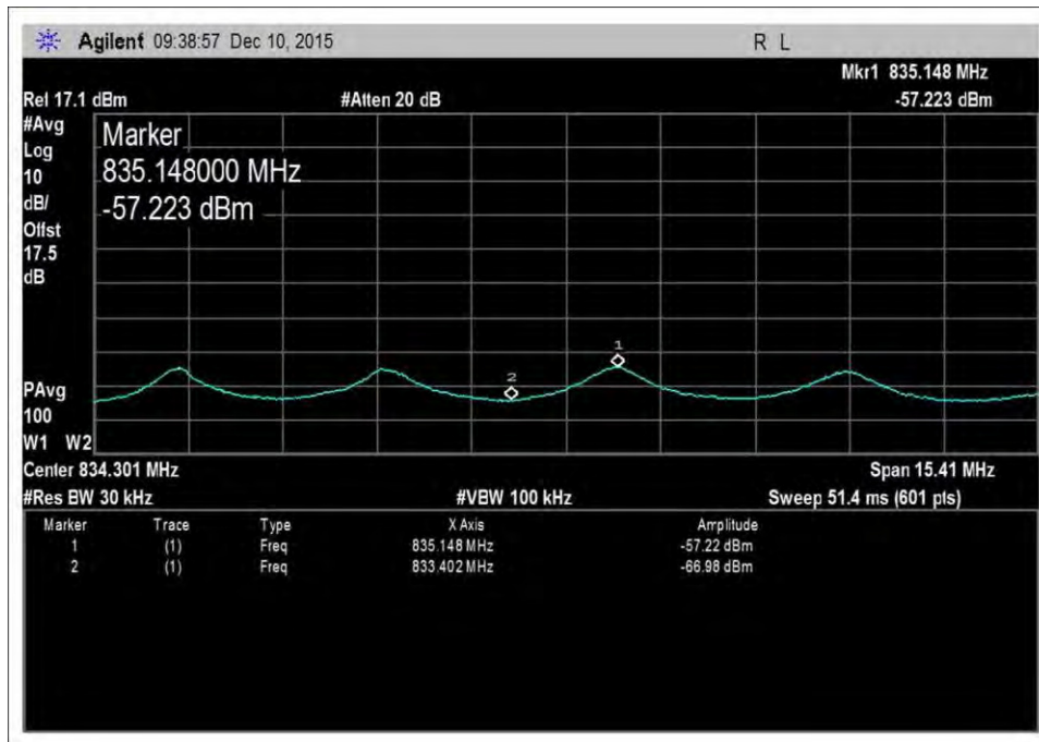
UL-824-849-AWGNR+3
