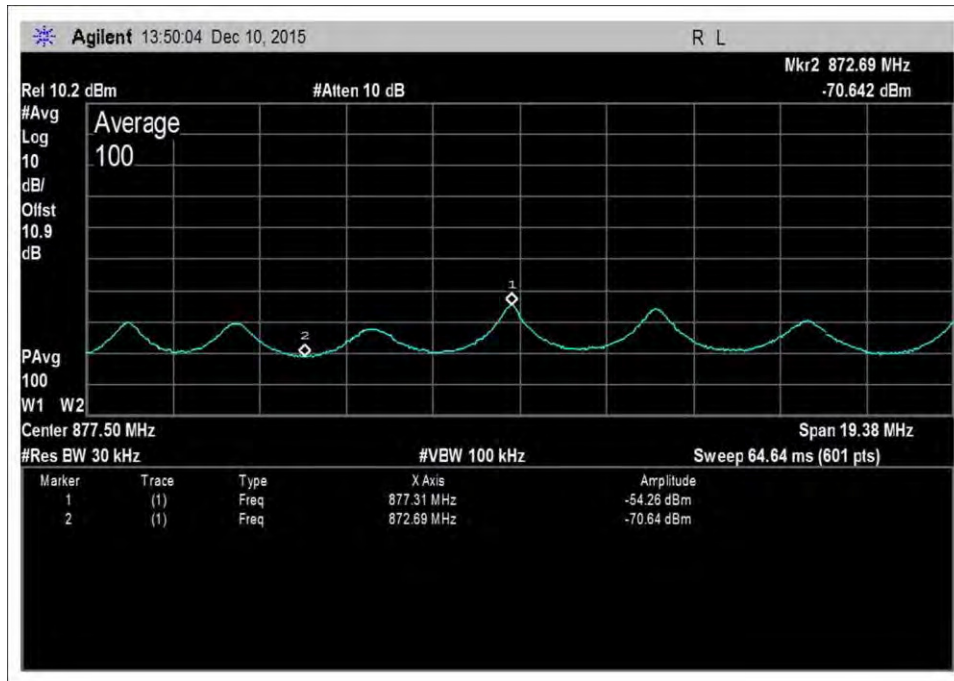
DL-869-894-AWGNR+3
