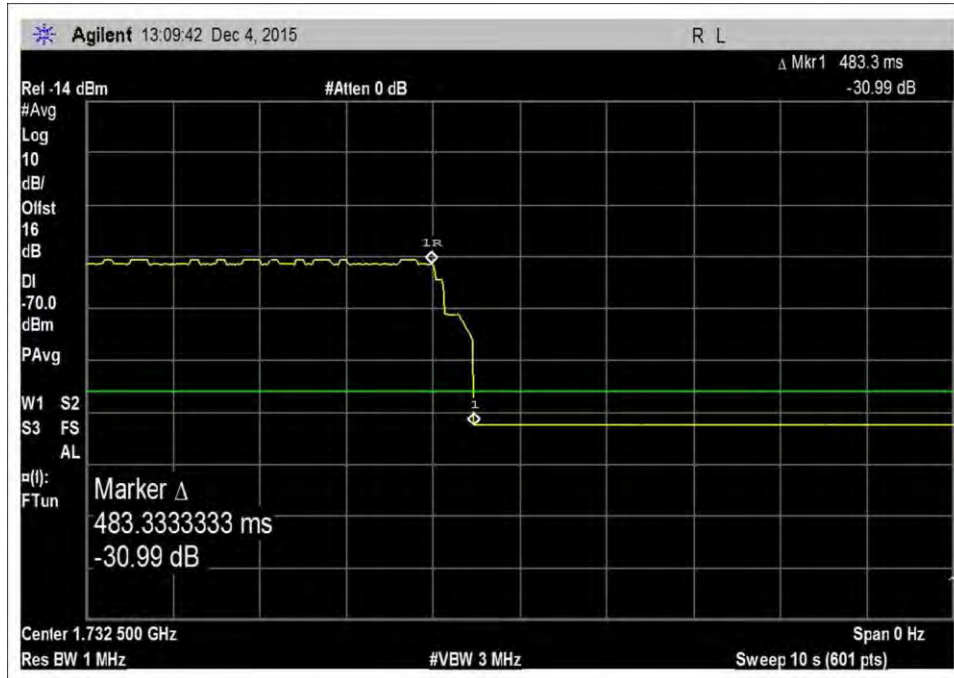
7.7_VarNoise_UL_1710-1755MHz
