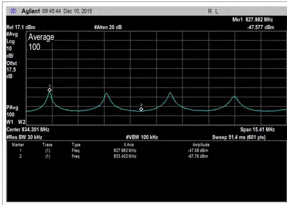
UL-824-849-AWGNR-1
