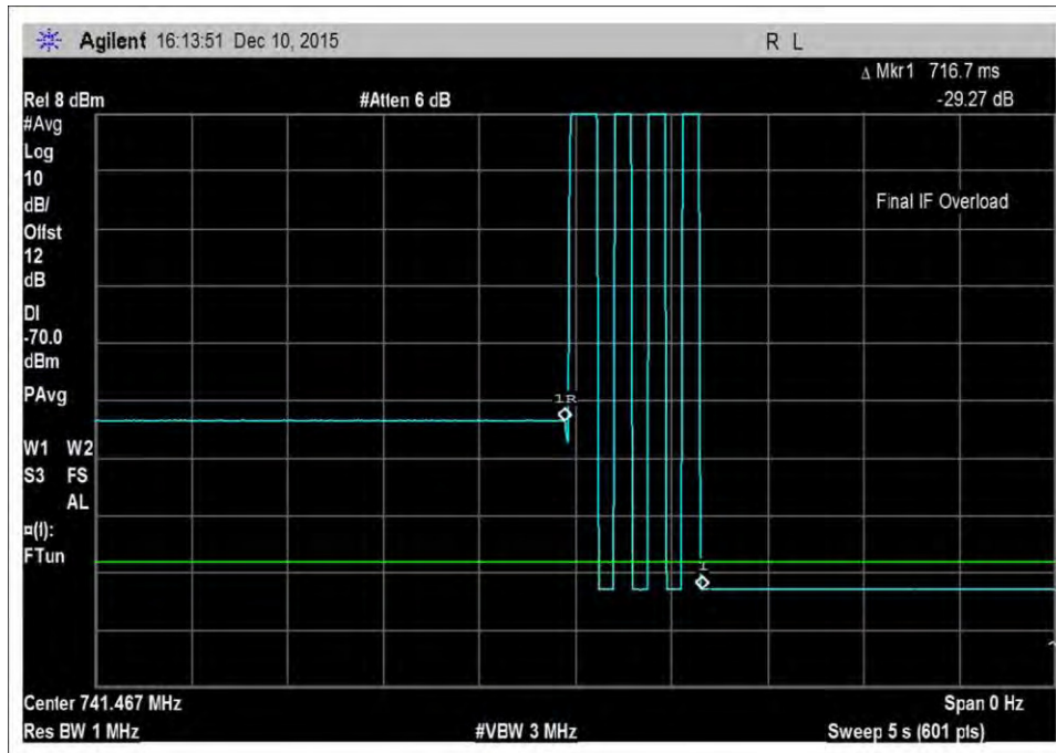
7.11_osc_DL-728-746MHz
