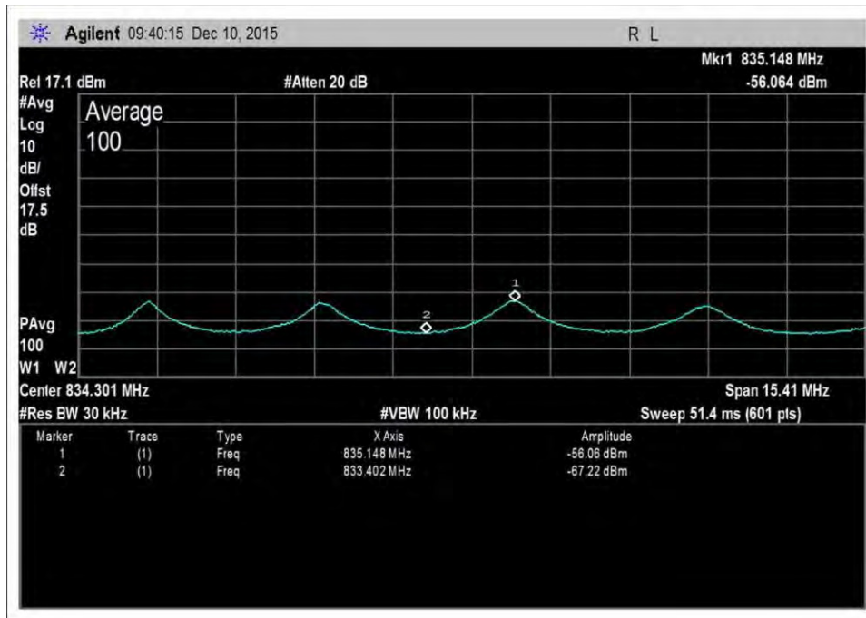
UL-824-849-AWGNR+2
