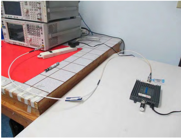
7.7.1 Test Setup
