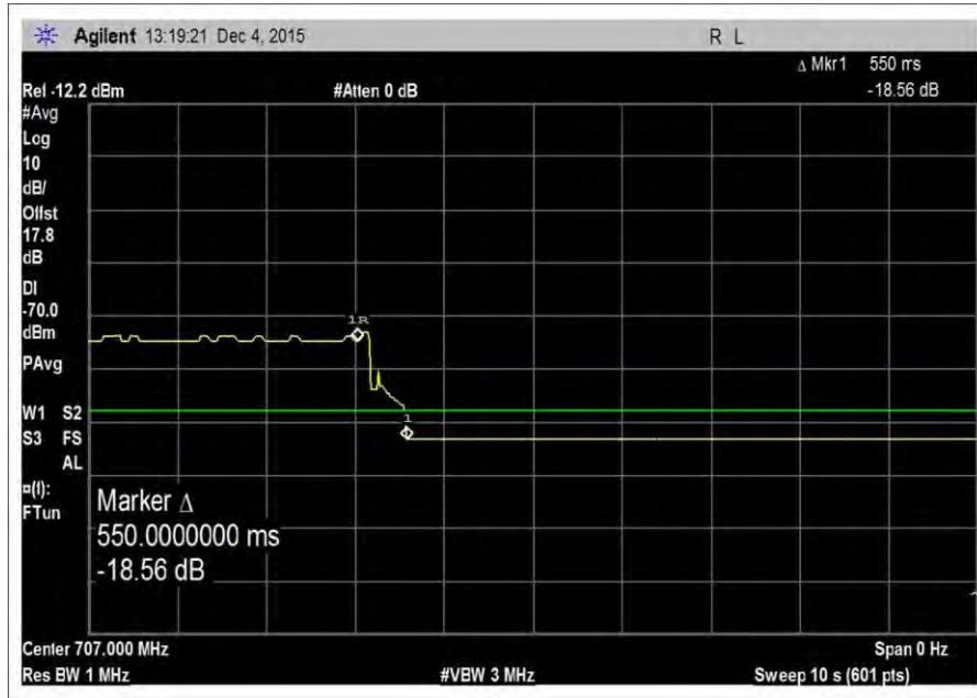
7.7_VarNoise_UL_698-716MHz
