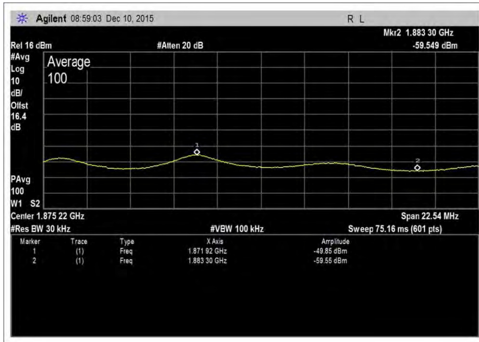
UL-1850-1915-AWGNR+4
