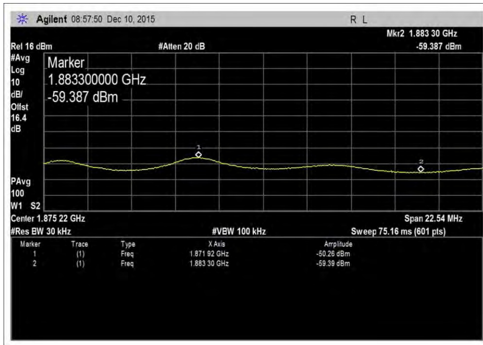
UL-1850-1915-AWGNR+5
