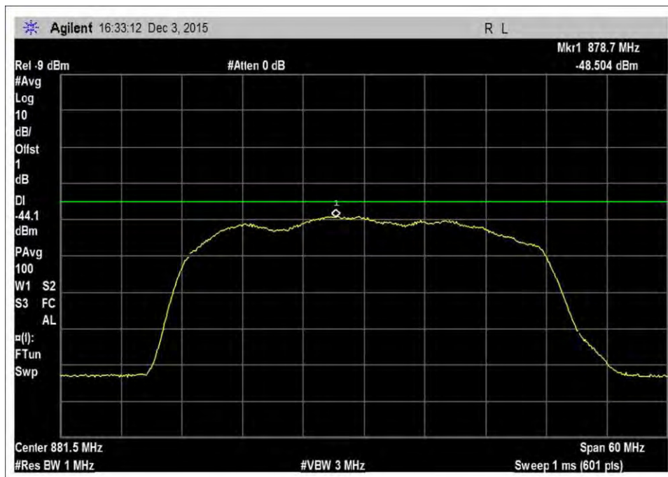
7.7_Noise_DL_869-894MHz-Zoom
