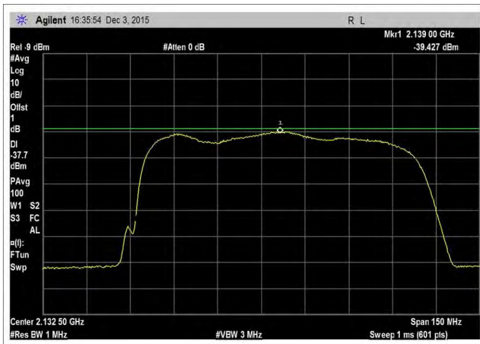
7.7_Noise_DL_2110-2155MHz
