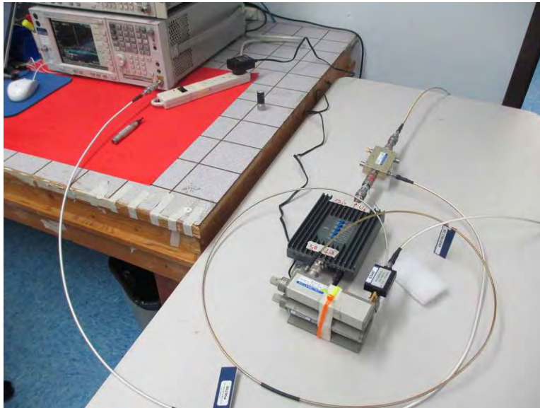
7.7.2 Test Setup
