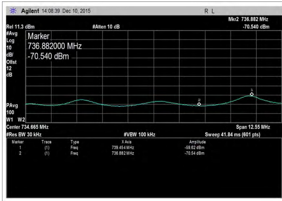
DL-728-746-AWGNR+4
