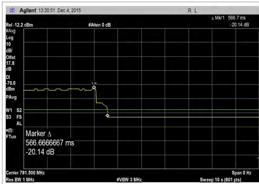
7.7_VarNoise_UL_776-787MHz
