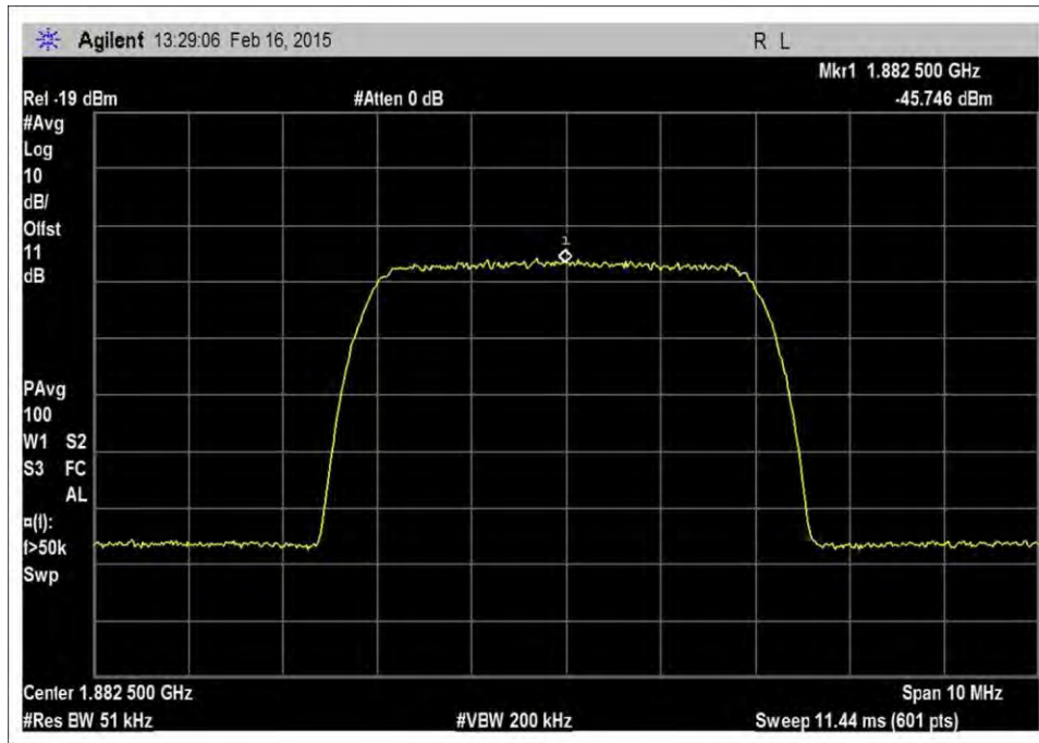
7.10_OBW_UL_1850-1915MHz_WCDMA_Input
