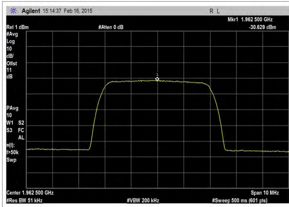
7.10_OBW_DL_1930-1995MHz_WCDMA_Output
