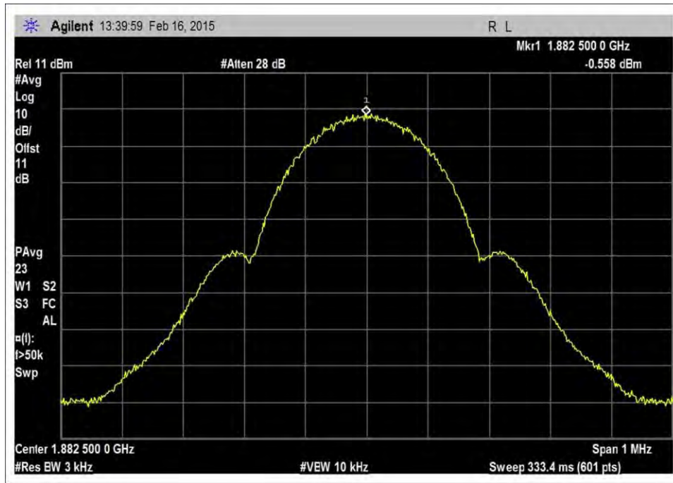
7.10_OBW_UL_1850-1915MHz_GSM_Output
