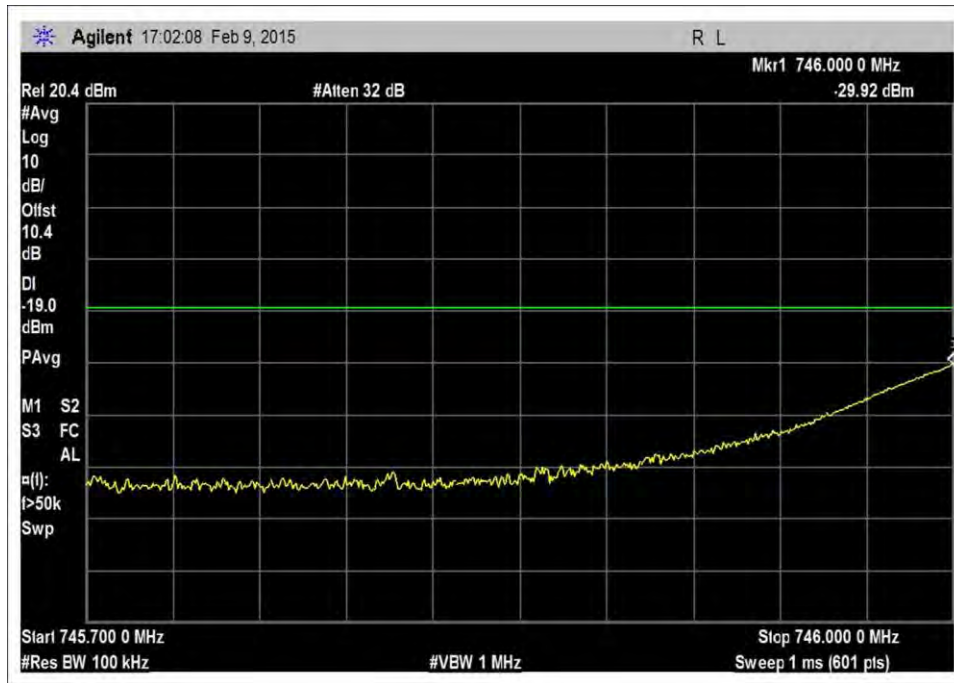
7.5_OBE_DL_746-757MHz_GSM_L_-48dBm
