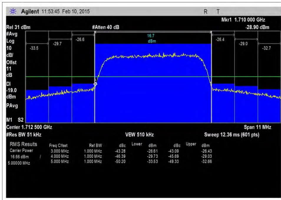
7.5_OBE_UL_1710-1755MHz_LTE_L_-26dBm
