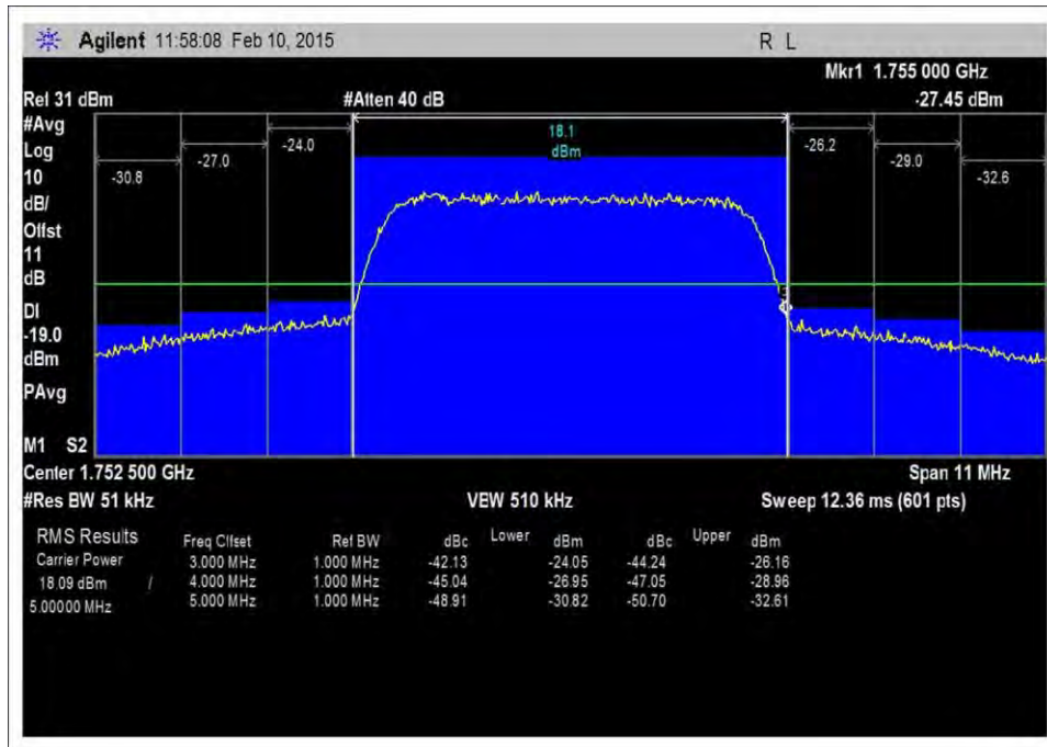
7.5_OBE_UL_1710-1755MHz_LTE_H_-24dBm
