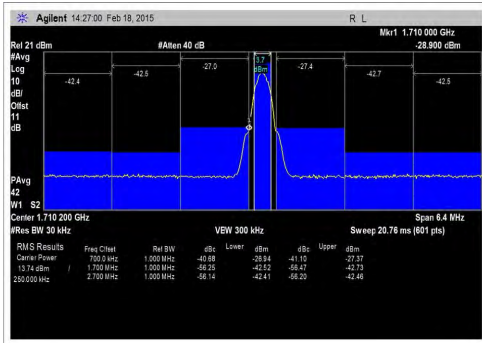
7.5_OBE_UL_1710-1755MHz_GSM_L_-27dBm
