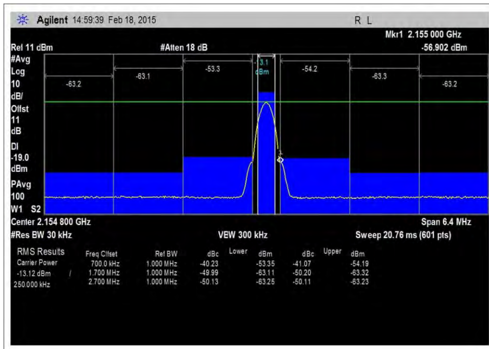
7.5_OBE_DL_2110-2155MHz_GSM_H_-48dBm
