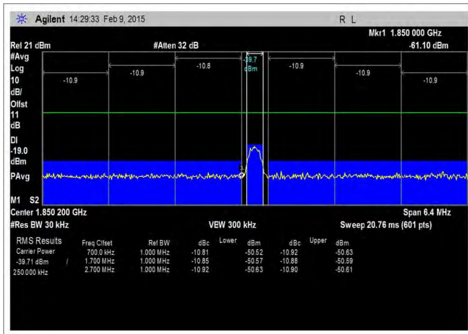
7.5_OBE_UL_1850-1915MHz_GSM_L_+10dBm
