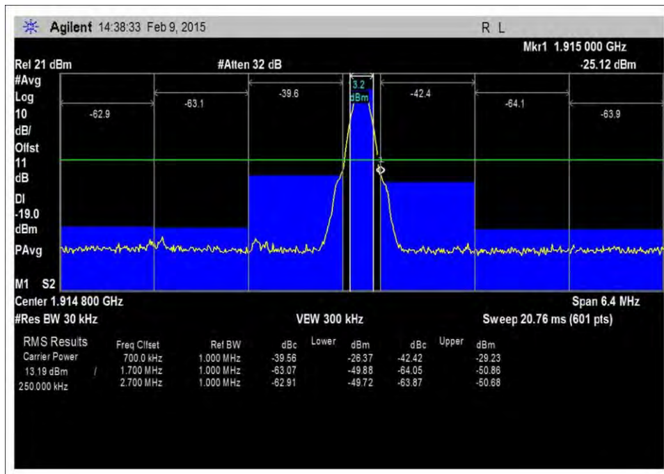
7.5_OBE_UL_1850-1915MHz_GSM_H_-5dBm
