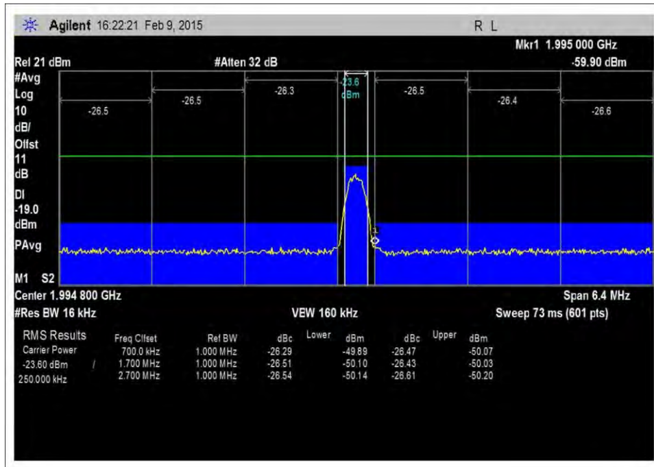
7.5_OBE_DL_1930-1995MHz_GSM_H_-55dBm
