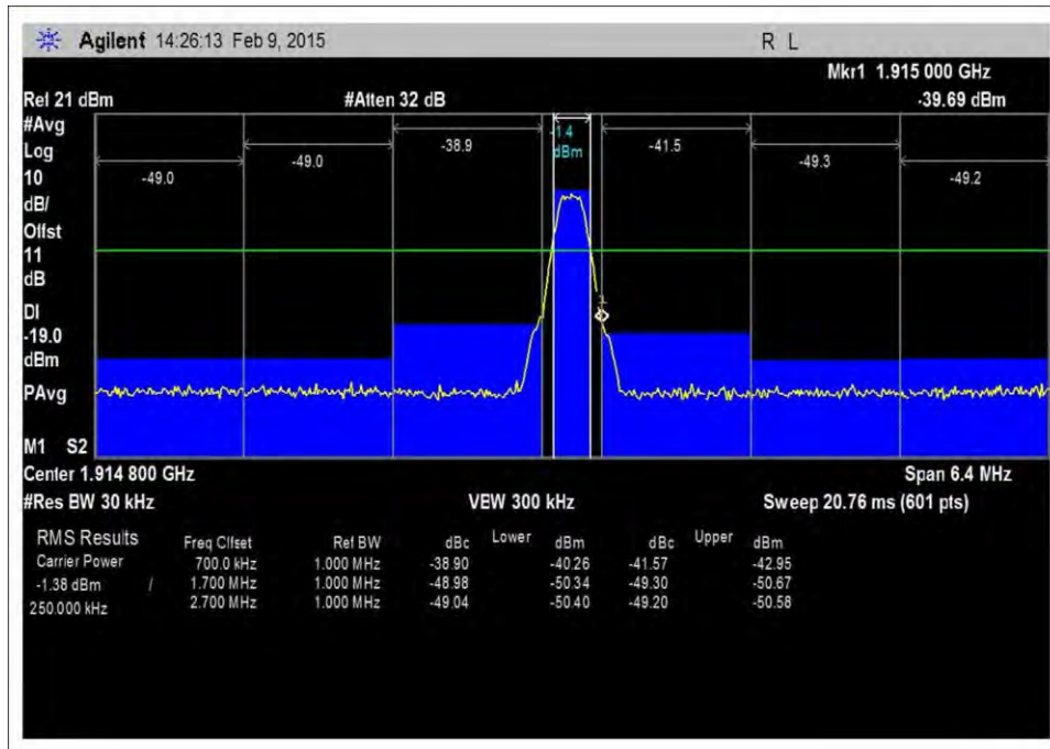
7.5_OBE_UL_1850-1915MHz_GSM_H_26
