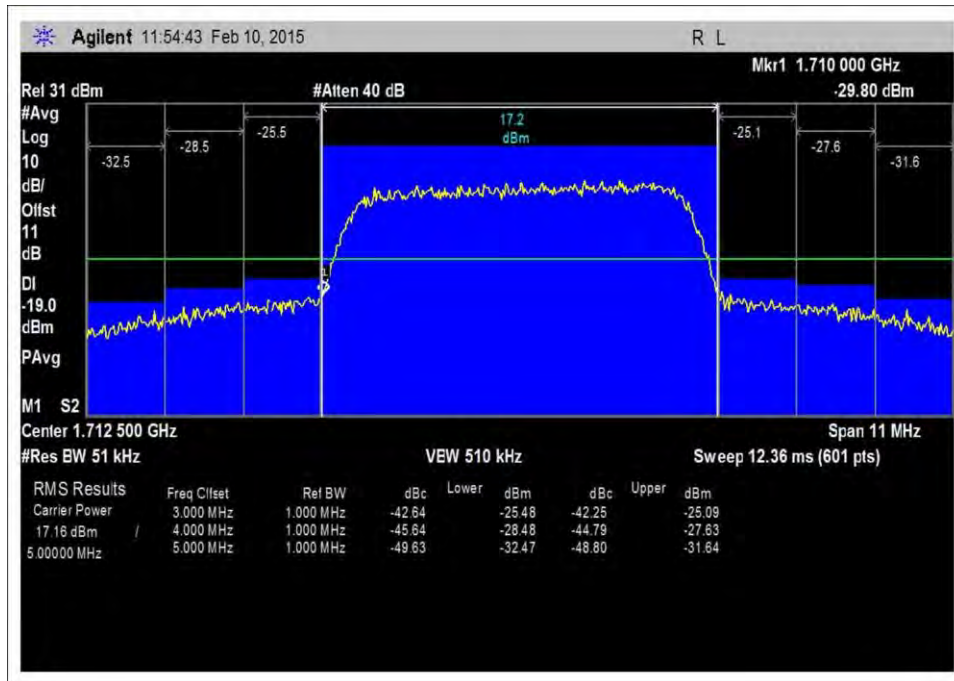
7.5_OBE_UL_1710-1755MHz_LTE_L_-20dBm
