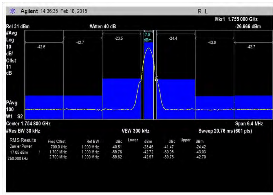
7.5_OBE_UL_1710-1755MHz_GSM_H_-26dBm
