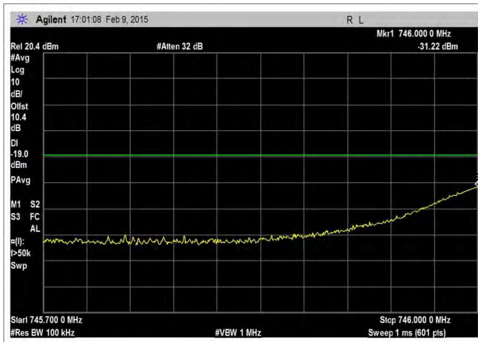
7.5_OBE_DL_746-757MHz_GSM_L_-54dBm
