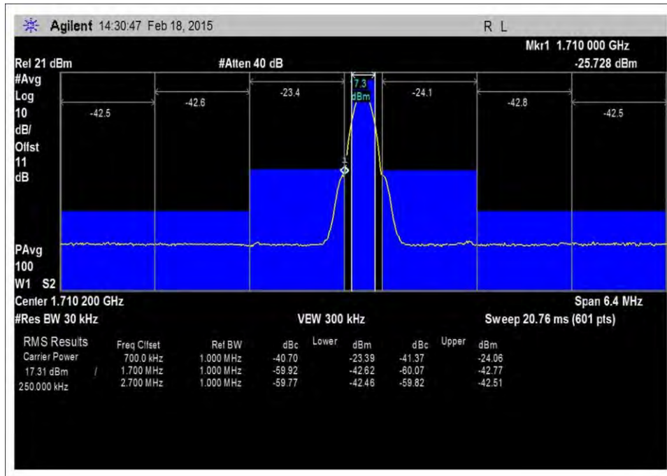
7.5_OBE_UL_1710-1755MHz_GSM_L_-18dBm
