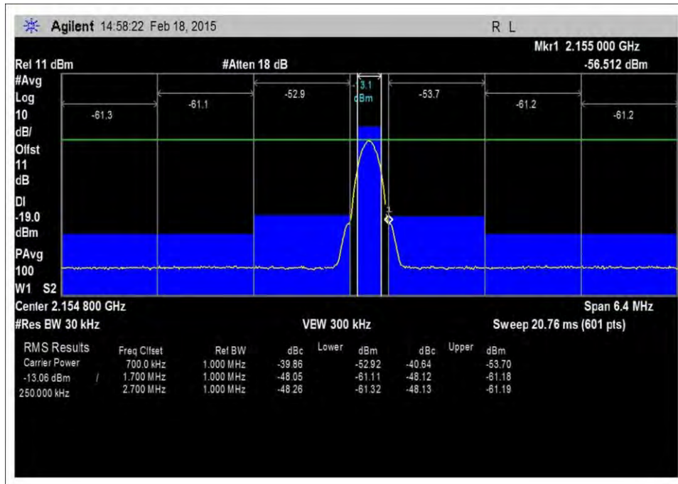
7.5_OBE_DL_2110-2155MHz_GSM_H_-53dBm
