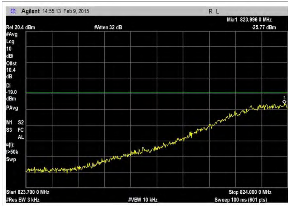
7.5_OBE_UL_824-849MHz_GSM_L_-21dBm
