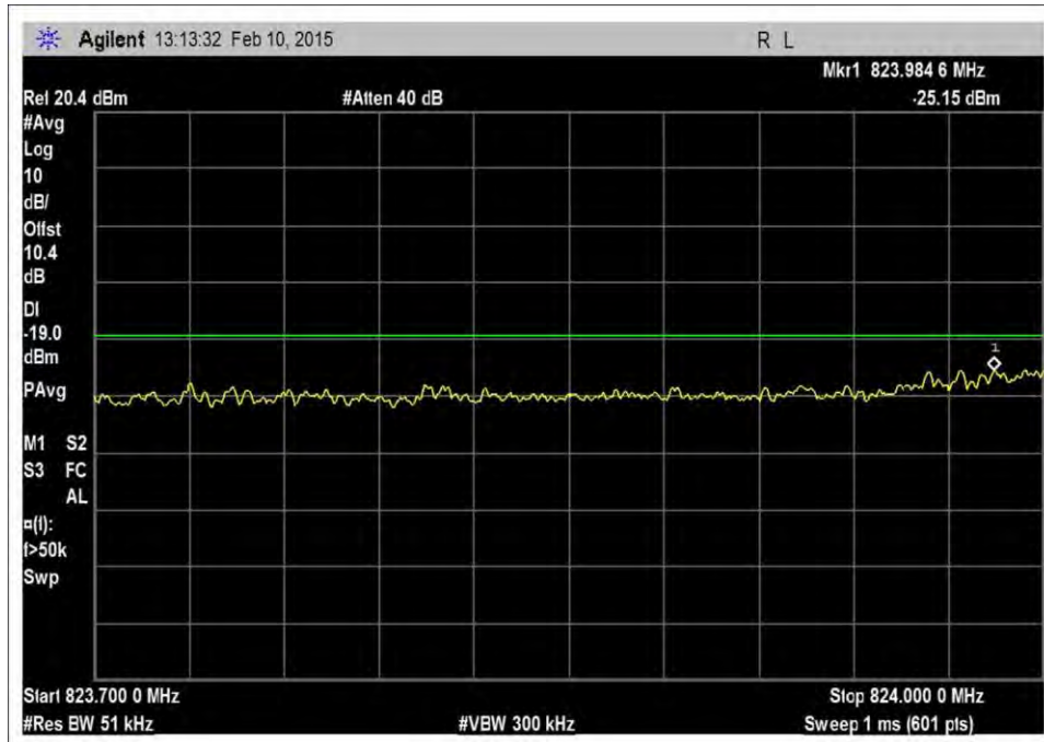
7.5_OBE_UL_824-849MHz_LTE_L_-26dBm
