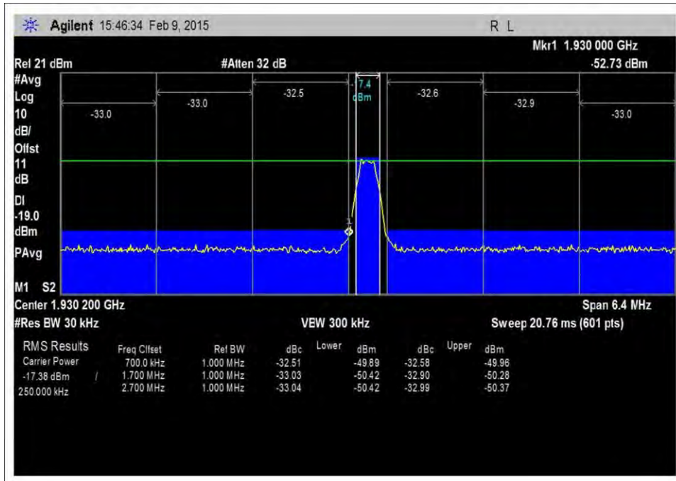
7.5_OBE_DL_1930-1995MHz_GSM_L_-54dBm
