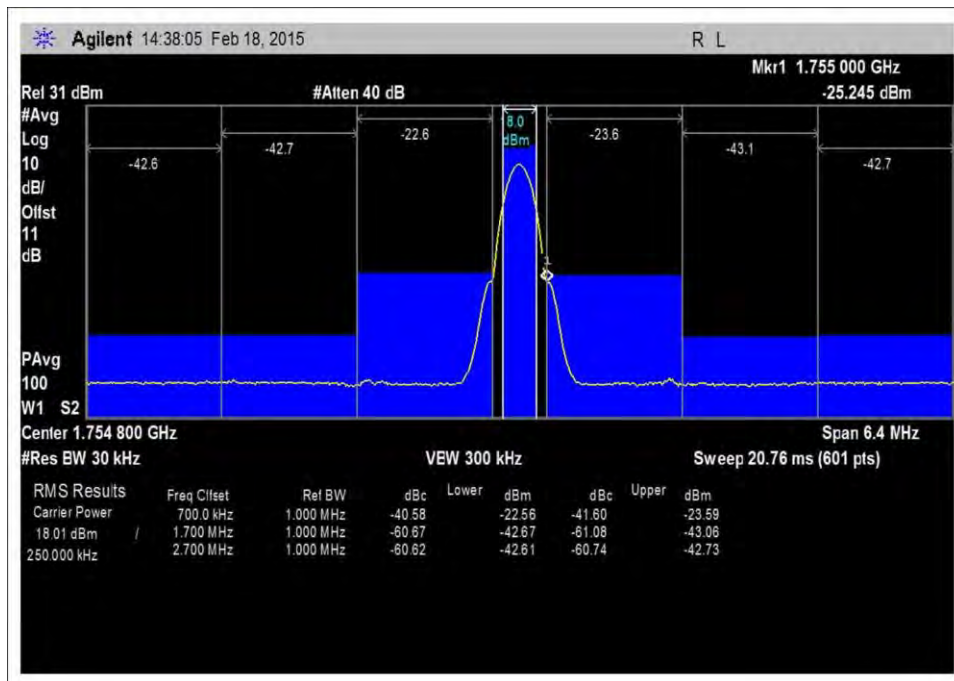
7.5_OBE_UL_1710-1755MHz_GSM_H_-21dBm
