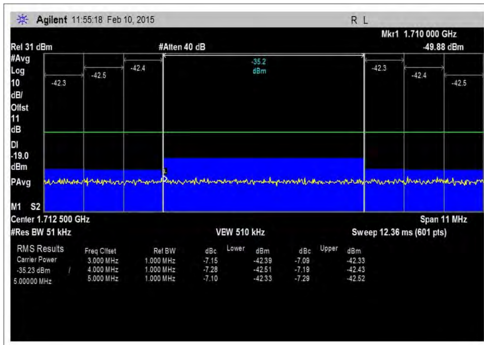
7.5_OBE_UL_1710-1755MHz_LTE_L_+10dBm
