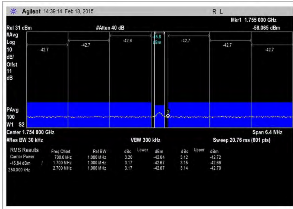
7.5_OBE_UL_1710-1755MHz_GSM_H_+10dBm
