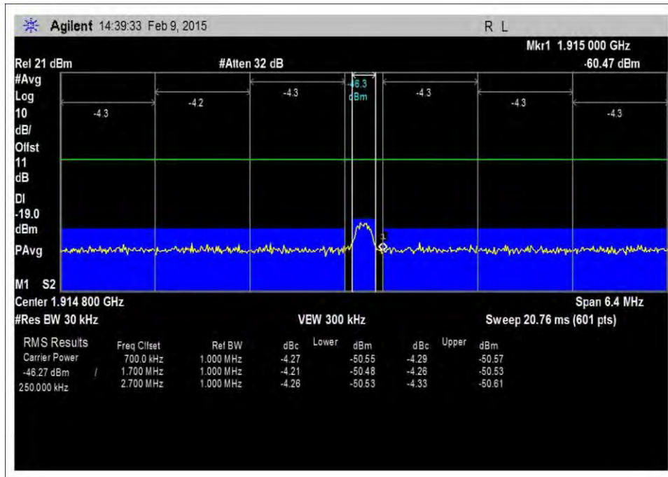
7.5_OBE_UL_1850-1915MHz_GSM_H_+10dBm
