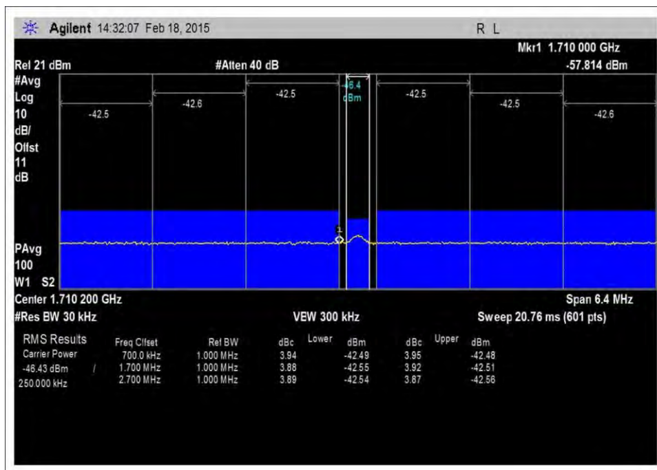
7.5_OBE_UL_1710-1755MHz_GSM_L_+10dBm
