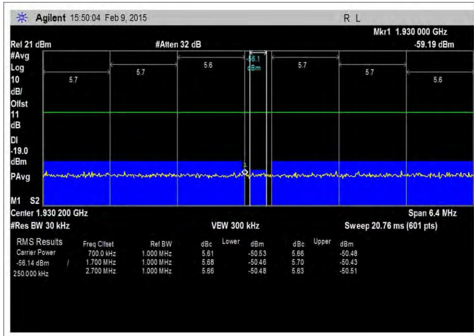
7.5_OBE_DL_1930-1995MHz_GSM_L_-20dBm
