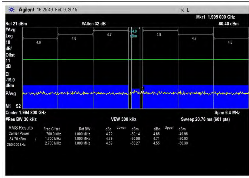
7.5_OBE_DL_1930-1995MHz_GSM_H_-20dBm
