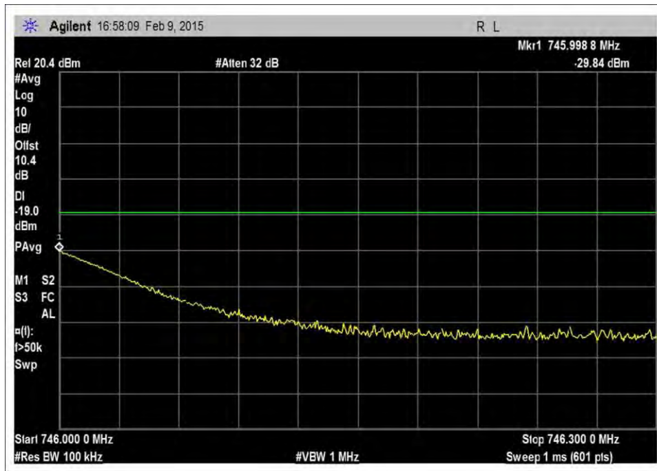
7.5_OBE_DL_728-746MHz_GSM_H_-48dBm
