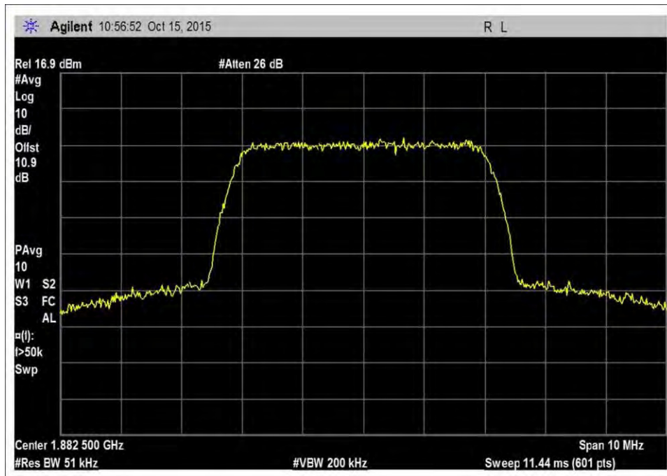
7.10_OBW_UL_1850-1915MHz_WCDMA
