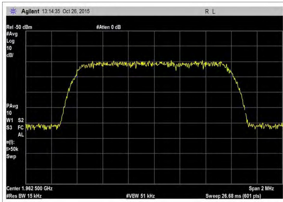
7.10_OBW_DL_1930-1995MHz_CDMA
