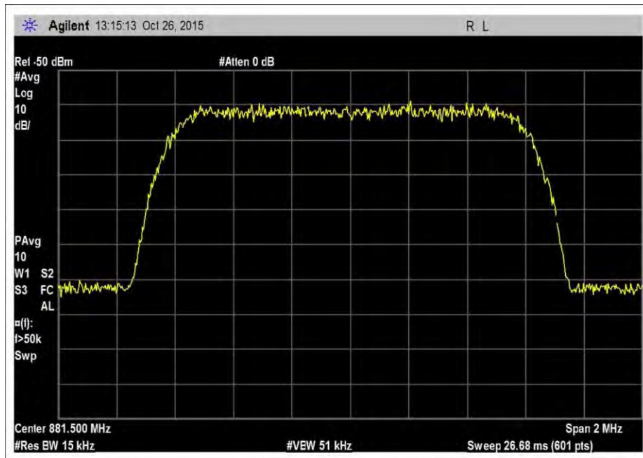
7.10_OBW_DL_869-894MHz_CDMA
