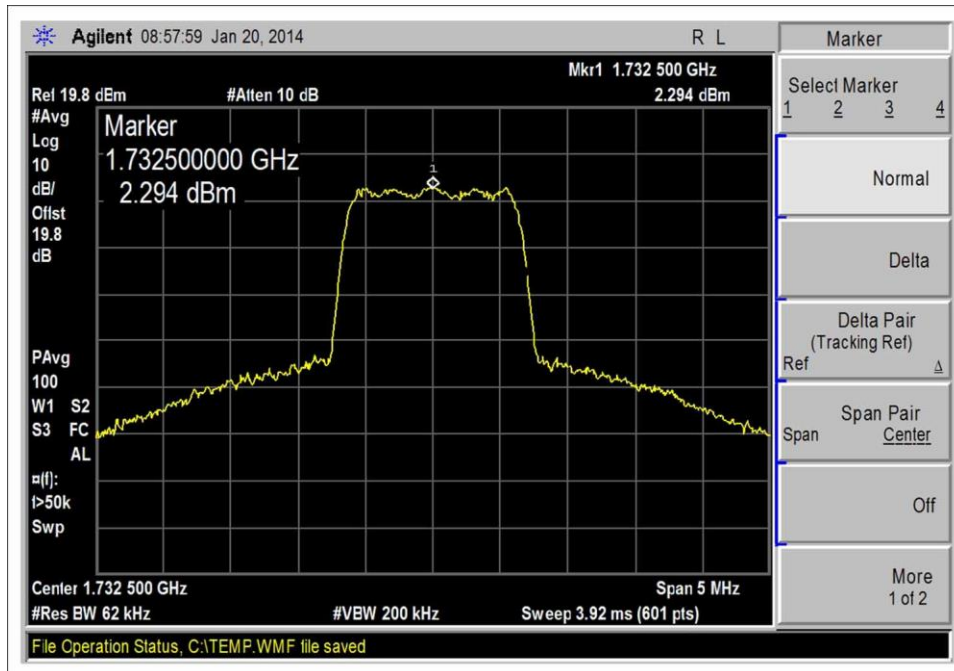
1710-1755MHz UL, CDMA-Output
