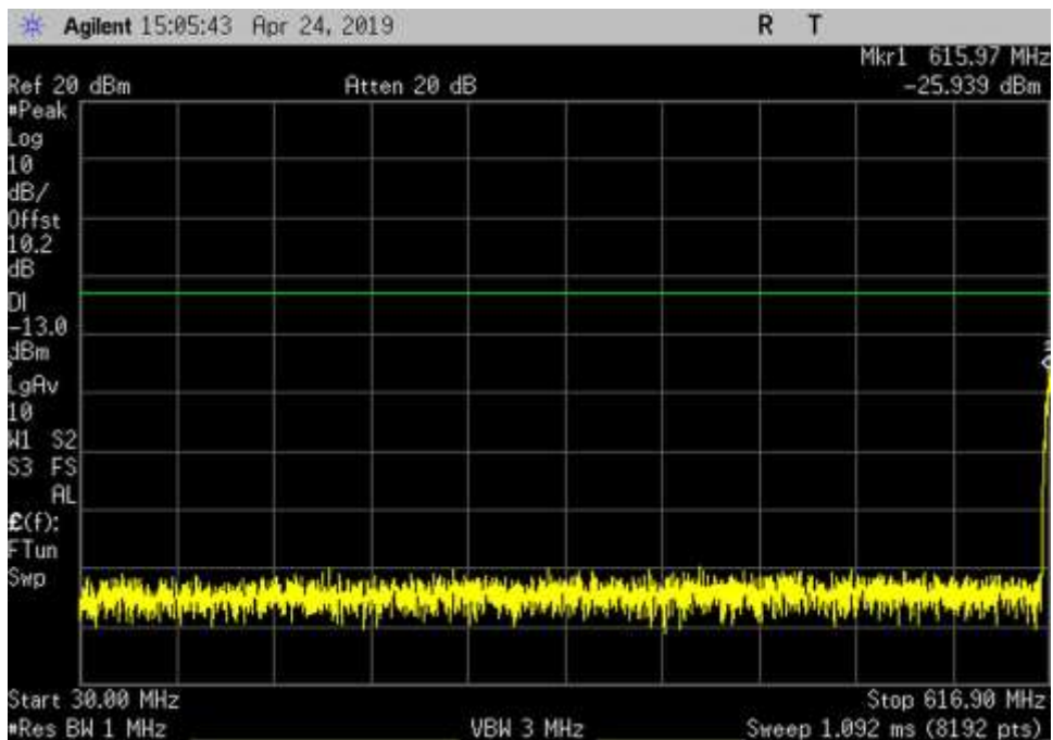
DL_617-652_GSM_30- 616.9MHz_HC
