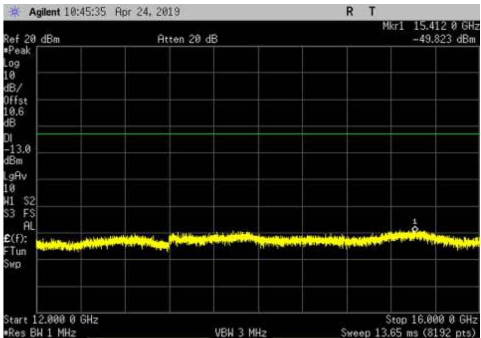
UL_1850-1915_GSM_12000-16000MHz_MC
