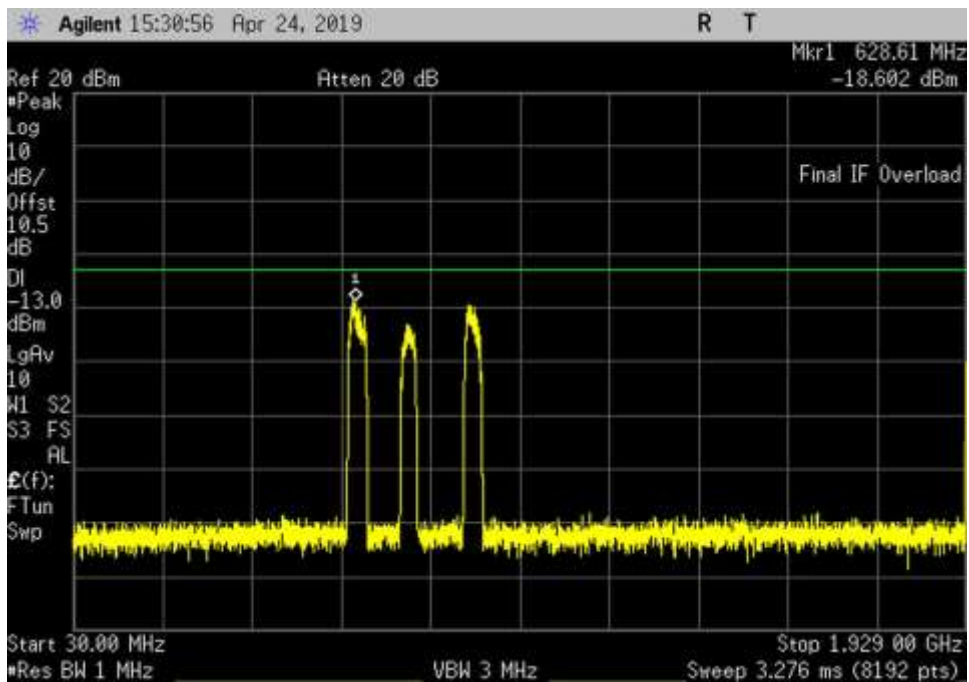
DL_1930-1995_AWGN_30-1929MHz_LC
