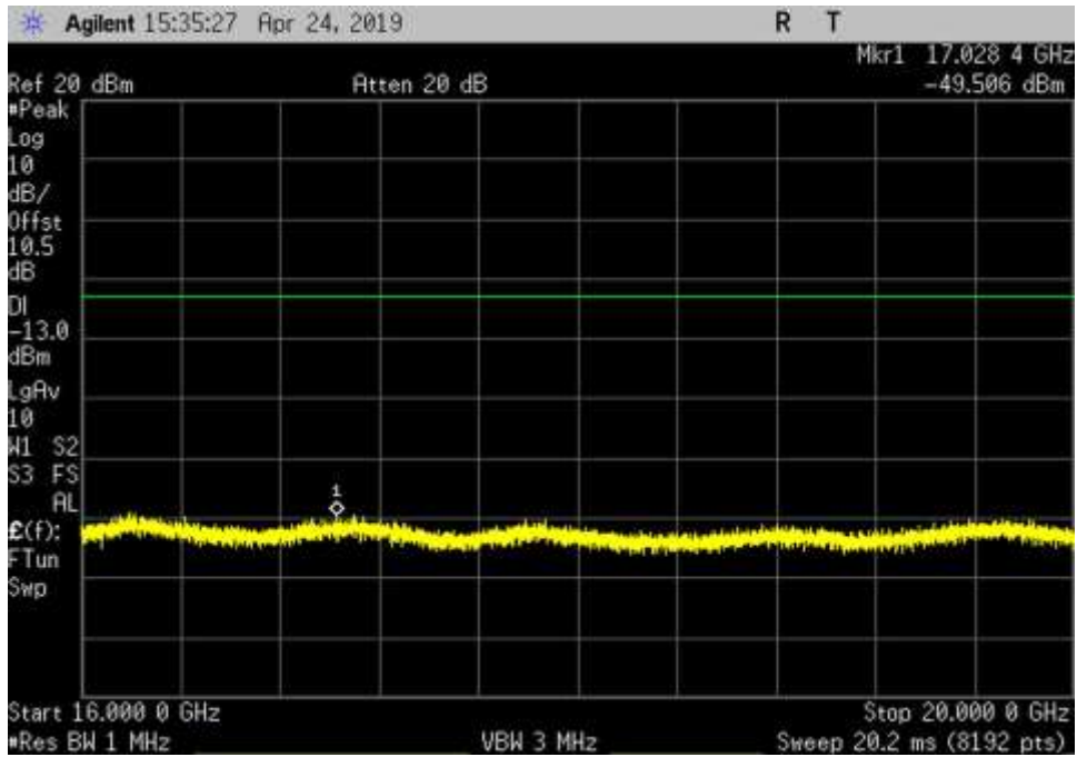
DL_1930-1995_AWGN_16000-20000MHz_HC
