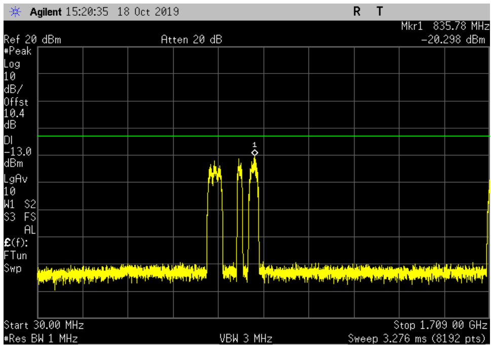
UL_1710-1755_GSM_30-1709MHz_MC
