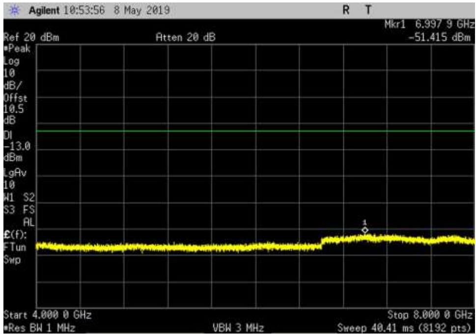
UL_2305-2315_GSM_4000-8000MHz_HC
