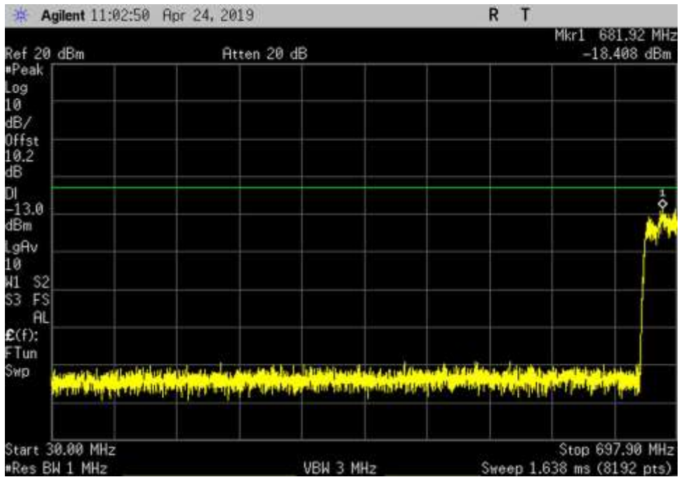
UL_698-716_GSM_30- 697.9MHz_MC
