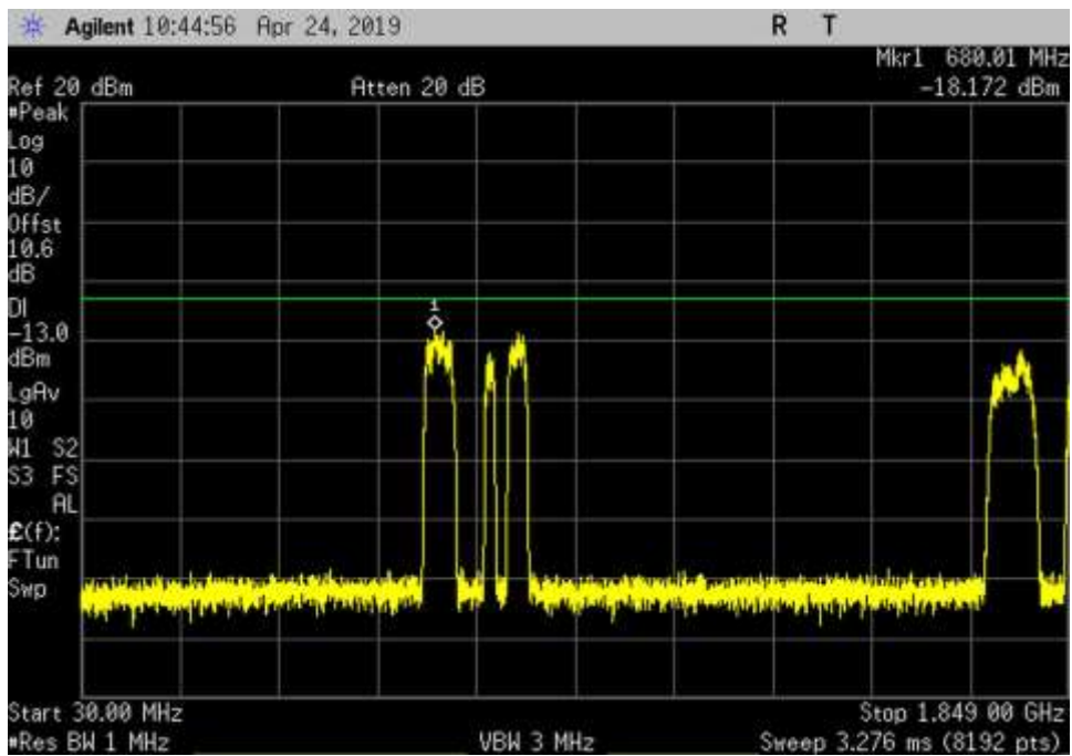
UL_1850-1915_GSM_30-1849MHz_MC
