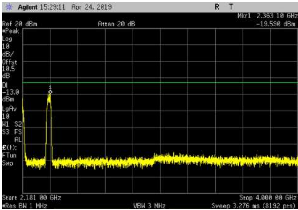
CSE_DL_2110-2155_AWGN_2181-4000MHz_HC
