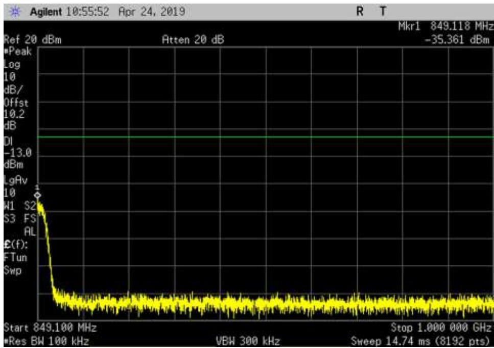
UL_824-849_GSM_849.1- 1000MHz_HC
