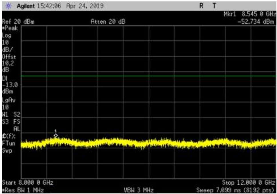
DL_869-894_AWGN_8000-12000MHz_HC
