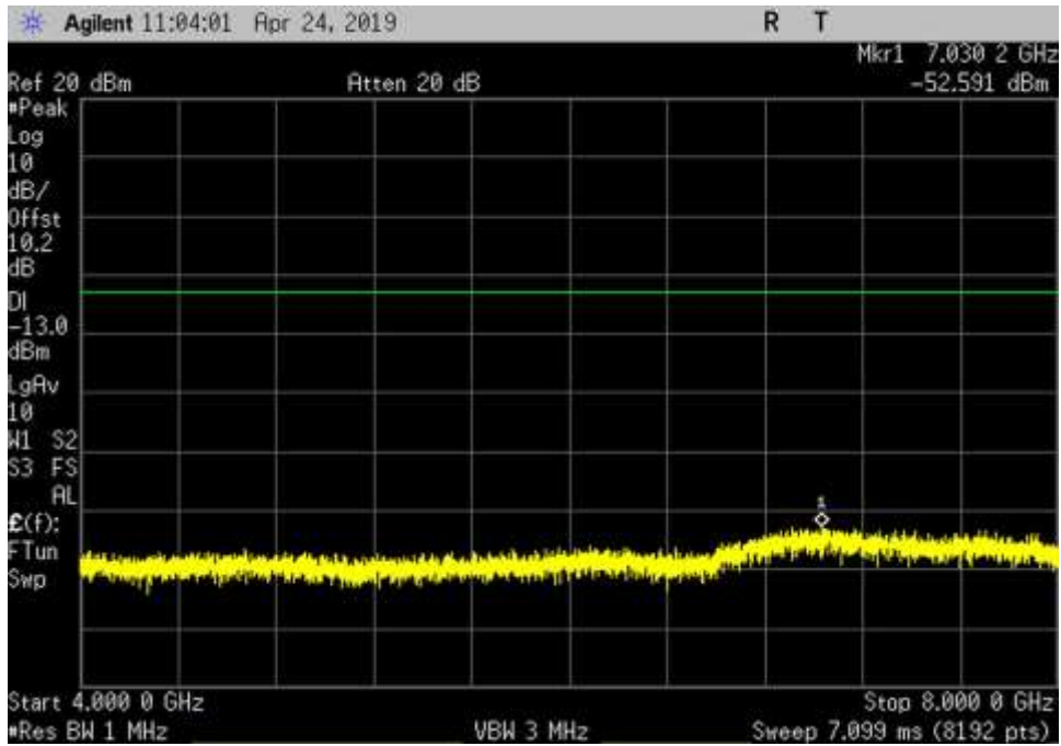
UL_698-716_GSM_4000-8000MHz_MC
