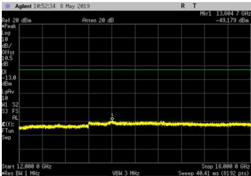
UL_2305-2315_GSM_12000-16000MHz_MC
